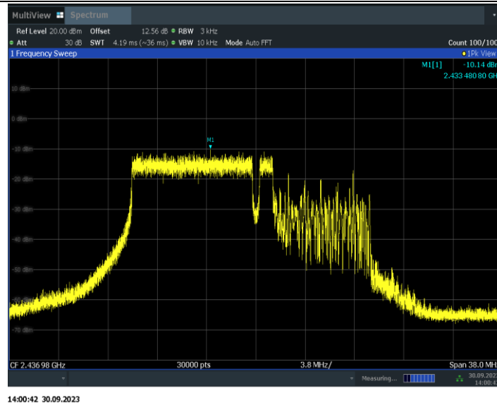
11BE20MIMO_Ant12_2437_106+26_OFDMA_2
