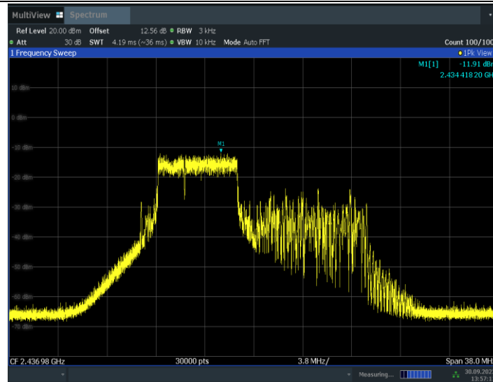
11BE20MIMO_Ant12_2437_52+26_OFDMA_3
