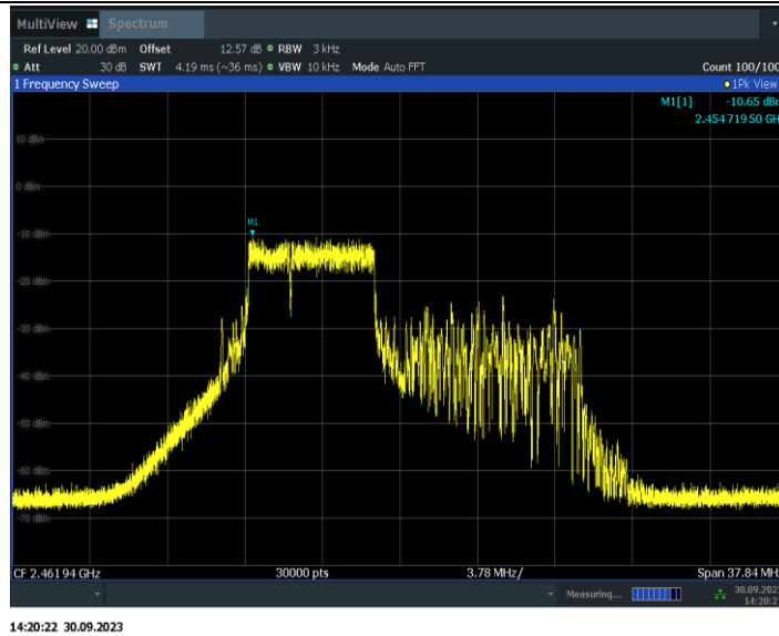
11BE20MIMO_Ant7_2462_52+26_OFDMA_3
