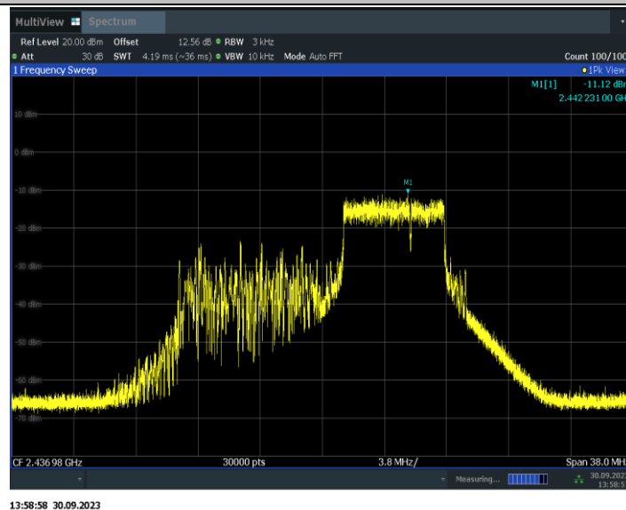
11BE20MIMO_Ant12_2437_106+26_OFDMA_1
