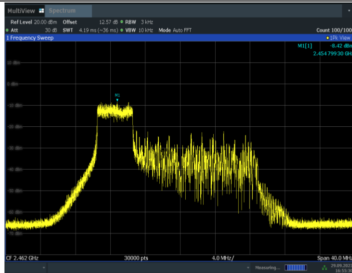
11AX20MIMO_Ant7_2462_52Tone_RU40
