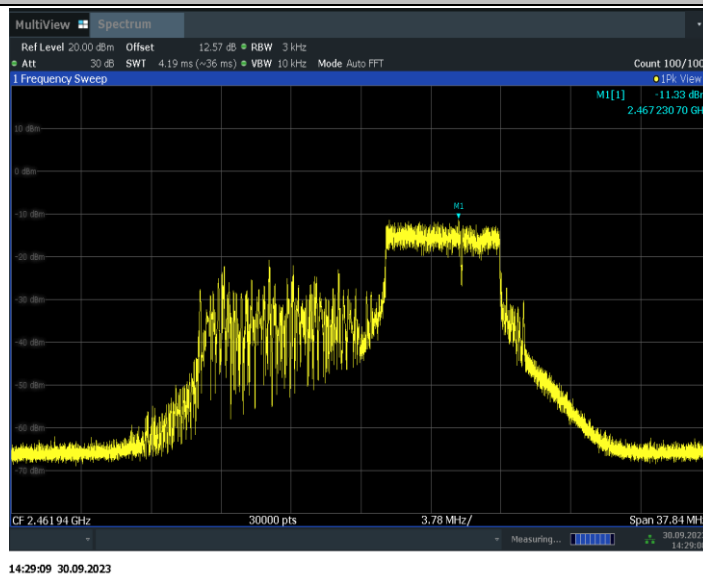
11BE20MIMO_Ant7_2462_106+26_OFDMA_1
