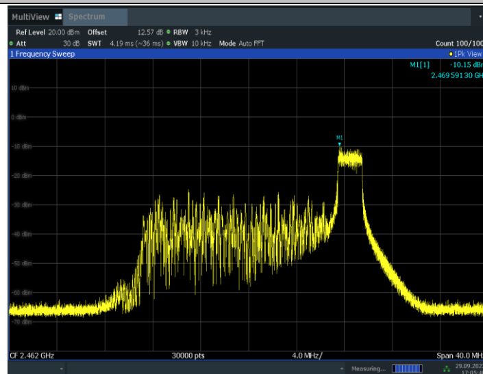
11AX20MIMO_Ant7_2462_26Tone_RU8
