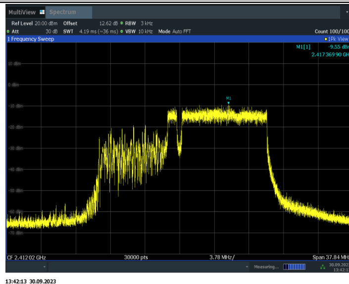
11BE20MIMO_Ant7_2412_52+26_OFDMA_1
