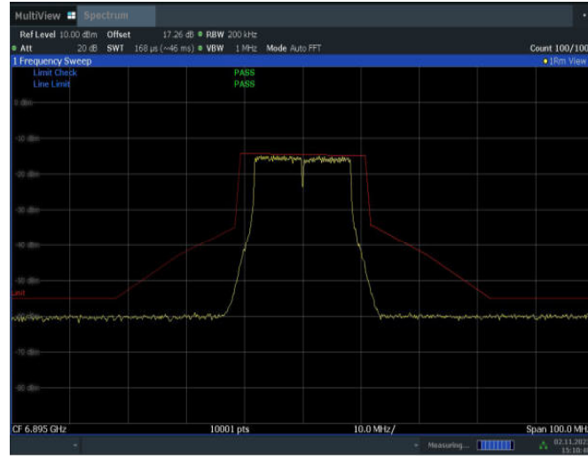
11A-MIMO_Ant15_6895
