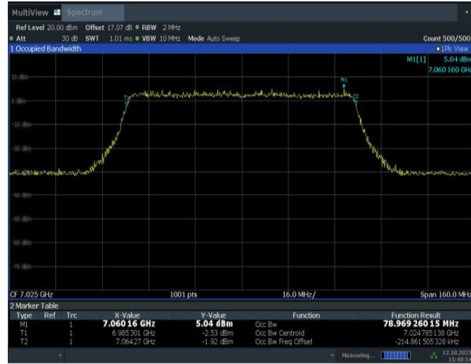
11BE80MIMO_Ant15_7025
