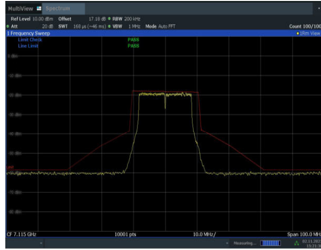
11A-MIMO_Ant15_7115
