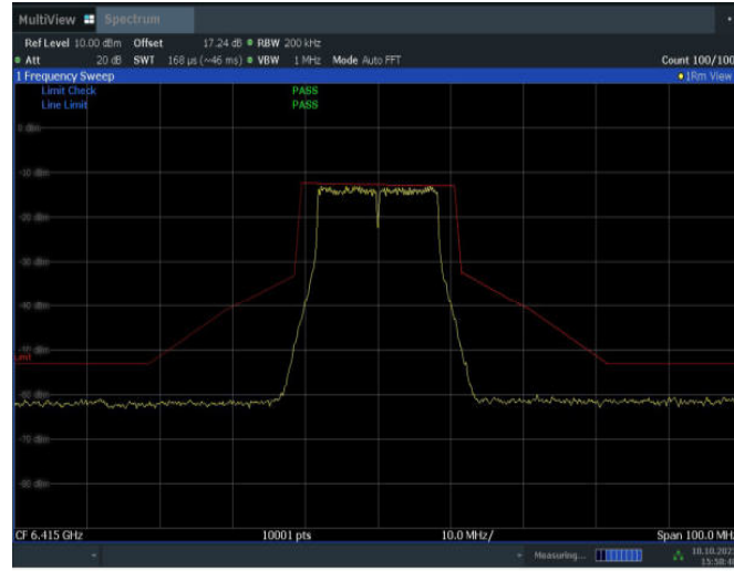
11A-MIMO_Ant15_6415
