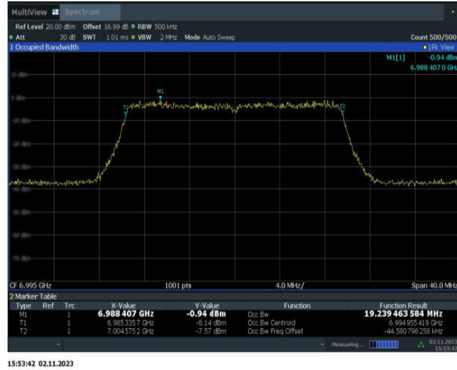
11BE20MIMO_Ant15_6995
