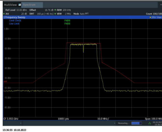
11A-MIMO_Ant15_5955
