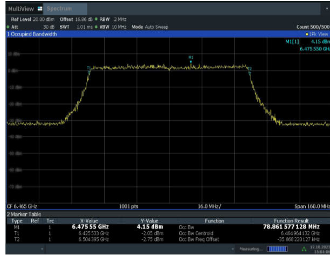
11BE80MIMO_Ant15_6465
