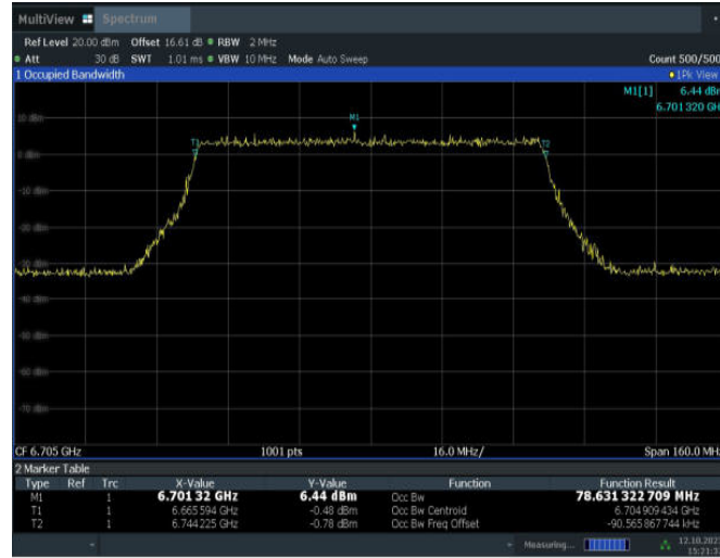
11BE80MIMO_Ant15_6705
