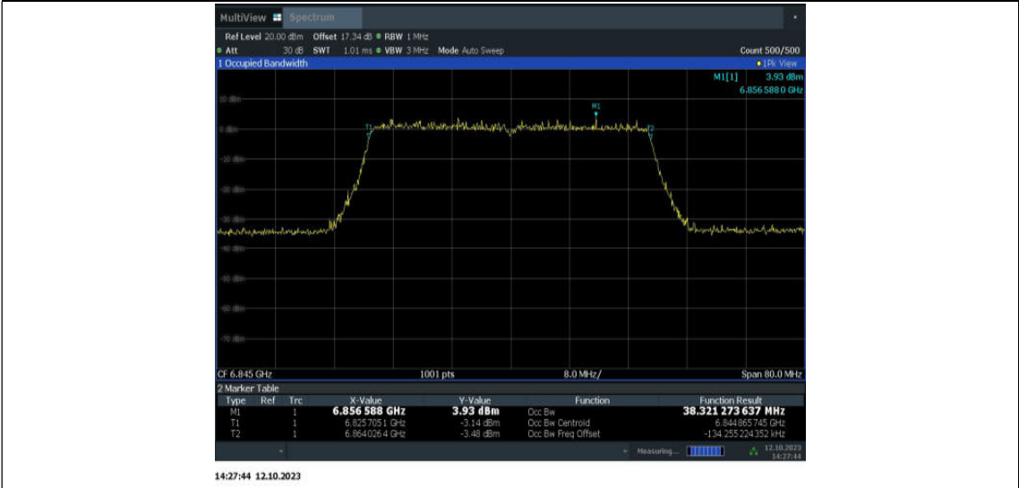
11BE40MIMO_Ant15_6845
