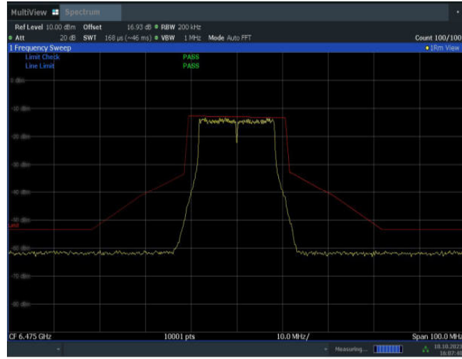
11A-MIMO_Ant15_6475
