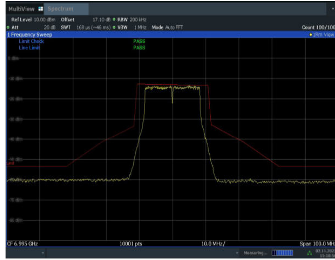
11A-MIMO_Ant15_6995
