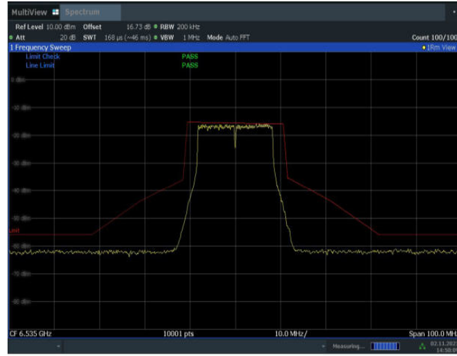
11A-MIMO_Ant15_6535
