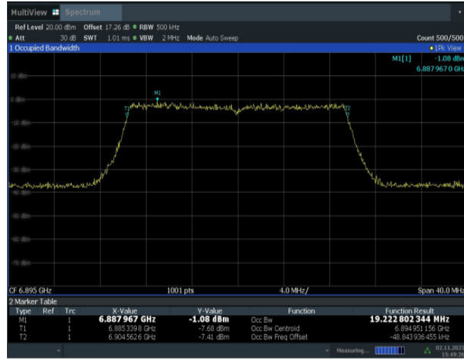
11BE20MIMO_Ant15_6895
