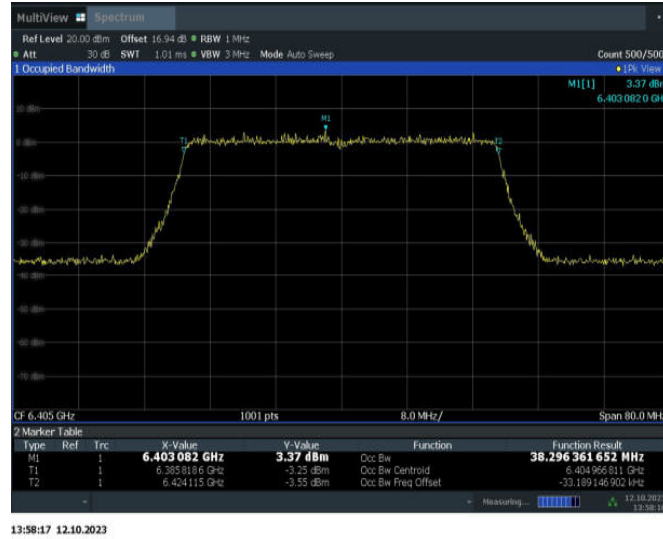
11BE40MIMO_Ant15_6405
