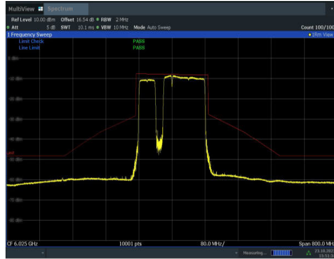
11BE160MIMO_Ant9_6025_996+484+242_OFDMA_4
