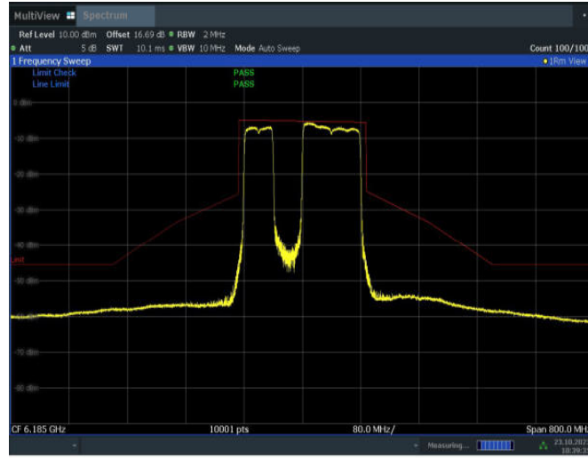
11BE160MIMO_Ant15_6185_996+484_OFDMA_2
