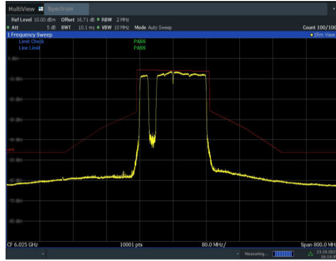
11BE160MIMO_Ant15_6025_996+484+242_OFDMA_2
