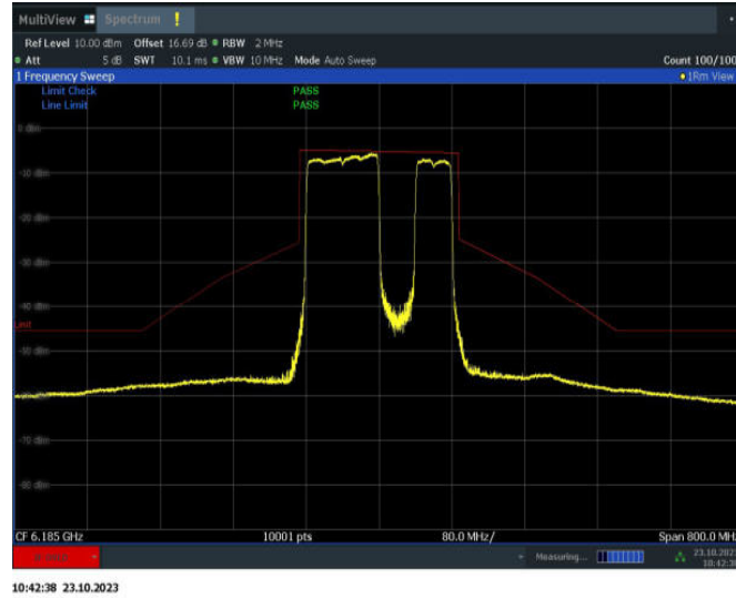
11BE160MIMO_Ant15_6185_996+484_OFDMA_4
