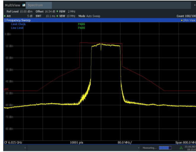
11BE160MIMO_Ant9_6025_996+484_OFDMA_2
