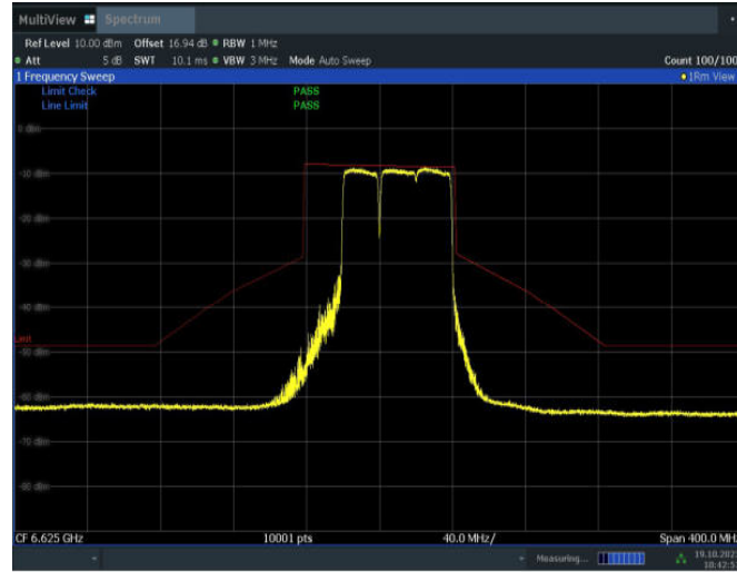
11BE80MIMO_Ant15_6625_484+242_OFDMA_2
