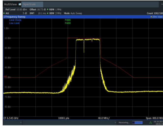
11BE80MIMO_Ant9_6545_484+242_OFDMA_2
