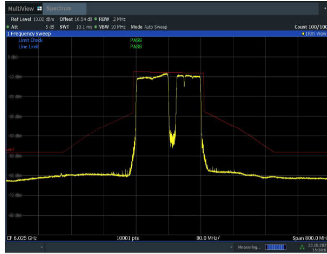
11BE160MIMO_Ant9_6025_996+484+242_OFDMA_6
