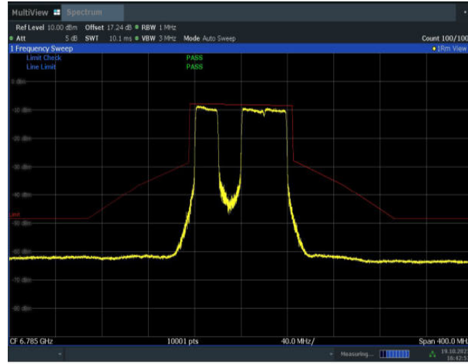
11BE80MIMO_Ant15_6785_484+242_OFDMA_2
