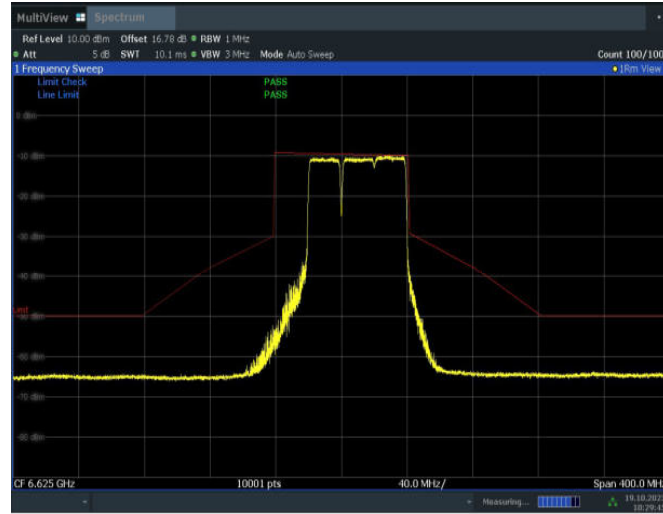
11BE80MIMO_Ant9_6625_484+242_OFDMA_2
