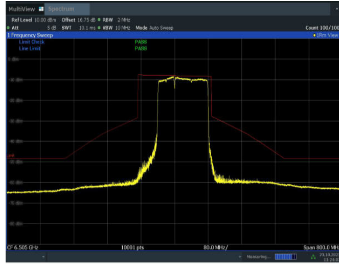
11BE160MIMO_Ant9_6505_996+484_OFDMA_2
