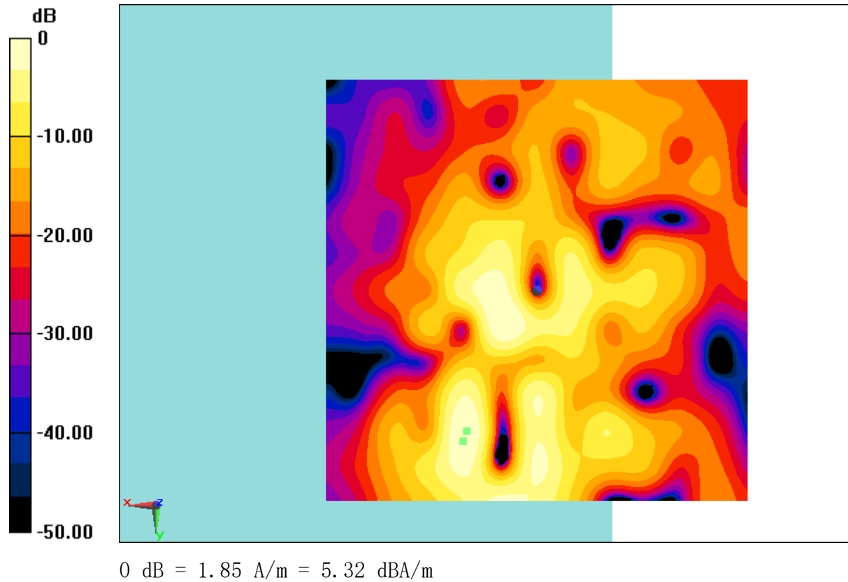
Fig B.43 T-Coil EDGE 1900
