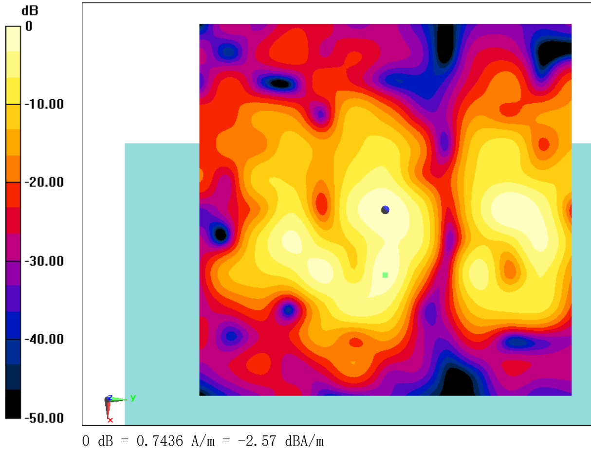
Fig B.39 T-Coil WiFi-2. 4G
