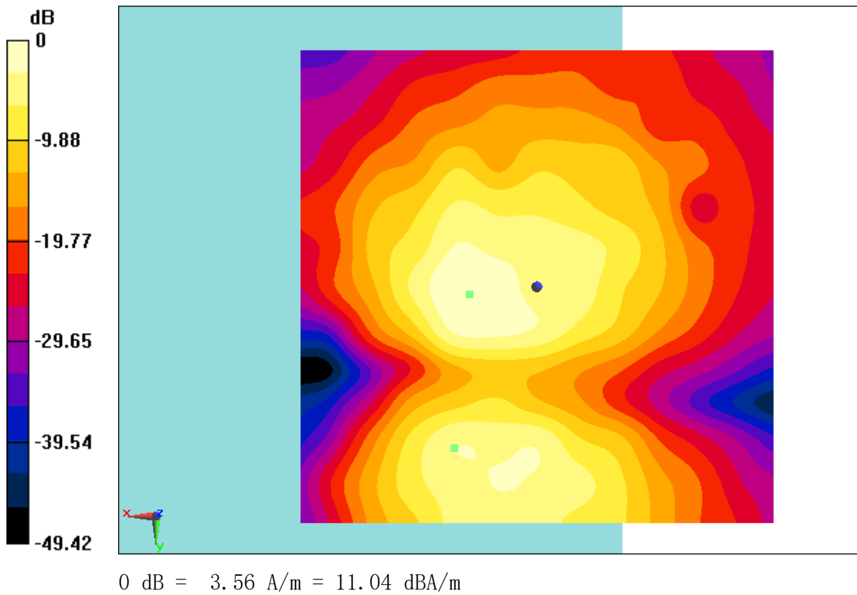
Fig B.45 T-Coil WCDMA 1900
