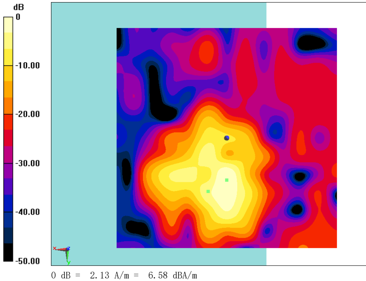
Fig B.44 T-Coil EDGE 1900
