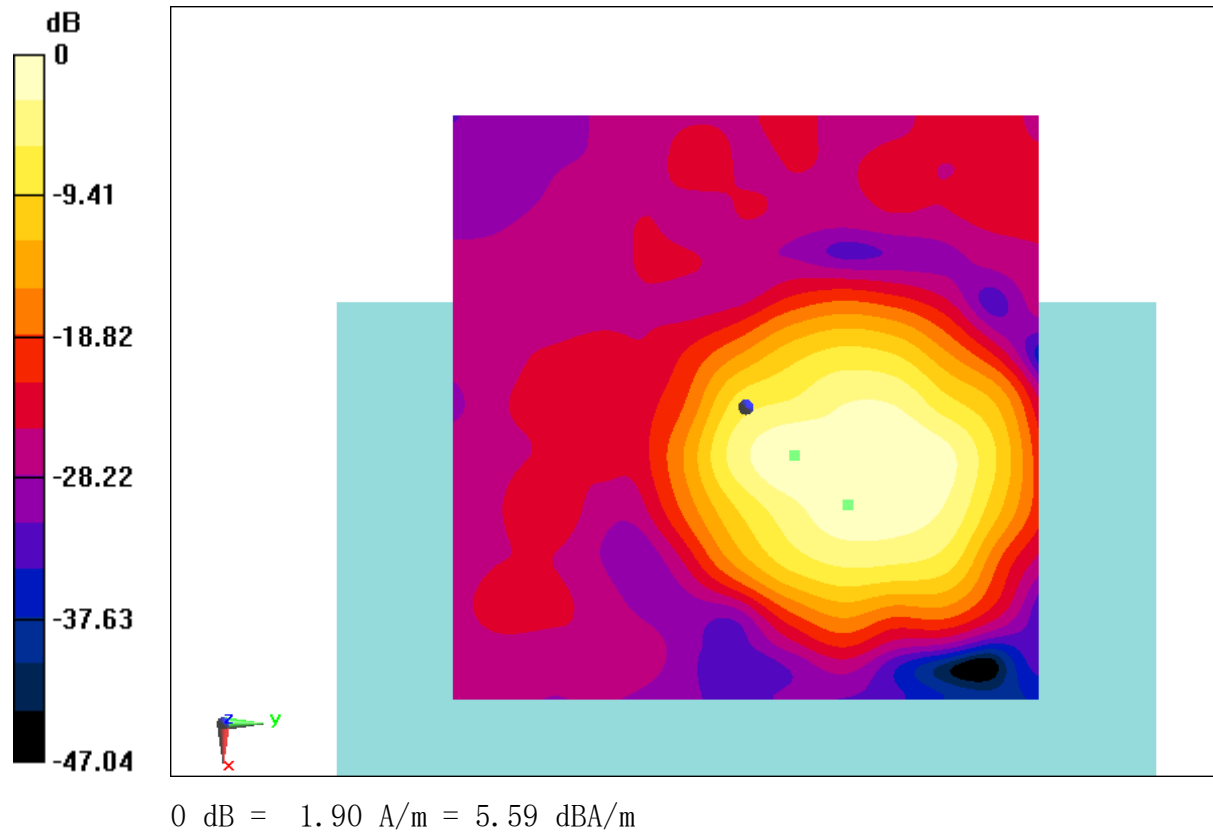
Fig B.46 T-Coil WCDMA 850
