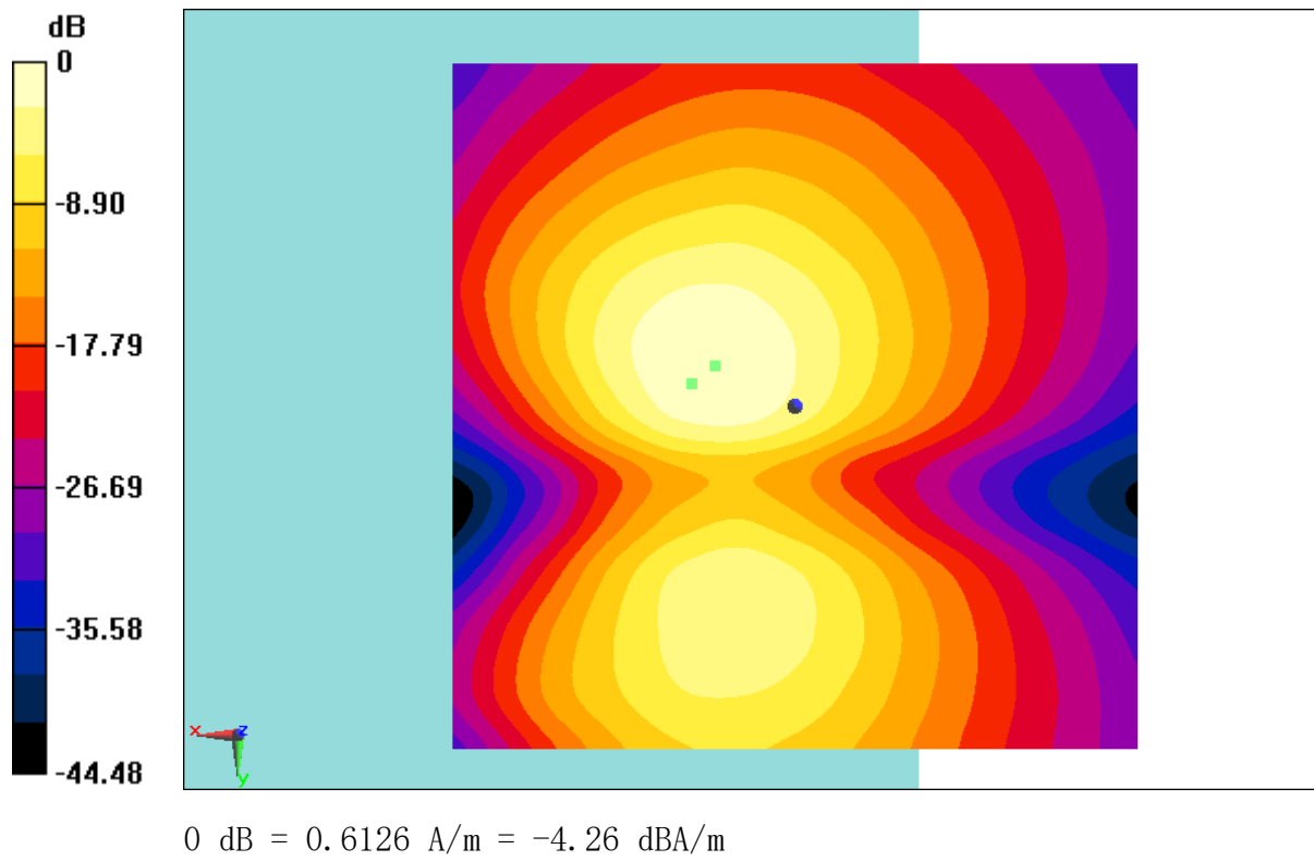
Fig B.9 T-Coil WCDMA 1700
