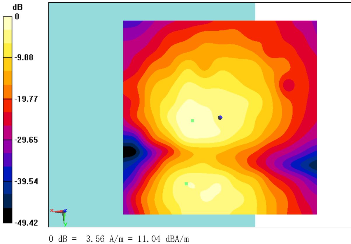
Fig B.41 T-Coil WCDMA 1900
