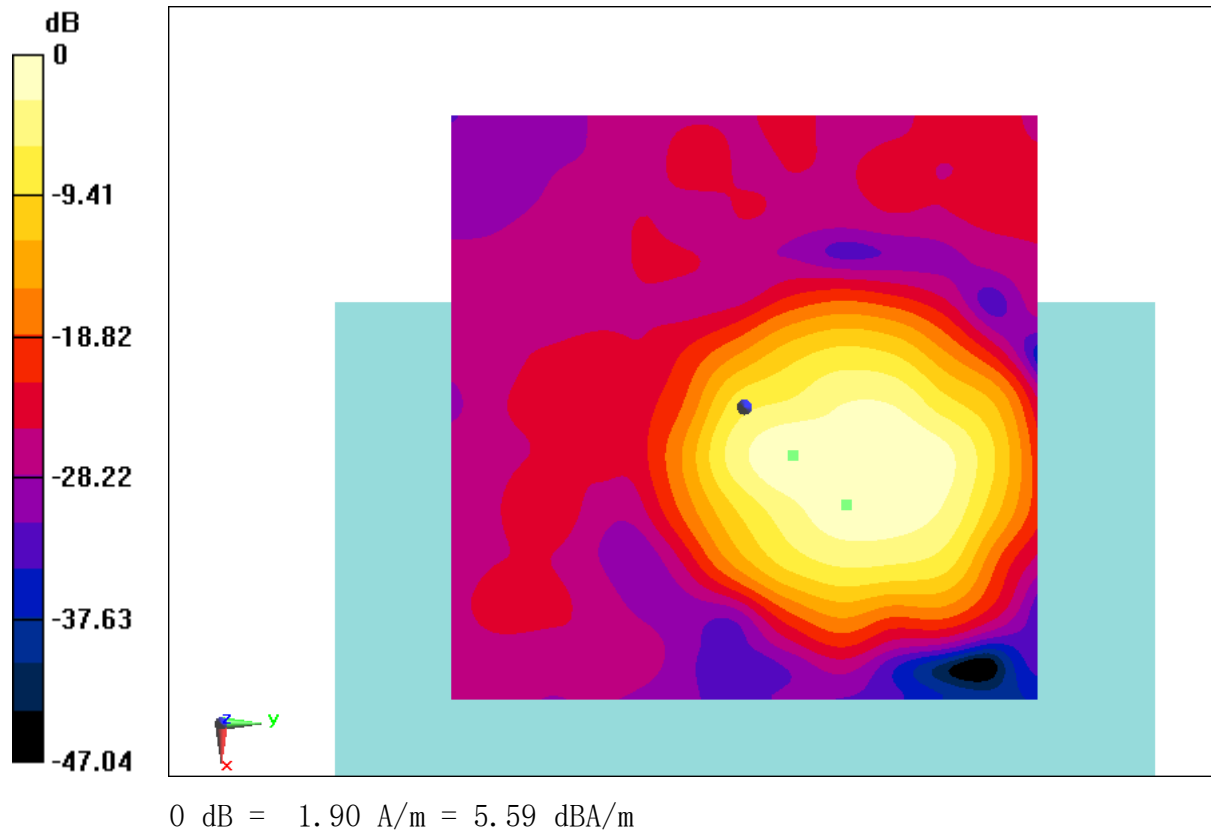
Fig B.42 T-Coil WCDMA 850
