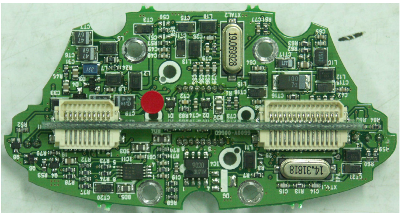
CCD Module
