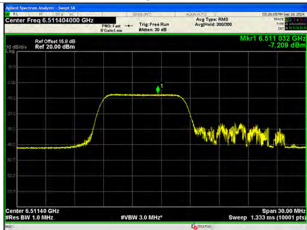
PSD NVNT ax20 106@53 6515MHz Ant13 MIMO
