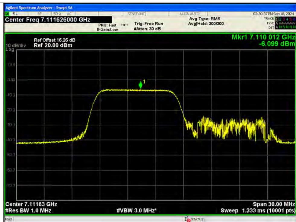
PSD NVNT ax20 106@53 7115MHz Ant13 MIMO
