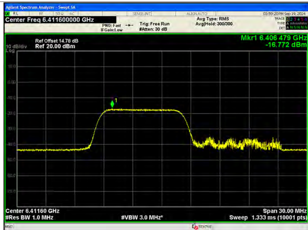
PSD NVNT ax20 106@53 6415MHz Ant13 MIMO
