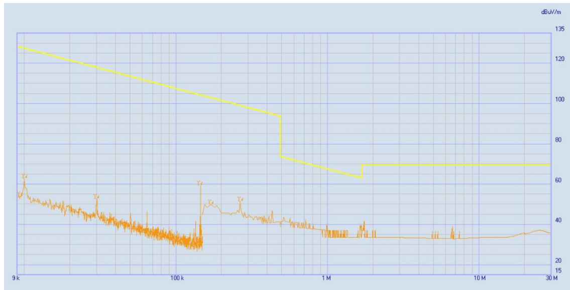
(Plot A: 9kHz to 30MHz, Close)
