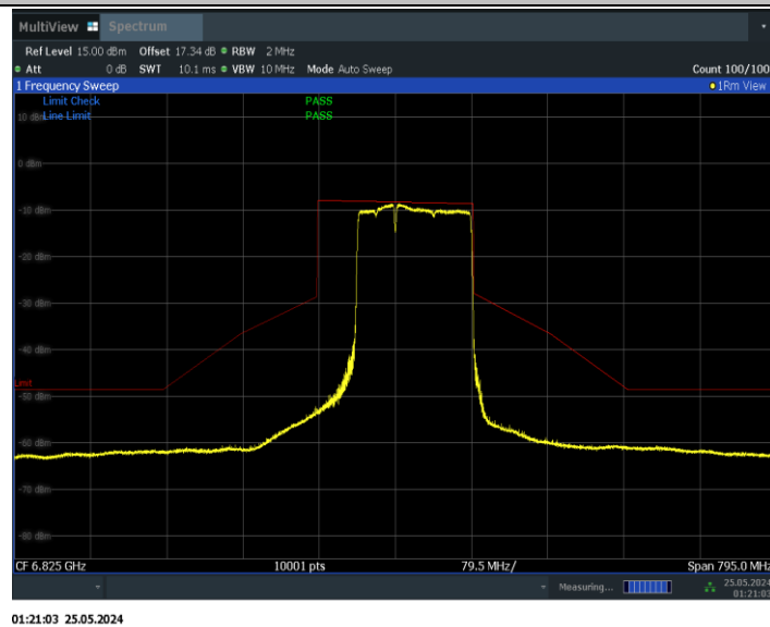
11BE160MIMO_Ant0_6825_996+484+242_Non-OFDMA_1
