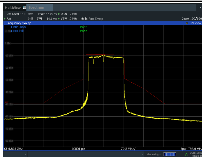
11BE160MIMO_Ant1_6825_996+484+242_Non-OFDMA_1
