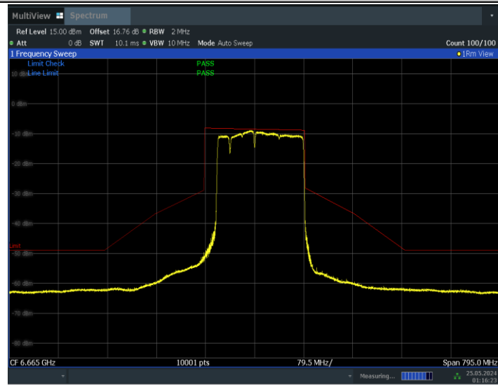
11BE160MIMO_Ant0_6665_996+484+242_Non-OFDMA_1
