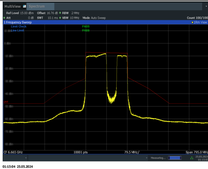
11BE160MIMO_Ant0_6665_996+484_Non-OFDMA_3
