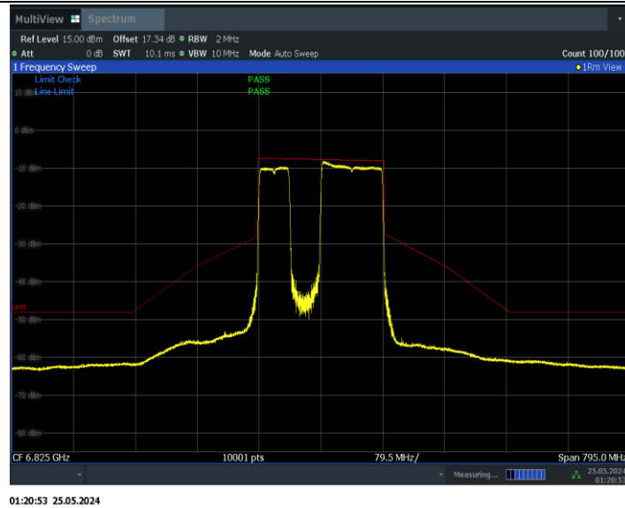
11BE160MIMO_Ant0_6825_996+484_Non-OFDMA_4
