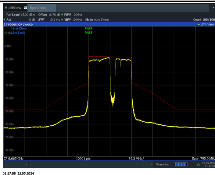
11BE160MIMO_Ant0_6665_996+484+242_Non-OFDMA_5
