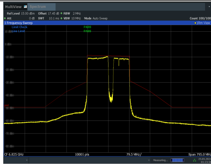
11BE160MIMO_Ant1_6825_996+484+242_Non-OFDMA_5
