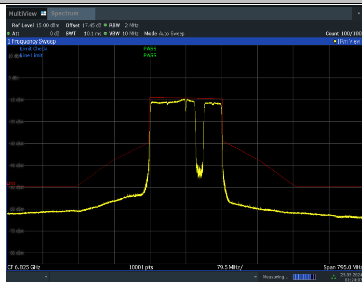
11BE160MIMO_Ant1_6825_996+484+242_Non-OFDMA_6
