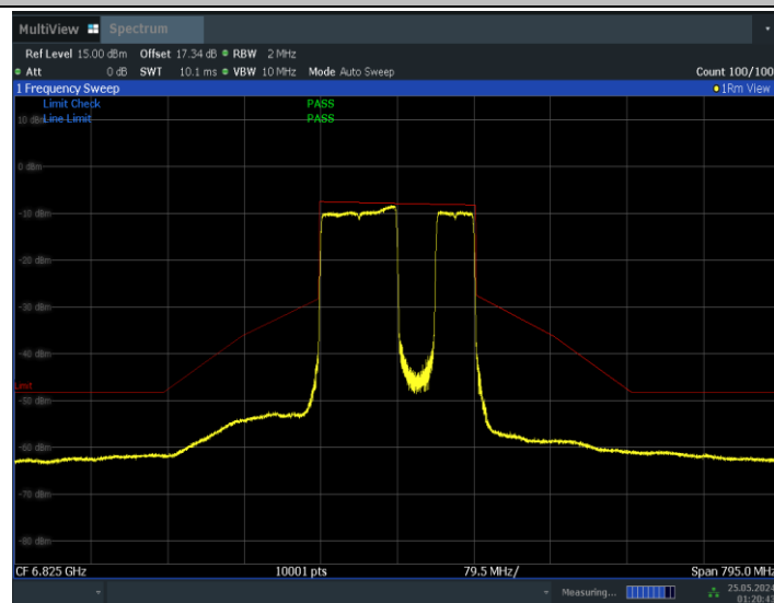
11BE160MIMO_Ant0_6825_996+484_Non-OFDMA_2
