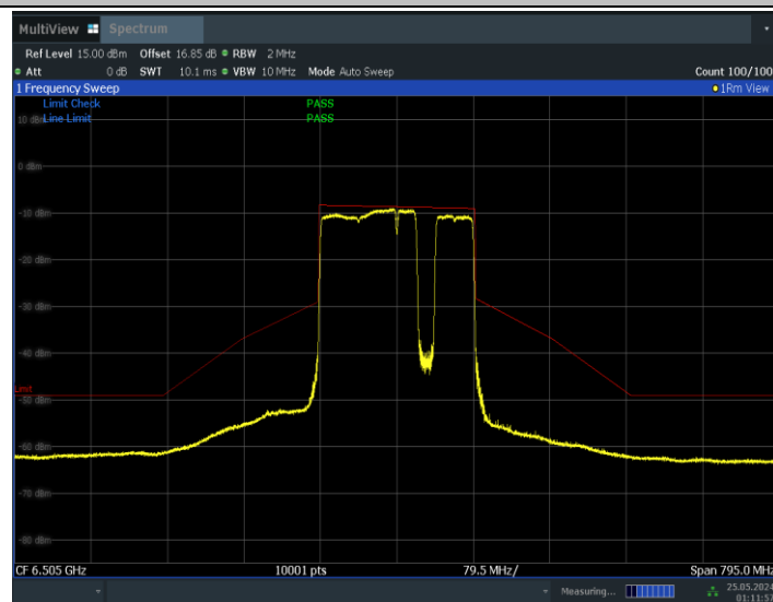
11BE160MIMO_Ant0_6505_996+484+242_Non-OFDMA_6
