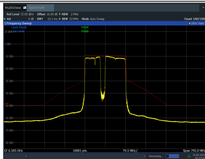
11BE160MIMO_Ant1_6505_996+484+242_Non-OFDMA_4
