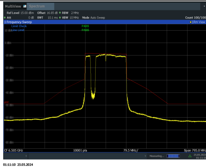
11BE160MIMO_Ant0_6505_996+484+242_Non-OFDMA_3
