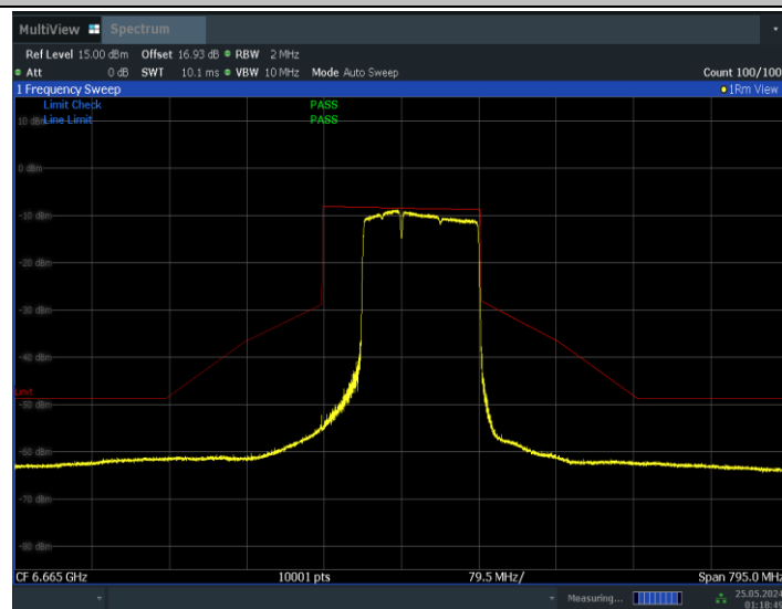
11BE160MIMO_Ant1_6665_996+484_Non-OFDMA_4
