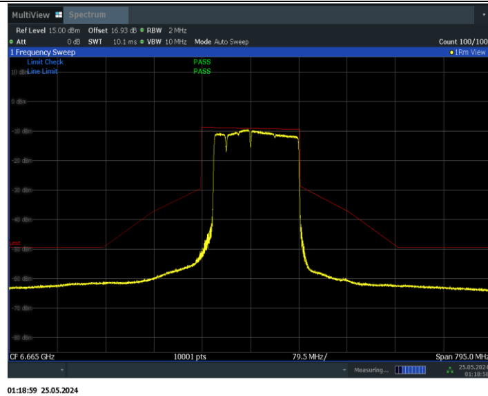
11BE160MIMO_Ant1_6665_996+484+242_Non-OFDMA_2
