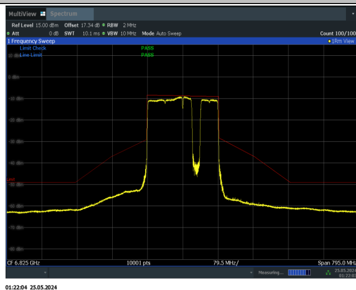
11BE160MIMO_Ant0_6825_996+484+242_Non-OFDMA_6
