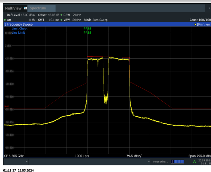
11BE160MIMO_Ant0_6505_996+484+242_Non-OFDMA_4
