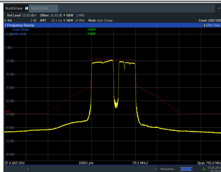
11BE160MIMO_Ant1_6665_996+484+242_Non-OFDMA_5
