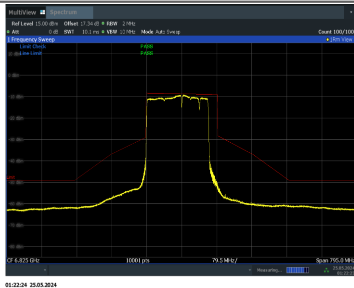
11BE160MIMO_Ant1_6825_996+484_Non-OFDMA_1
