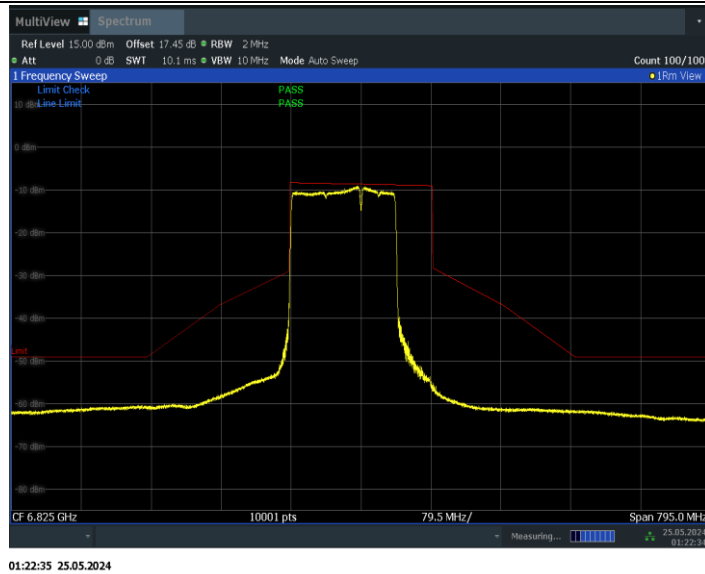
11BE160MIMO_Ant1_6825_996+484_Non-OFDMA_2
