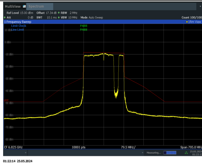
11BE160MIMO_Ant0_6825_996+484+242_Non-OFDMA_8
