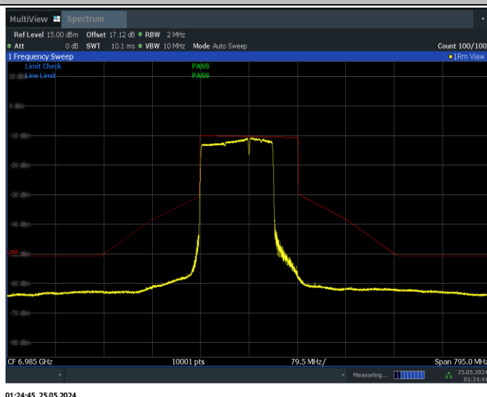
11BE160MIMO_Ant0_6985_996+484_Non-OFDMA_1
