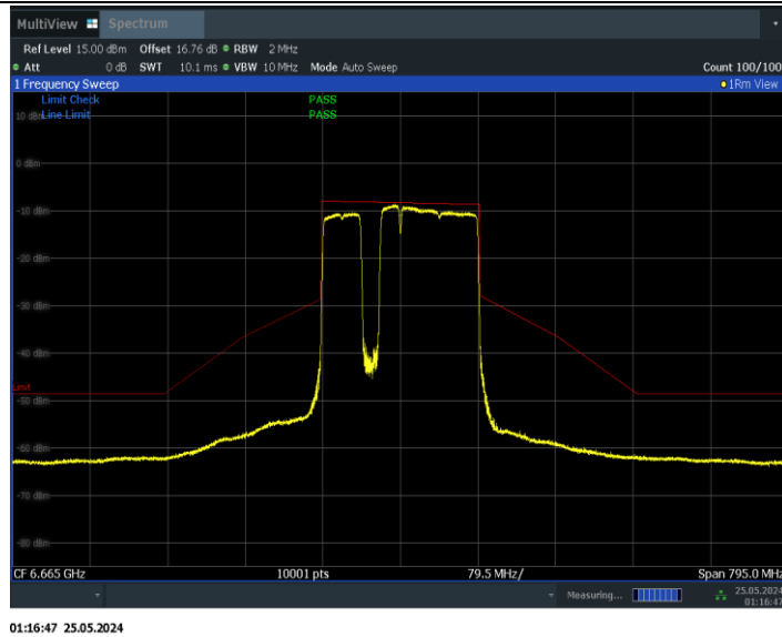
11BE160MIMO_Ant0_6665_996+484+242_Non-OFDMA_4
