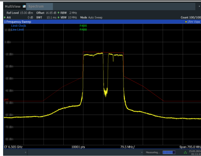
11BE160MIMO_Ant0_6505_996+484+242_Non-OFDMA_5
