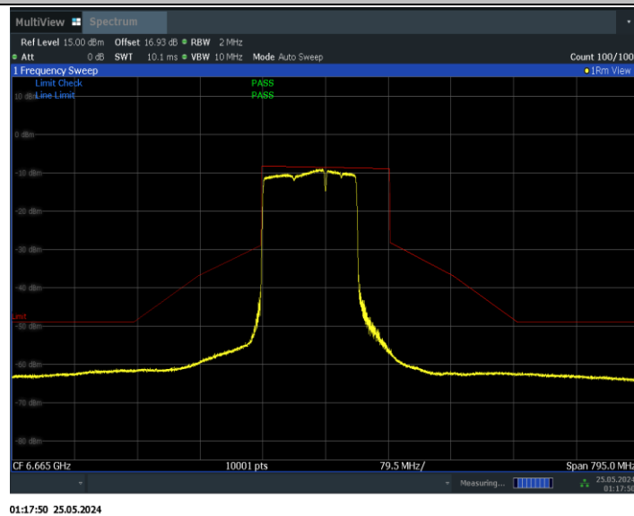
11BE160MIMO_Ant1_6665_996+484_Non-OFDMA_2
