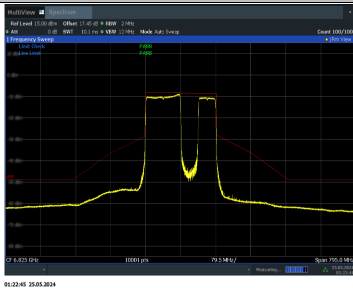
11BE160MIMO_Ant1_6825_996+484_Non-OFDMA_3
