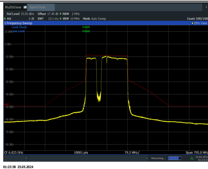
11BE160MIMO_Ant1_6825_996+484+242_Non-OFDMA_4
