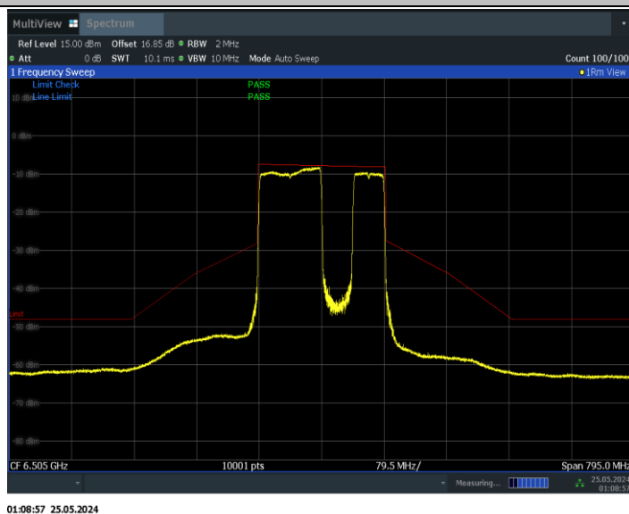
11BE160MIMO_Ant0_6505_996+484_Non-OFDMA_3
