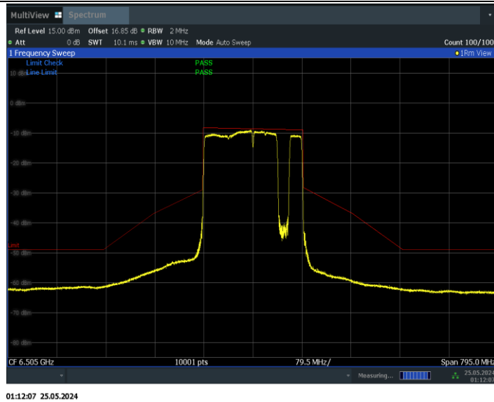
11BE160MIMO_Ant0_6505_996+484+242_Non-OFDMA_8
