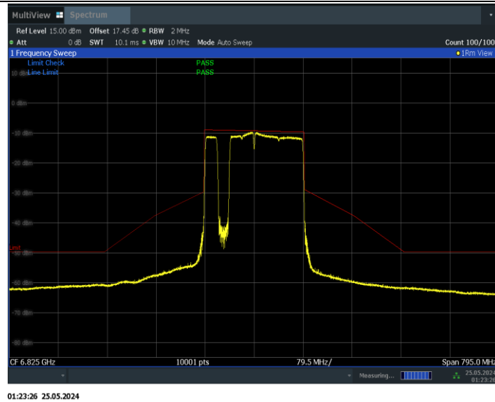
11BE160MIMO_Ant1_6825_996+484+242_Non-OFDMA_3
