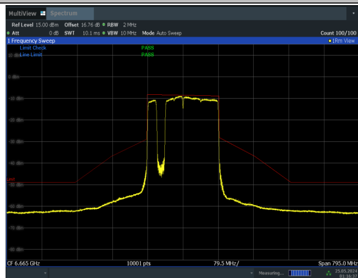
11BE160MIMO_Ant0_6665_996+484+242_Non-OFDMA_2
