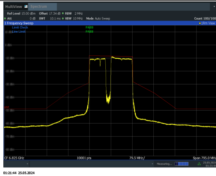
11BE160MIMO_Ant0_6825_996+484+242_Non-OFDMA_5
