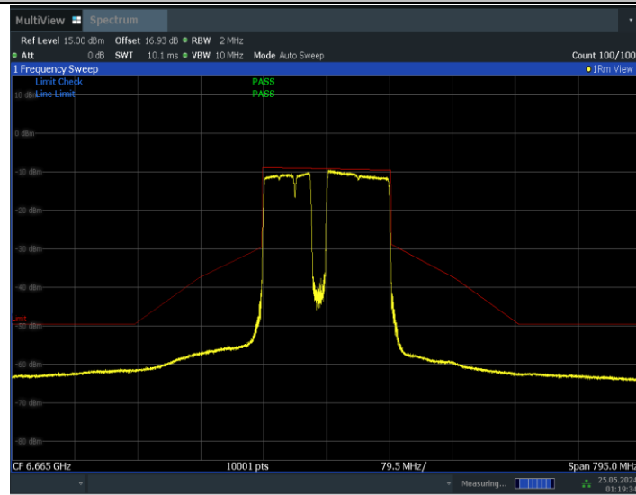
11BE160MIMO_Ant1_6665_996+484+242_Non-OFDMA_4
