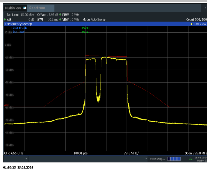
11BE160MIMO_Ant1_6665_996+484+242_Non-OFDMA_3
