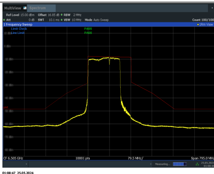
11BE160MIMO_Ant0_6505_996+484_Non-OFDMA_2
