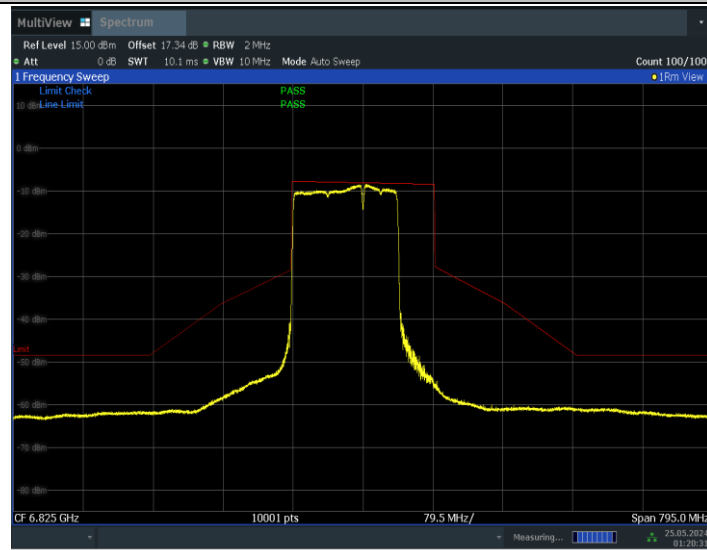
11BE160MIMO_Ant0_6825_996+484_Non-OFDMA_1
