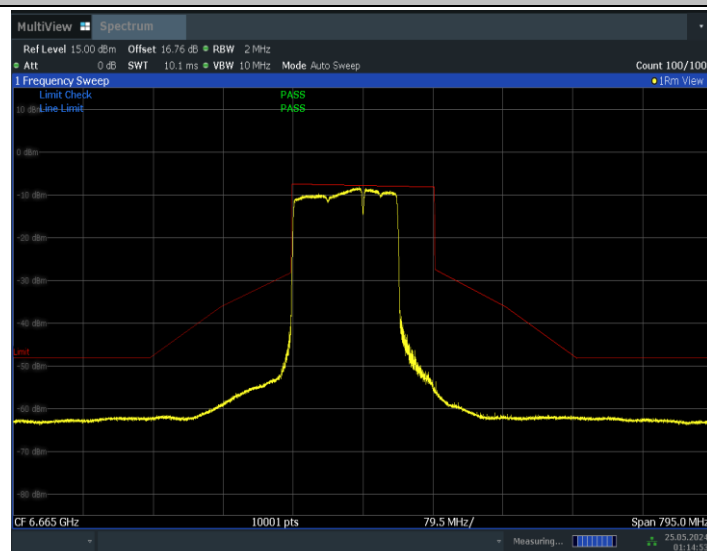
11BE160MIMO_Ant0_6665_996+484_Non-OFDMA_1
