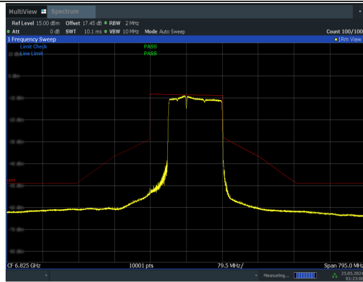
11BE160MIMO_Ant1_6825_996+484_Non-OFDMA_4
