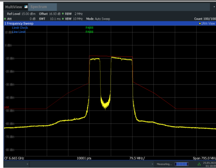
11BE160MIMO_Ant1_6665_996+484_Non-OFDMA_3
