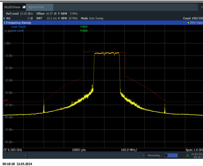
11BE320MIMO_Ant0_6585_3*996_Non-OFDMA_1
