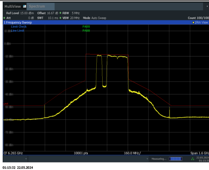
11BE320MIMO_Ant1_6265_2*996+484_Non-OFDMA_9
