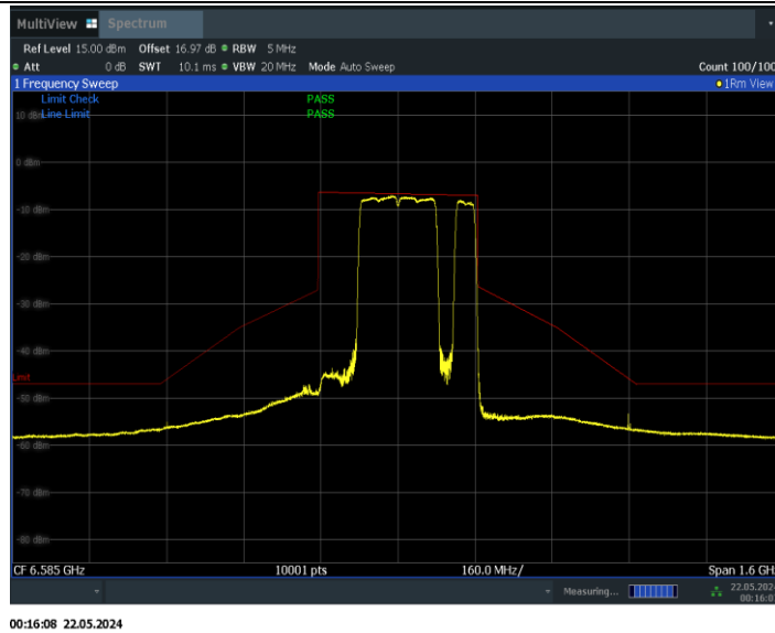
11BE320MIMO_Ant0_6585_2*996+484_Non-OFDMA_12
