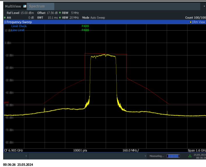
11BE320MIMO_Ant1_6905_2*996+484_Non-OFDMA_2
