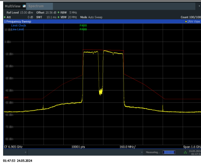
11BE320MIMO_Ant0_6905_3*996+484_Non-OFDMA_5
