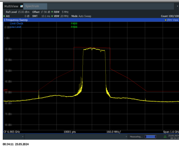
11BE320MIMO_Ant1_6905_3*996_Non-OFDMA_1
