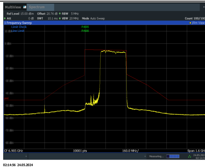
11BE320MIMO_Ant1_6905_2*996+484_Non-OFDMA_8
