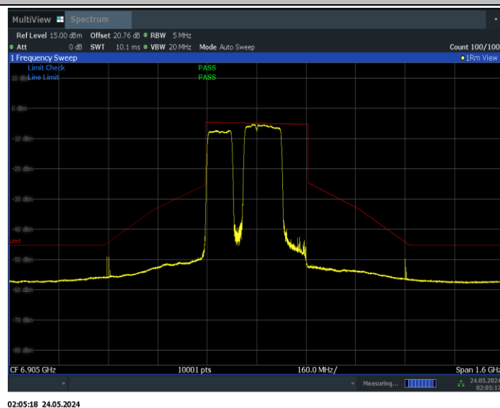
11BE320MIMO_Ant1_6905_2*996+484_Non-OFDMA_3
