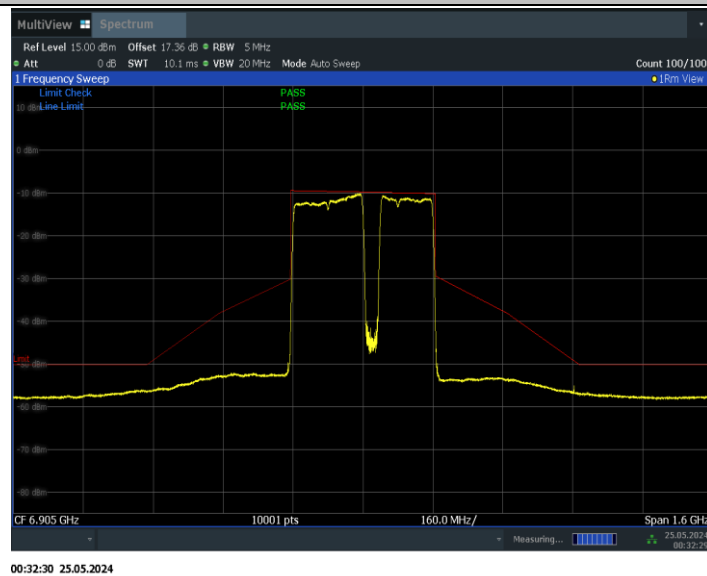
11BE320MIMO_Ant0_6905_3*996+484_Non-OFDMA_6
