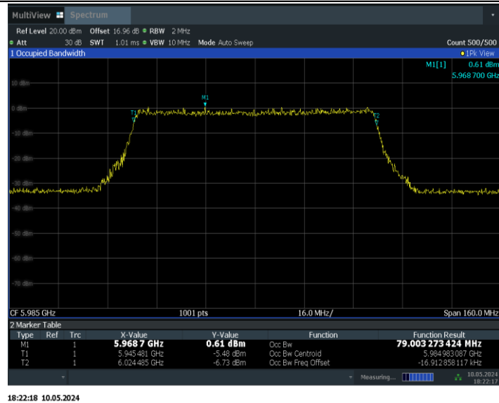
11BE80MIMO_Ant1_5985
