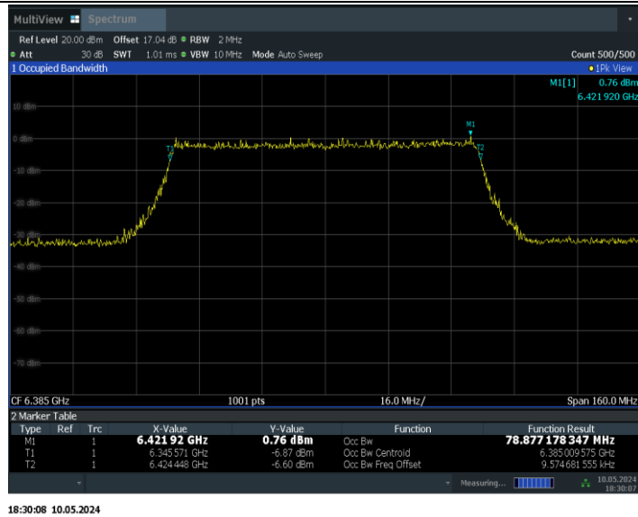
11BE80MIMO_Ant1_6385
