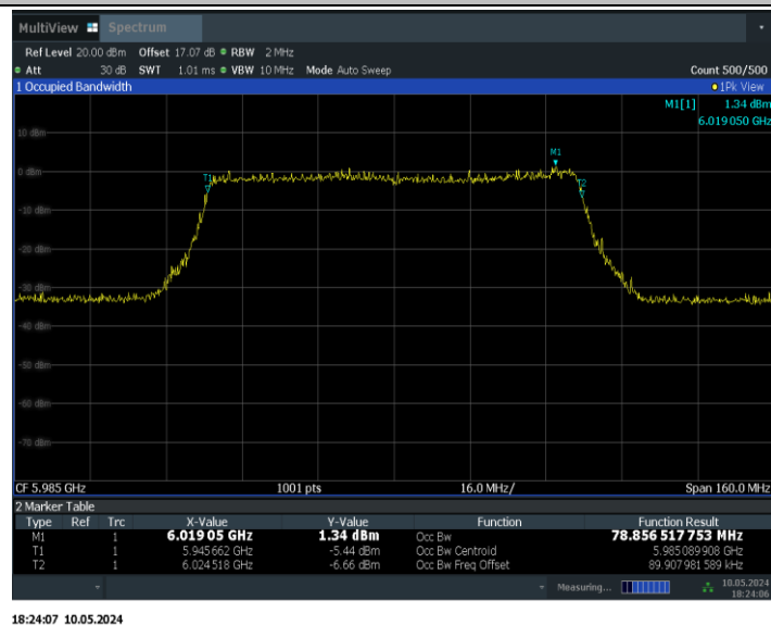
11BE80MIMO_Ant1_5985
