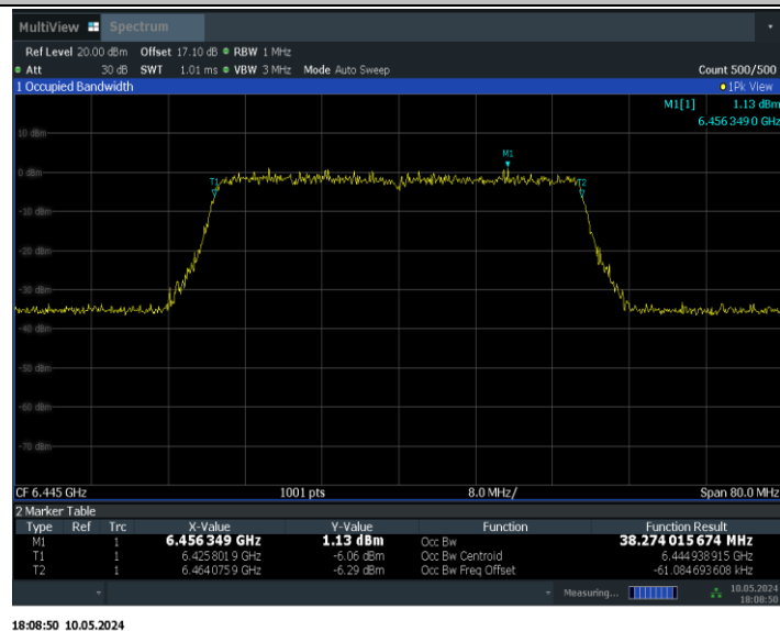
11BE40MIMO_Ant1_6445
