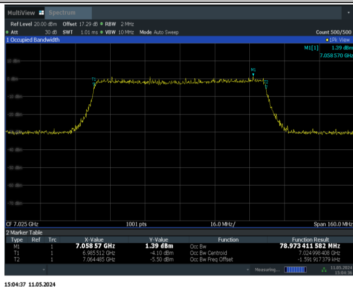
11BE80MIMO_Ant1_7025
