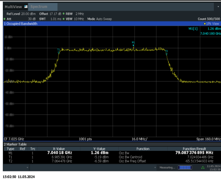
11BE80MIMO_Ant1_7025
