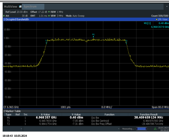
11BE40MIMO_Ant0_6965
