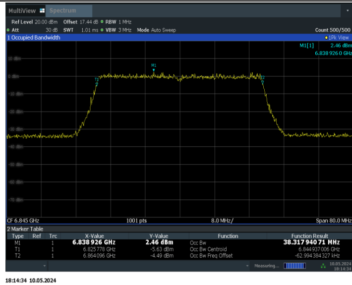
11BE40MIMO_Ant1_6845
