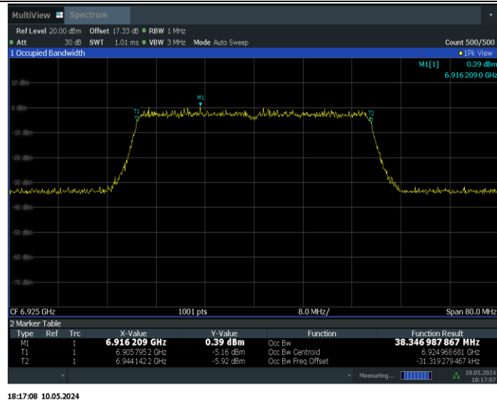
11BE40MIMO_Ant1_6925
