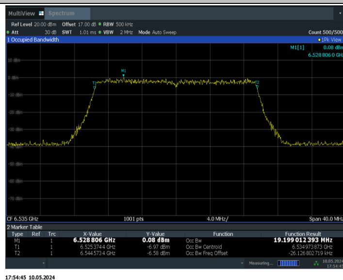
11BE20MIMO_Ant1_6535
