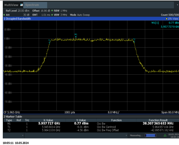
11BE40MIMO_Ant1_5965
