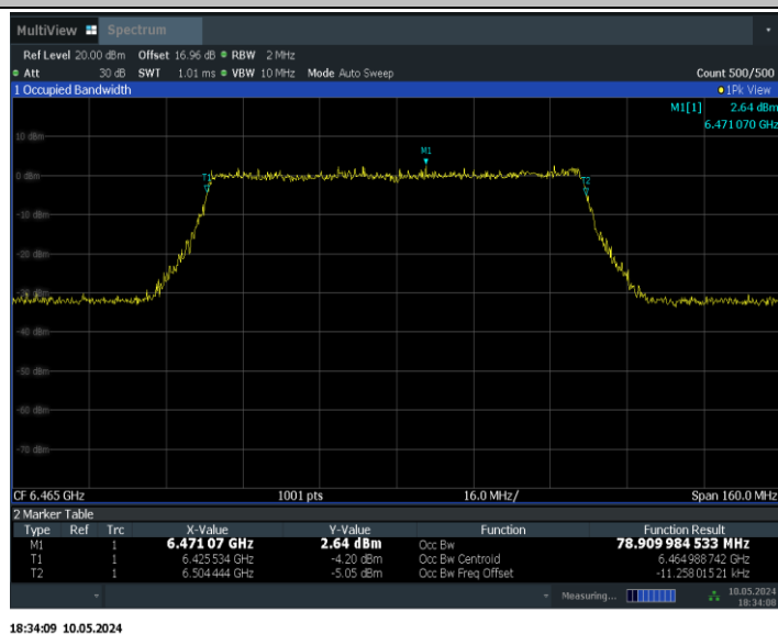
11BE80MIMO_Ant0_6465
