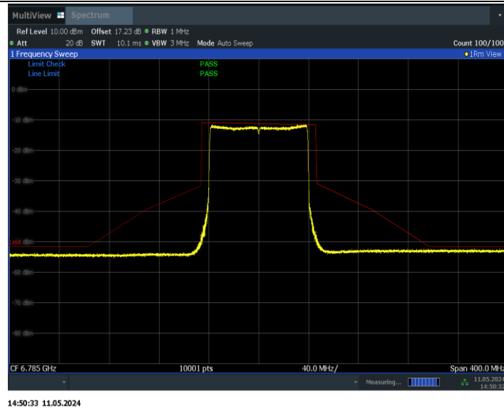
11BE80MIMO_Ant1_6785
