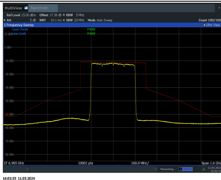
11BE320MIMO_Ant0_6905
