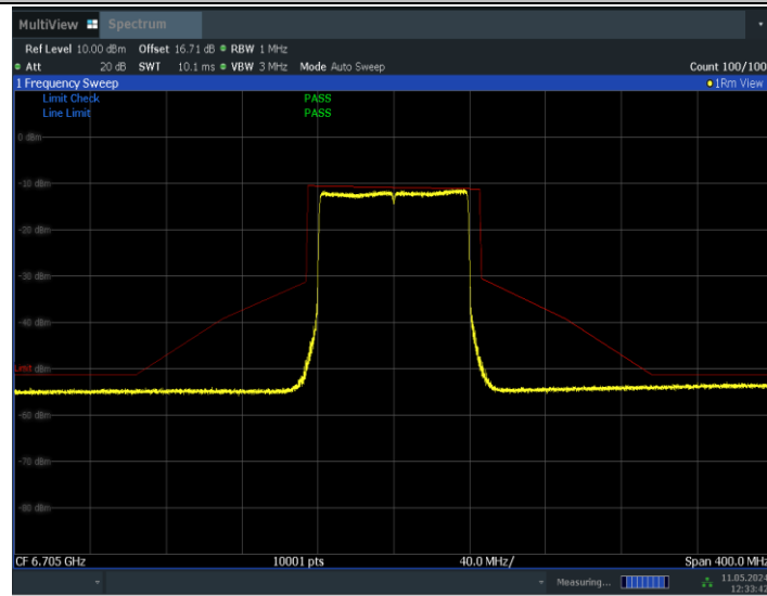
11BE80MIMO_Ant0_6705
