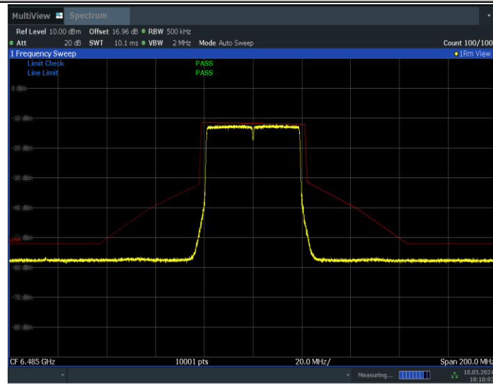
11BE40MIMO_Ant0_6485
