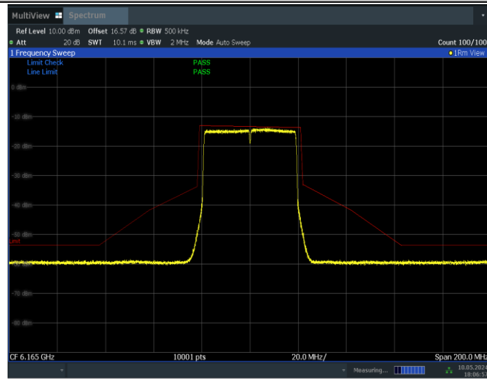
11BE40MIMO_Ant1_6165
