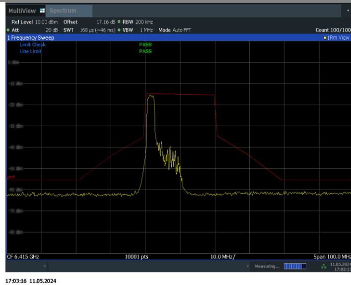
11BE20MIMO_Ant0_6415_52Tone_RU37
