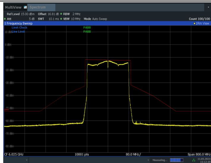
11BE160MIMO_Ant1_6025
