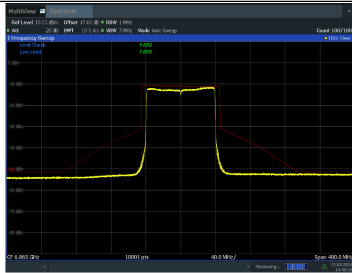
11BE80MIMO_Ant1_6865
