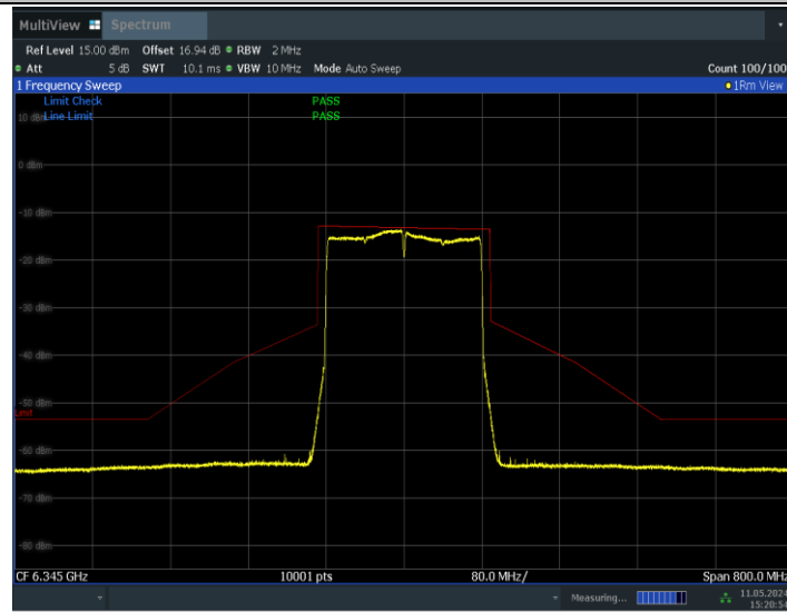
11BE160MIMO_Ant1_6345
