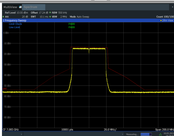
11BE40MIMO_Ant0_7085
