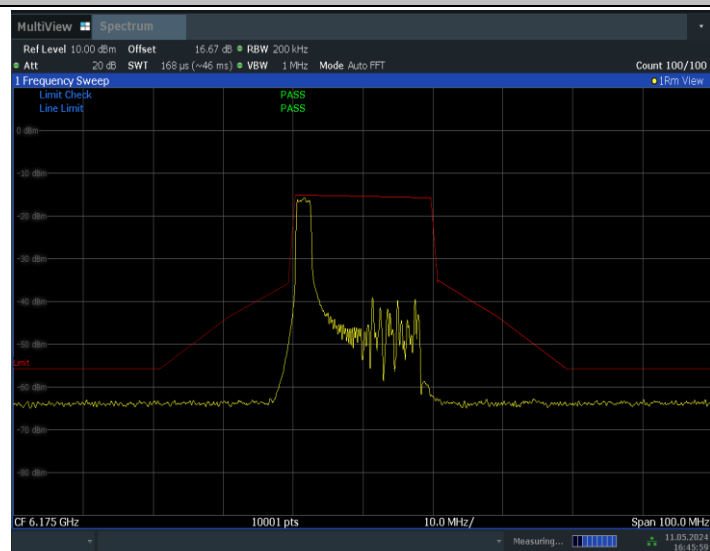
11BE20MIMO_Ant0_6175_26Tone_RU0
