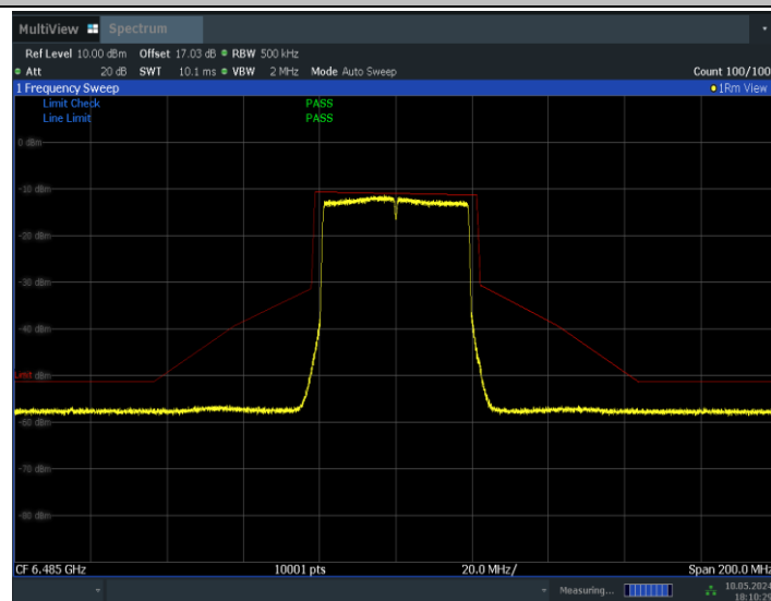
11BE40MIMO_Ant1_6485
