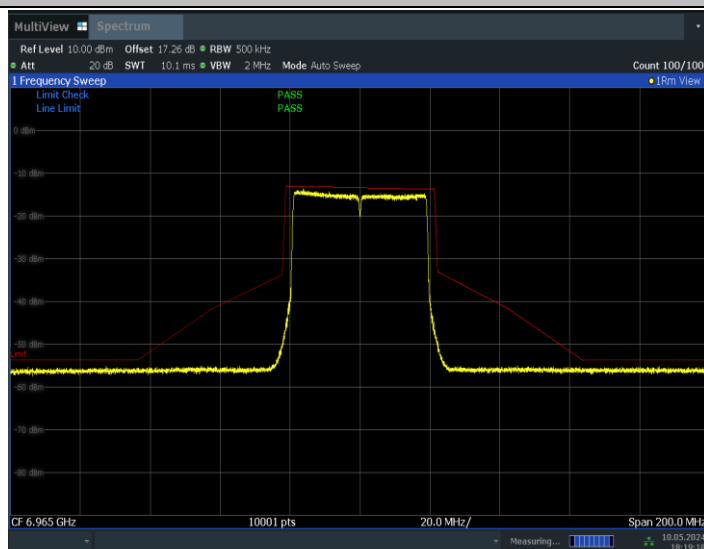
11BE40MIMO_Ant1_6965
