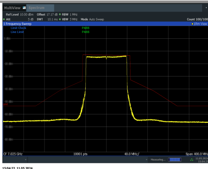
11BE80MIMO_Ant1_7025
