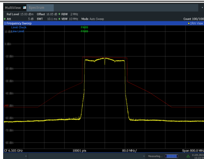
11BE160MIMO_Ant0_6505
