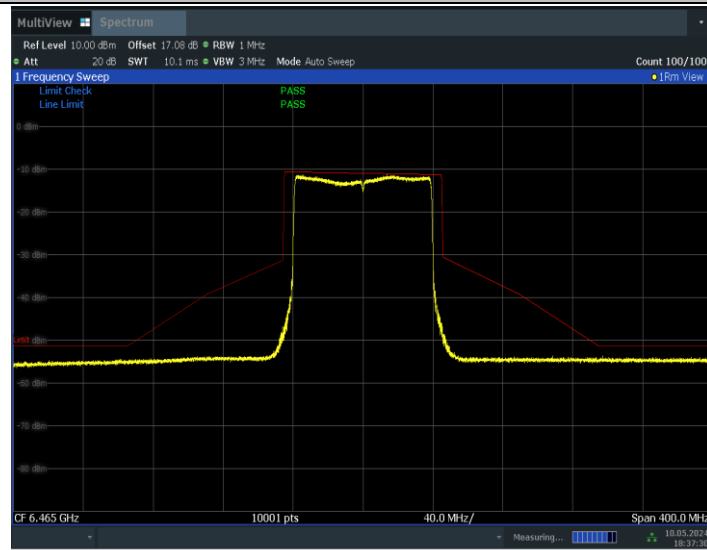
11BE80MIMO_Ant1_6465
