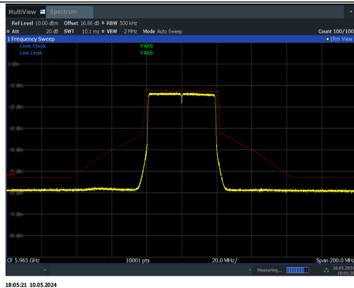
11BE40MIMO_Ant1_5965
