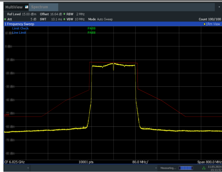
11BE160MIMO_Ant0_6025
