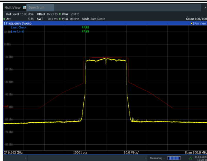
11BE160MIMO_Ant1_6665
