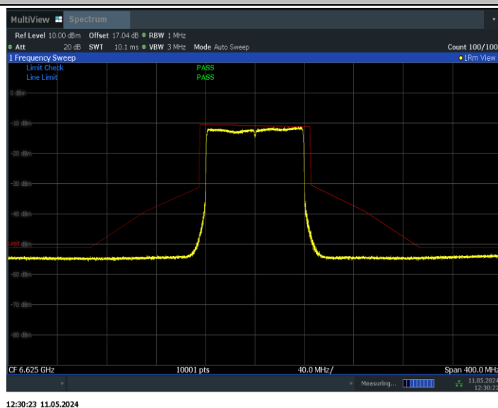
11BE80MIMO_Ant1_6625
