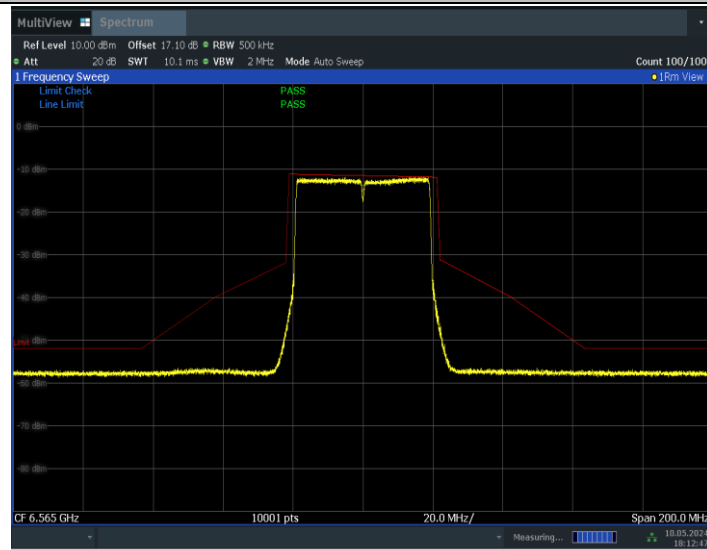
11BE40MIMO_Ant1_6565
