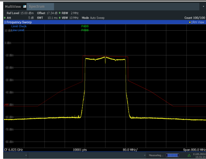
11BE160MIMO_Ant0_6825
