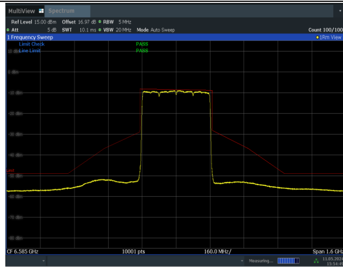
11BE320MIMO_Ant0_6585
