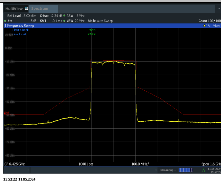
11BE320MIMO_Ant1_6425
