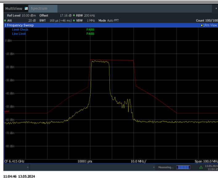
11BE20MIMO_Ant0_6415_106Tone_RU53
