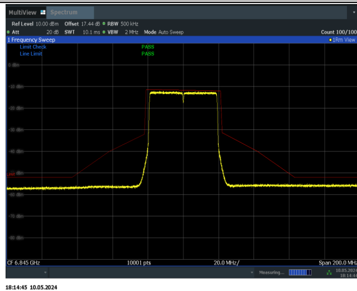
11BE40MIMO_Ant1_6845
