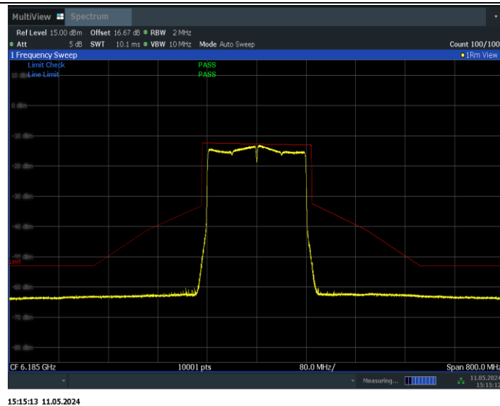
11BE160MIMO_Ant1_6185
