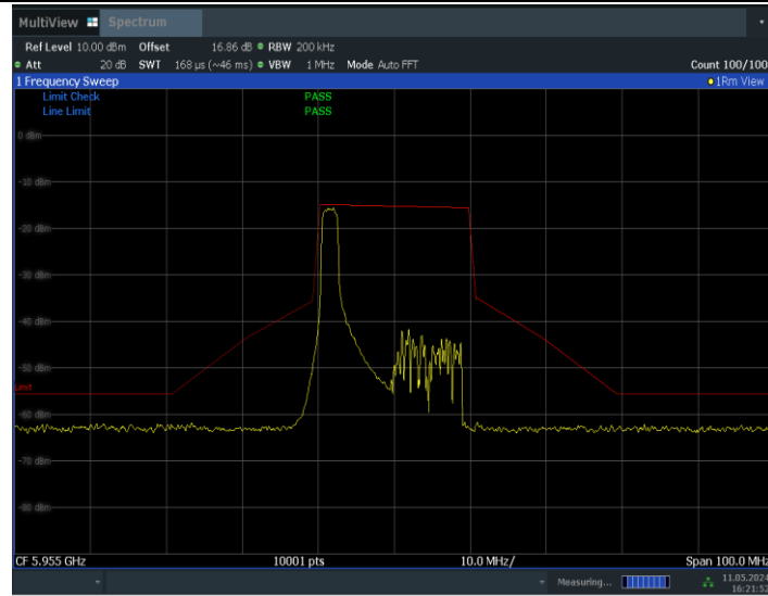
11BE20MIMO_Ant0_5955_26Tone_RU0
