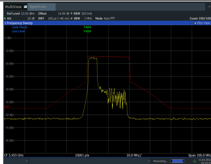
11BE20MIMO_Ant0_5955_52Tone_RU37
