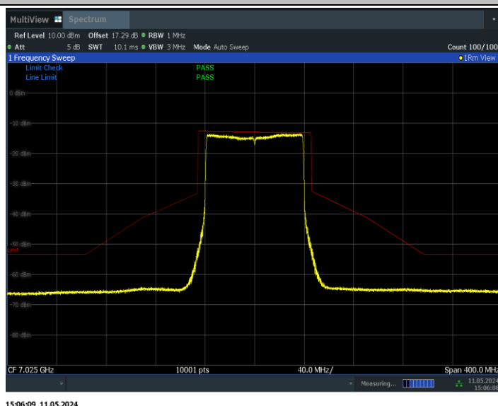
11BE80MIMO_Ant1_7025
