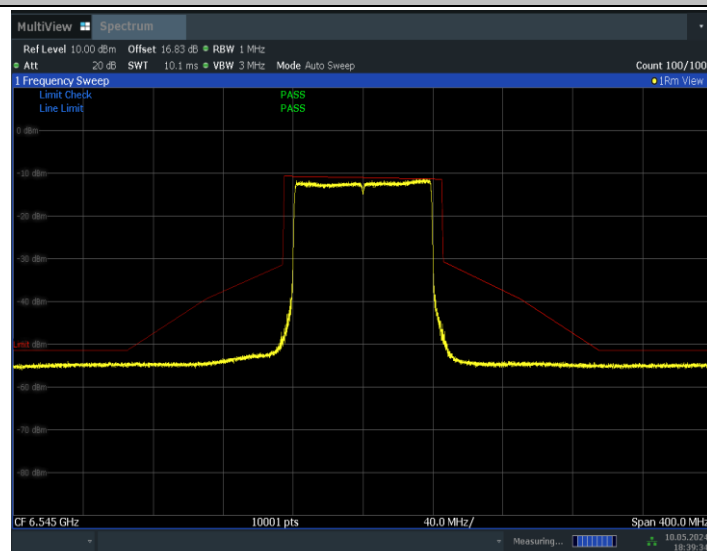
11BE80MIMO_Ant0_6545
