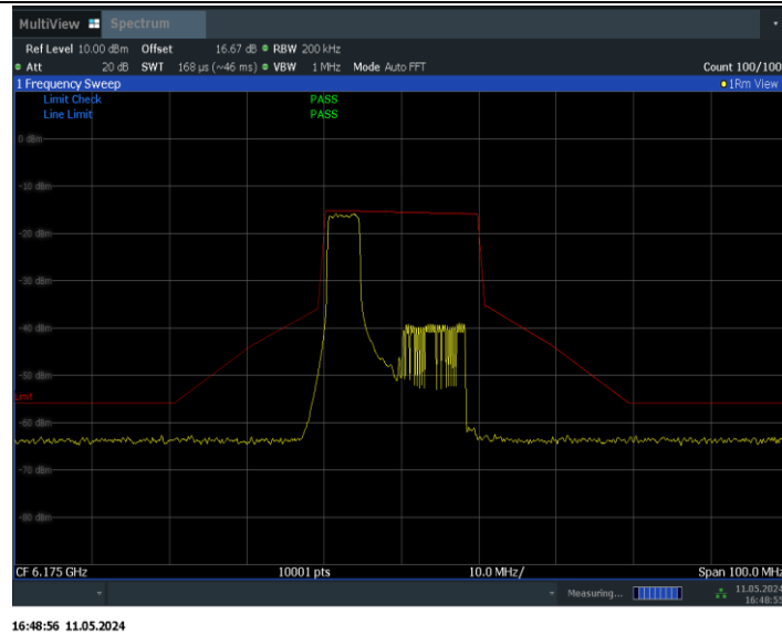
11BE20MIMO_Ant0_6175_106Tone_RU53
