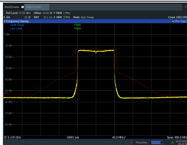
11BE80MIMO_Ant1_6145
