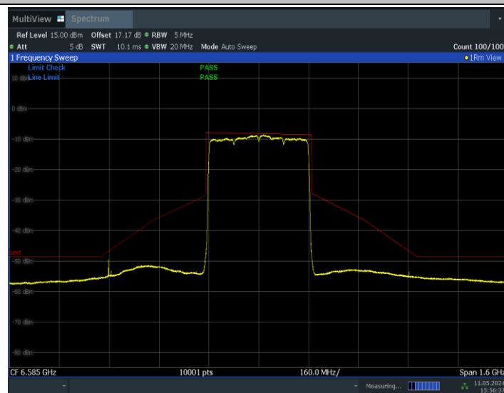
11BE320MIMO_Ant1_6585
