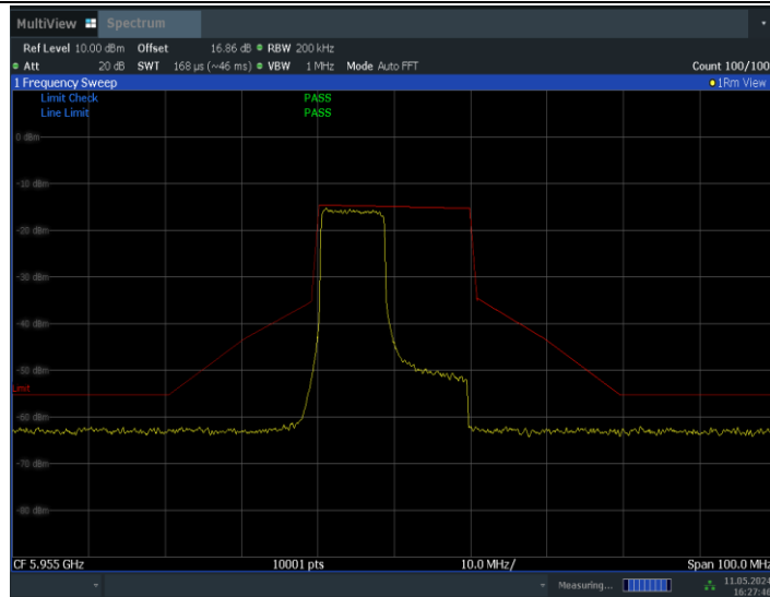
11BE20MIMO_Ant1_5955_26Tone_RU0
