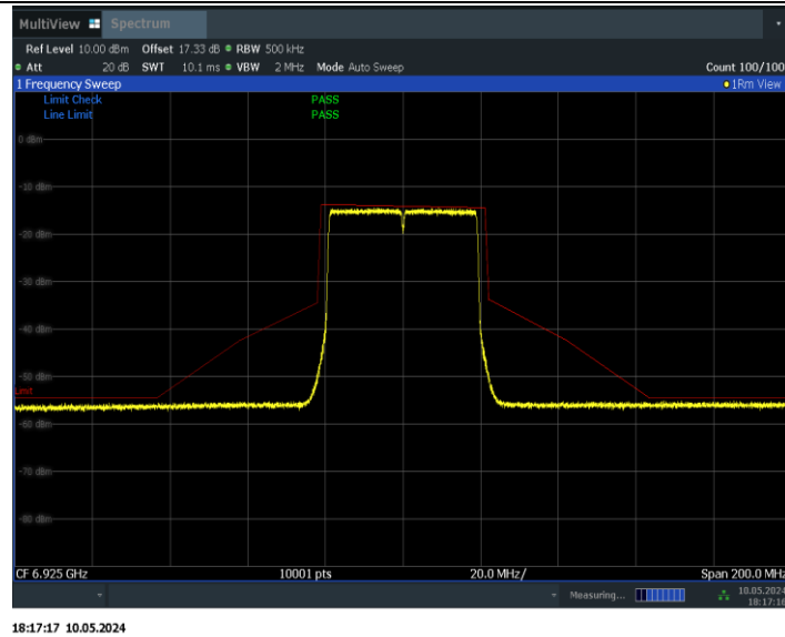
11BE40MIMO_Ant1_6925
