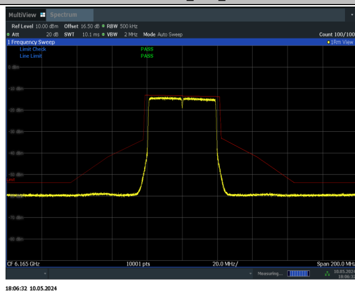
11BE40MIMO_Ant0_6165
