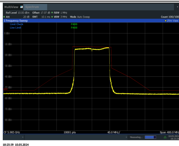
11BE80MIMO_Ant1_5985
