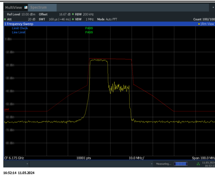
11BE20MIMO_Ant1_6175_26Tone_RU0
