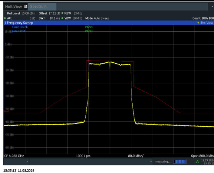
11BE160MIMO_Ant1_6985
