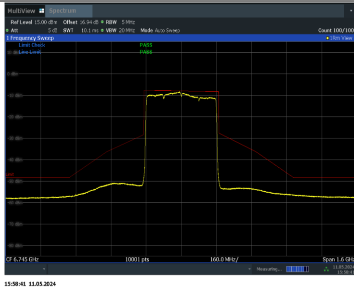
11BE320MIMO_Ant1_6745
