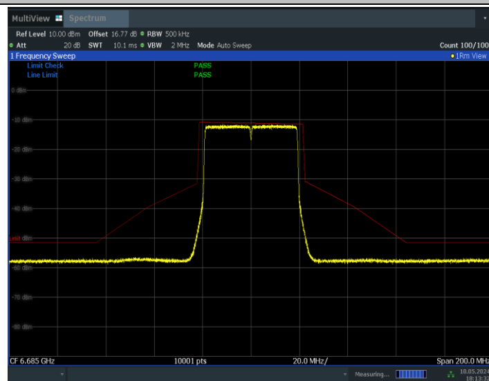
11BE40MIMO_Ant0_6685
