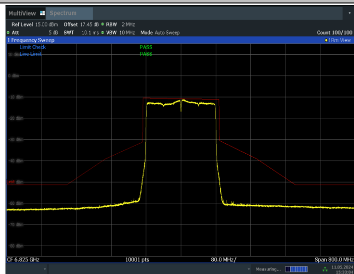
11BE160MIMO_Ant1_6825
