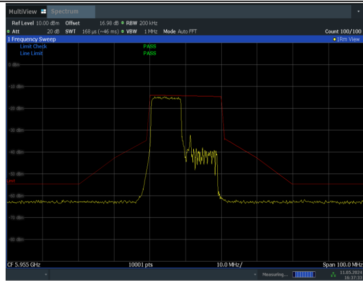
11BE20MIMO_Ant1_5955_106Tone_RU53
