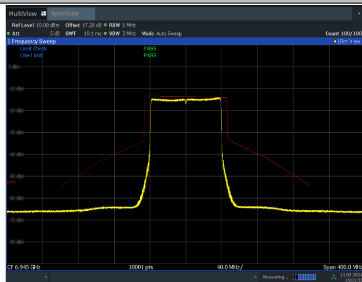
11BE80MIMO_Ant0_6945
