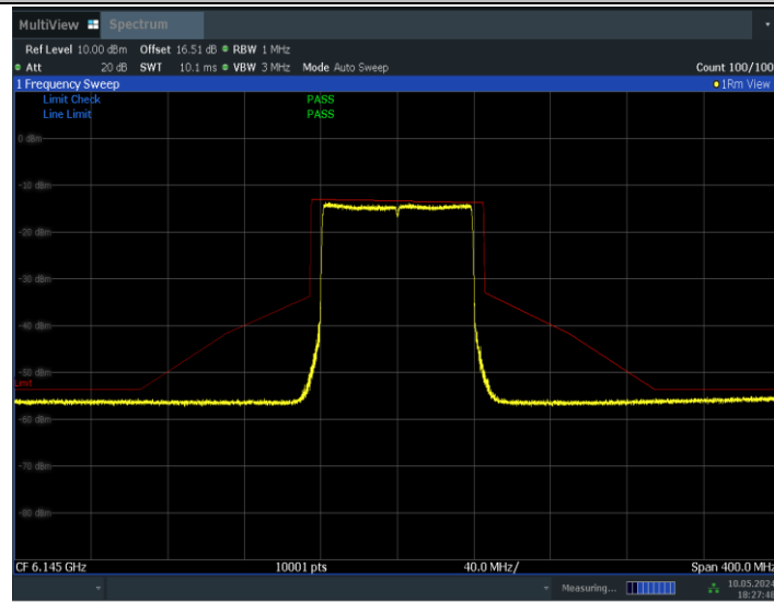
11BE80MIMO_Ant0_6145
