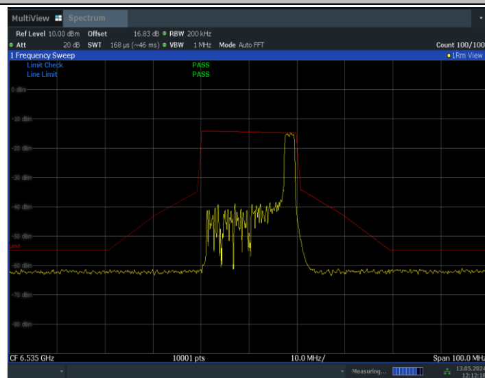
11BE20MIMO_Ant0_6535_26Tone_RU8
