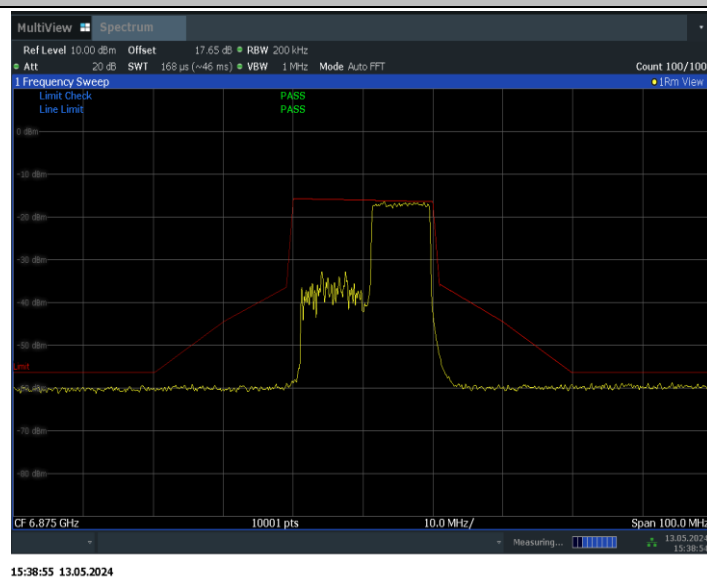
11BE20MIMO_Ant1_6875_106Tone_RU54
