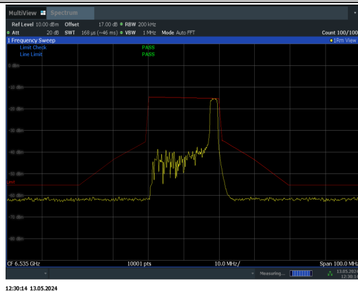
11BE20MIMO_Ant1_6535_26Tone_RU8
