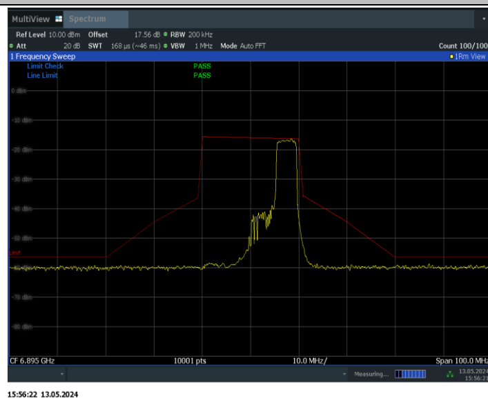
11BE20MIMO_Ant1_6895_52Tone_RU40
