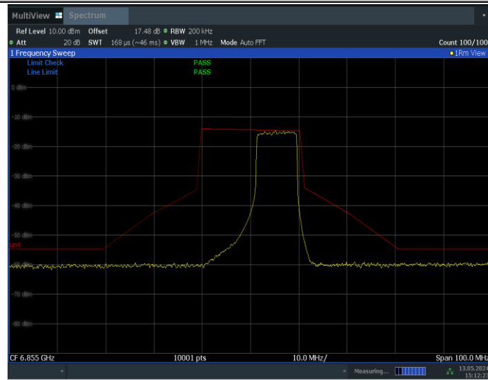
11BE20MIMO_Ant0_6855_106Tone_RU54
