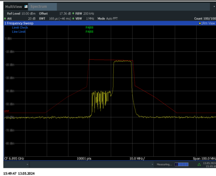
11BE20MIMO_Ant1_6895_26Tone_RU8
