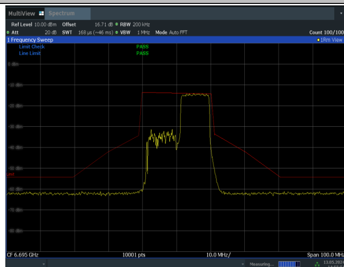
11BE20MIMO_Ant0_6695_106Tone_RU54
