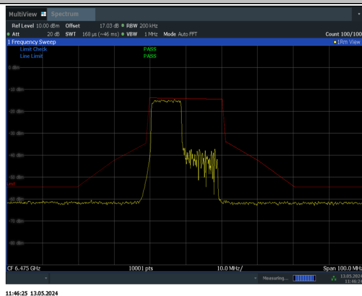
11BE20MIMO_Ant1_6475_106Tone_RU53
