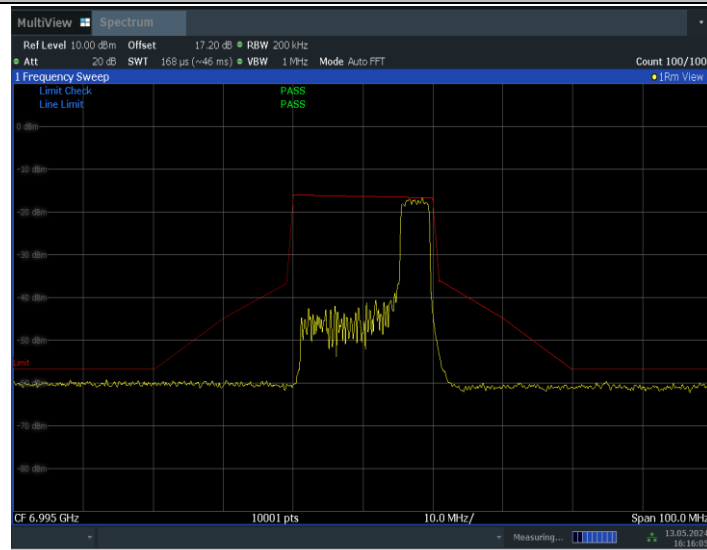
11BE20MIMO_Ant1_6995_52Tone_RU40
