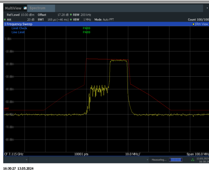
11BE20MIMO_Ant0_7115_106Tone_RU54
