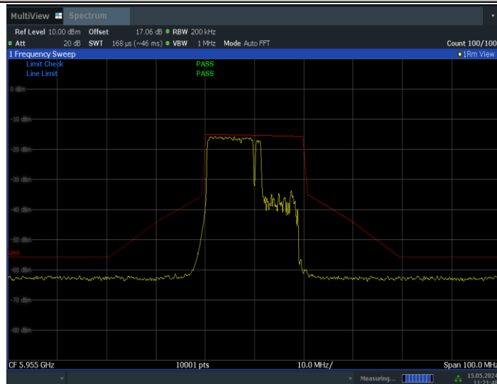
11BE20MIMO_Ant0_5955_106+26_OFDMA_1
