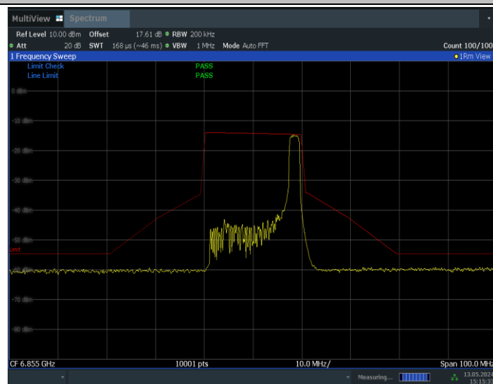
11BE20MIMO_Ant1_6855_26Tone_RU8
