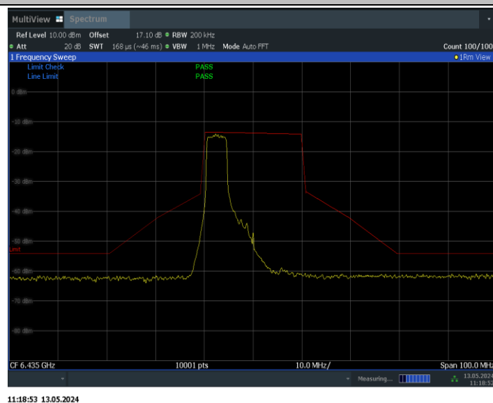
11BE20MIMO_Ant0_6435_52Tone_RU37
