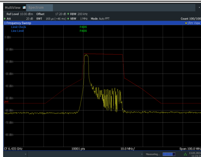
11BE20MIMO_Ant1_6435_26Tone_RU0
