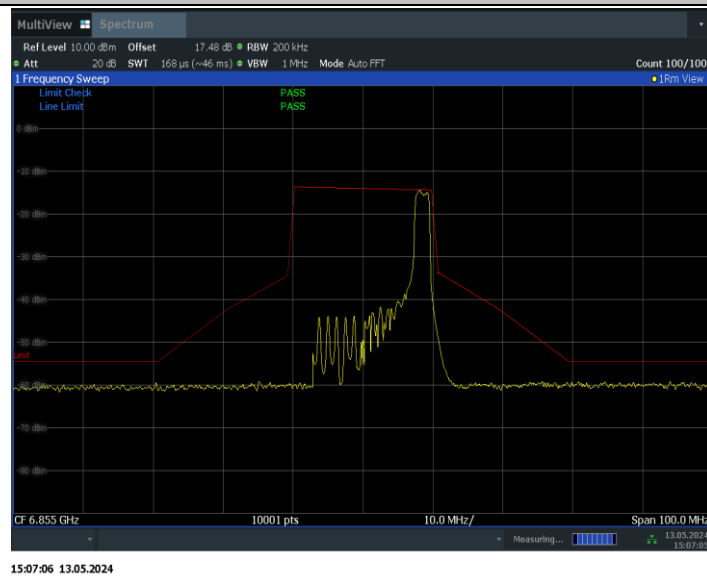
11BE20MIMO_Ant0_6855_52Tone_RU40
