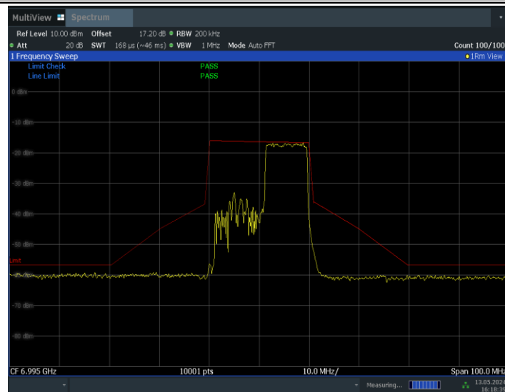
11BE20MIMO_Ant1_6995_106Tone_RU54
