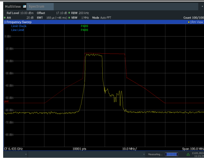
11BE20MIMO_Ant0_6435_106Tone_RU53
