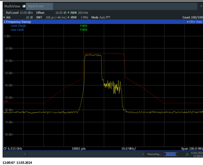
11BE20MIMO_Ant1_6515_26Tone_RU0
