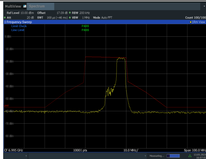
11BE20MIMO_Ant0_6995_106Tone_RU54
