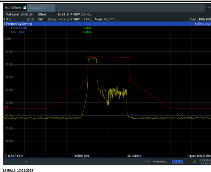
11BE20MIMO_Ant1_6515_52Tone_RU37
