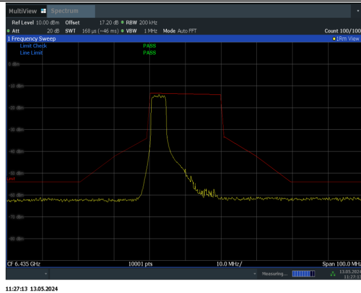
11BE20MIMO_Ant1_6435_106Tone_RU53
