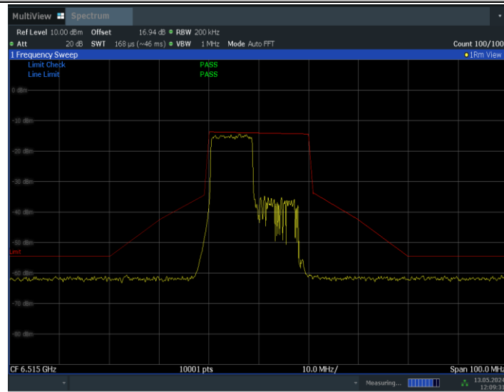
11BE20MIMO_Ant1_6515_106Tone_RU53
