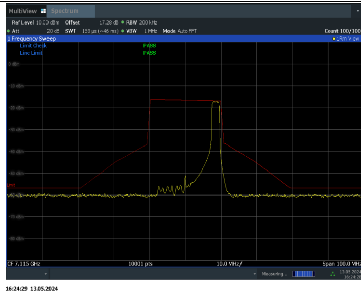
11BE20MIMO_Ant0_7115_52Tone_RU40
