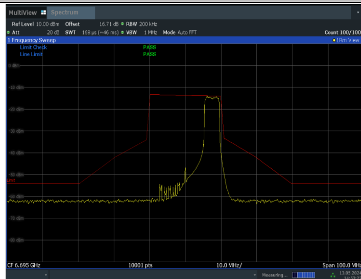
11BE20MIMO_Ant0_6695_52Tone_RU40
