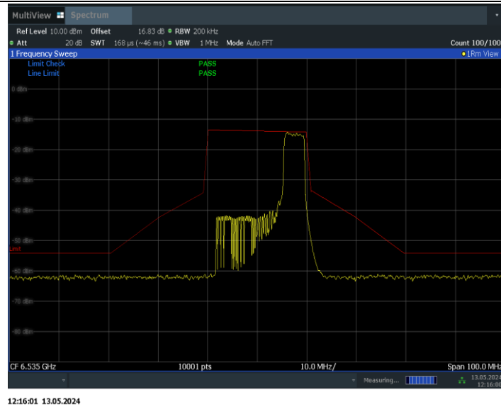
11BE20MIMO_Ant0_6535_106Tone_RU54
