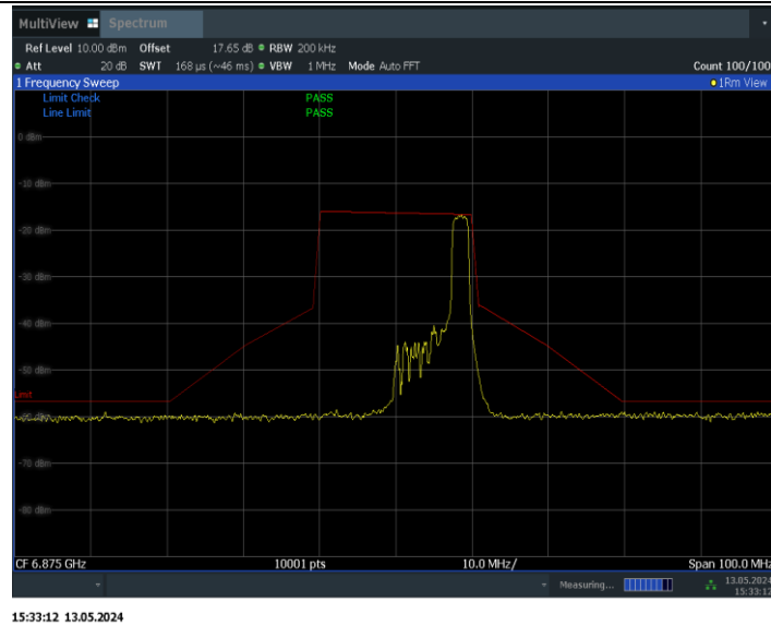
11BE20MIMO_Ant1_6875_52Tone_RU40
