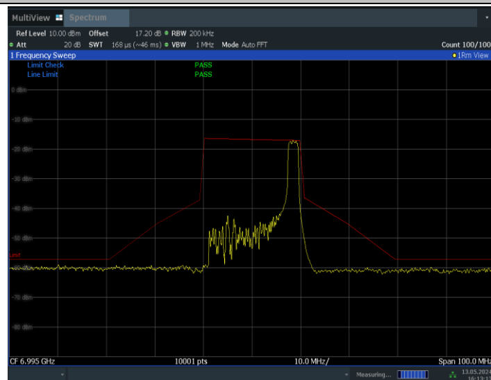
11BE20MIMO_Ant1_6995_26Tone_RU8
