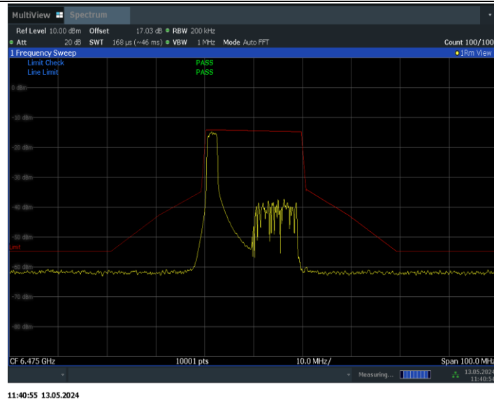
11BE20MIMO_Ant1_6475_52Tone_RU37
