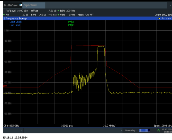
11BE20MIMO_Ant1_6855_106Tone_RU54
