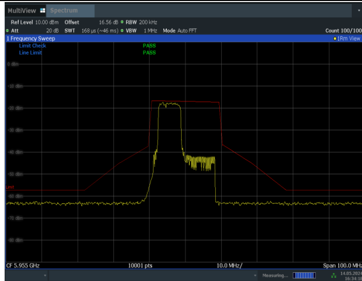
11BE20MIMO_Ant0_5955_52+26_OFDMA_1
