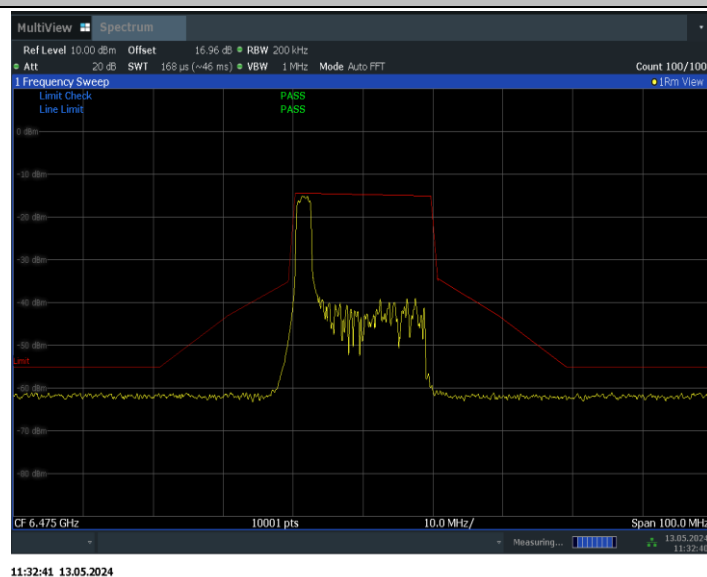
11BE20MIMO_Ant0_6475_26Tone_RU0
