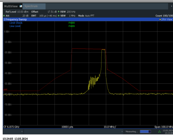
11BE20MIMO_Ant0_6875_26Tone_RU8
