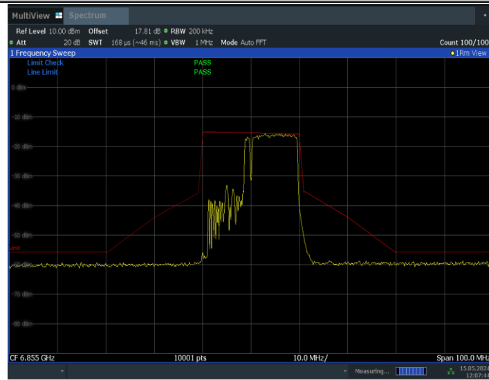
11BE20MIMO_Ant1_6855_106+26_OFDMA_2
