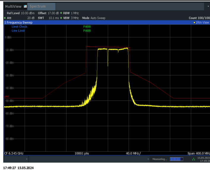
11BE80MIMO_Ant1_6545_484+242_Non-OFDMA_2
