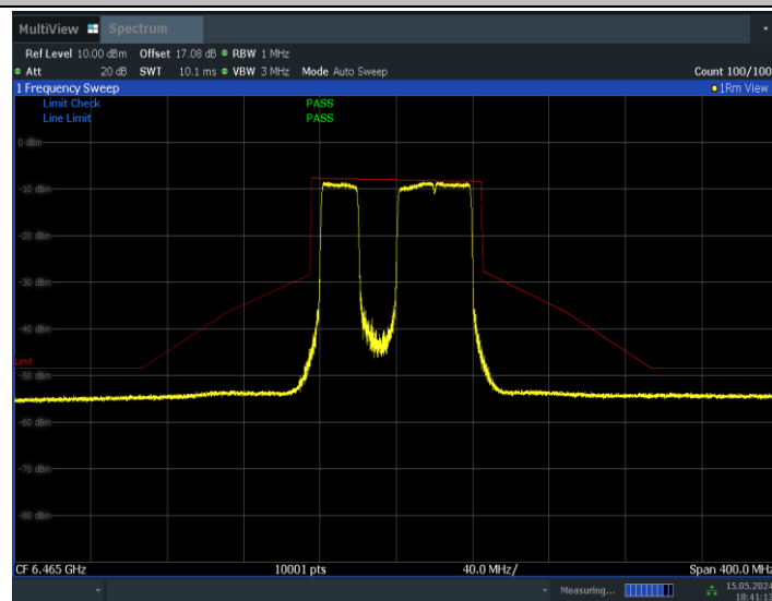
11BE80MIMO_Ant1_6465_484+242_Non-OFDMA_2
