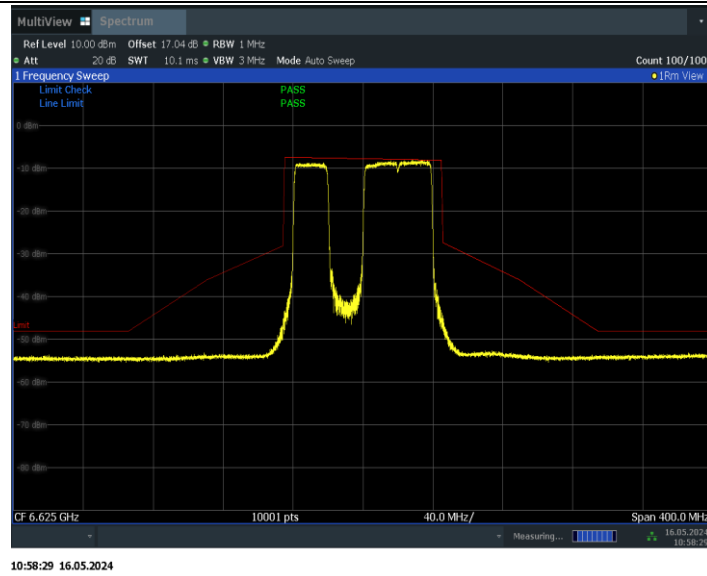
11BE80MIMO_Ant1_6625_484+242_Non-OFDMA_3
