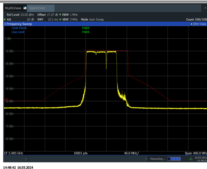
11BE80MIMO_Ant1_5985_484+242_Non-OFDMA_4
