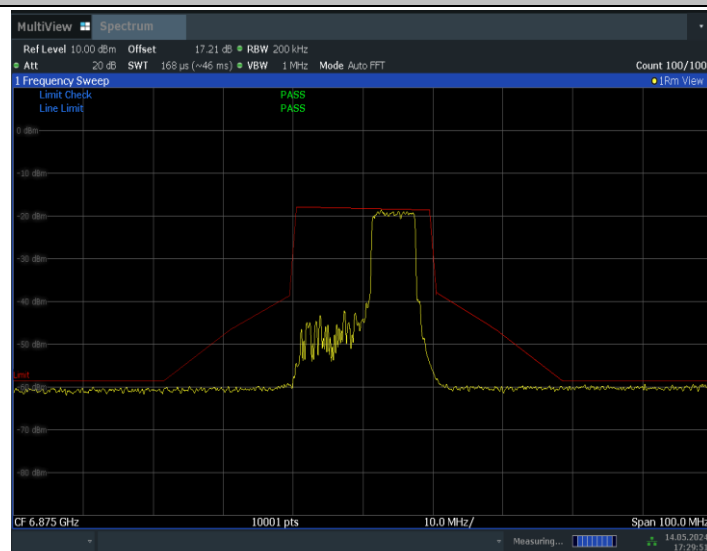
11BE20MIMO_Ant0_6875_52+26_OFDMA_3
