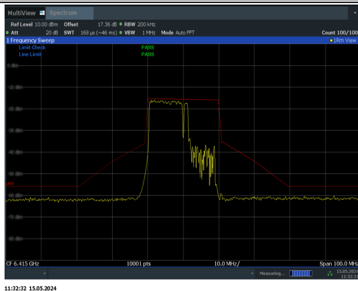
11BE20MIMO_Ant0_6415_106+26_OFDMA_1
