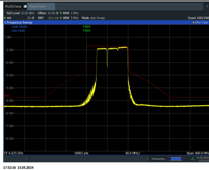
11BE80MIMO_Ant0_6625_484+242_Non-OFDMA_2
