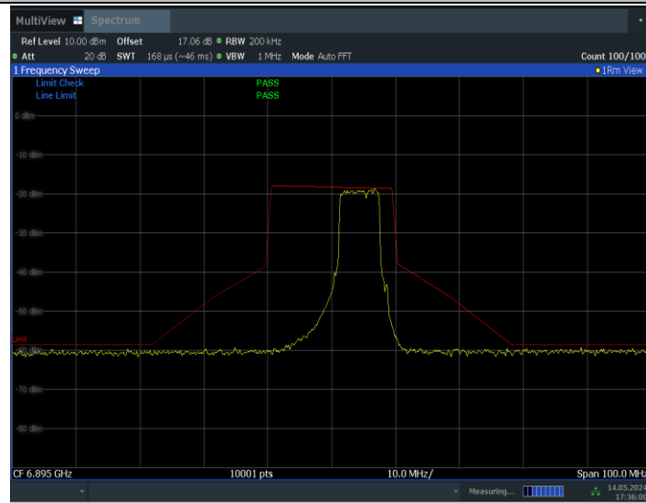
11BE20MIMO_Ant0_6895_52+26_OFDMA_3
