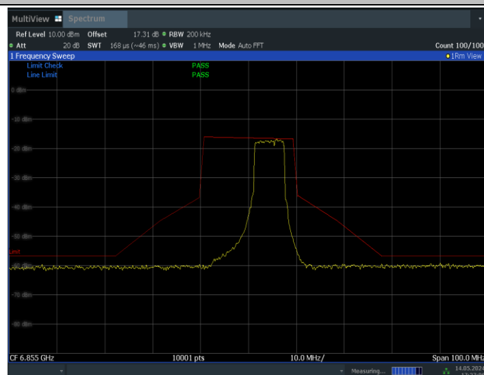
11BE20MIMO_Ant1_6855_52+26_OFDMA_3
