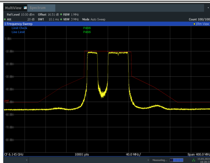
11BE80MIMO_Ant0_6145_484+242_Non-OFDMA_2
