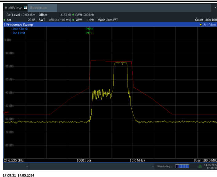
11BE20MIMO_Ant0_6535_52+26_OFDMA_3
