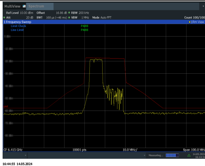
11BE20MIMO_Ant0_6415_106+26_OFDMA_1
