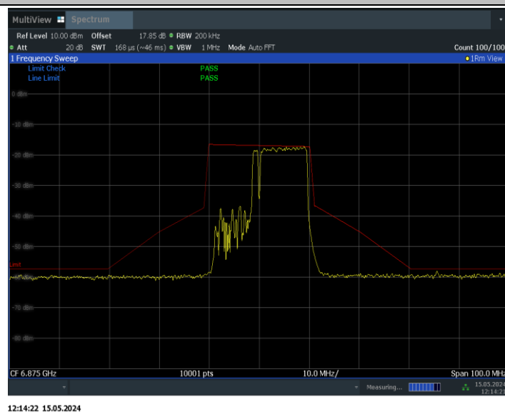
11BE20MIMO_Ant1_6875_106+26_OFDMA_2
