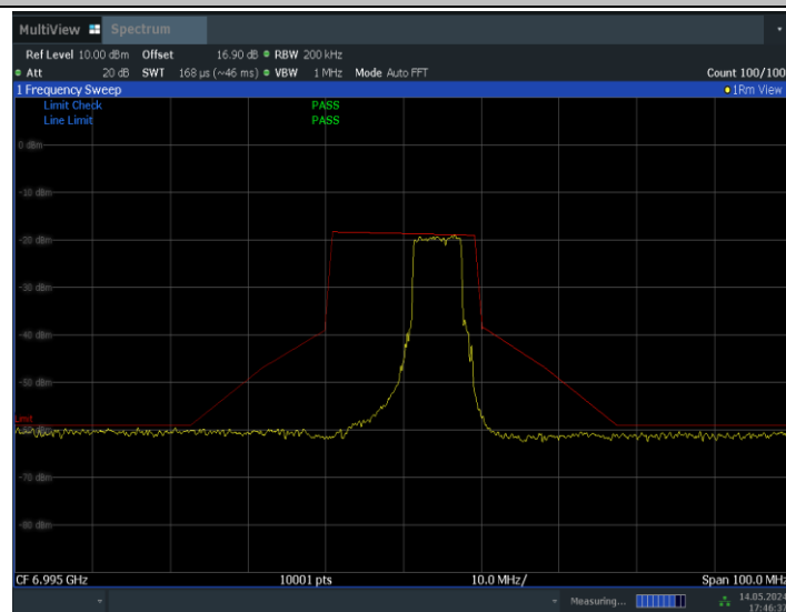
11BE20MIMO_Ant1_6995_52+26_OFDMA_3
