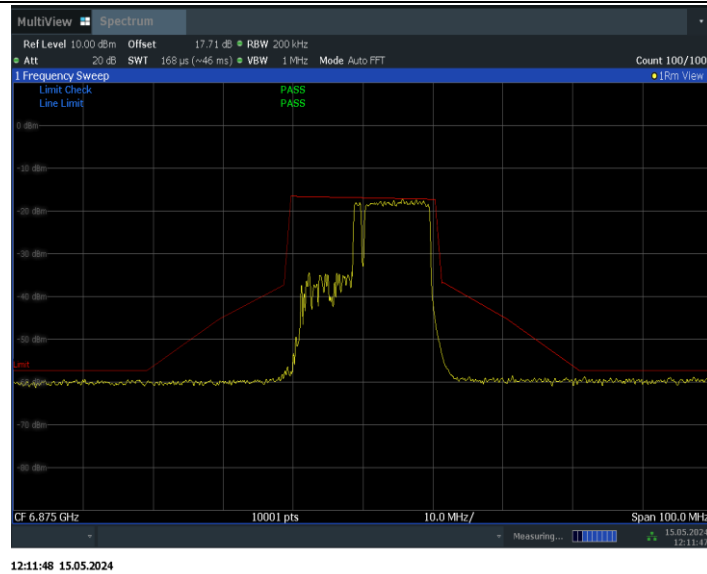
11BE20MIMO_Ant1_6875_52+26_OFDMA_3
