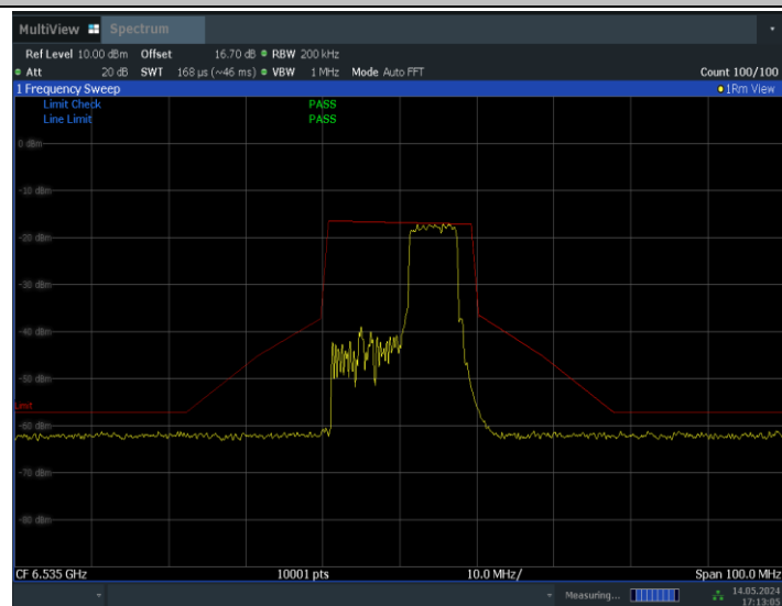
11BE20MIMO_Ant1_6535_52+26_OFDMA_3
