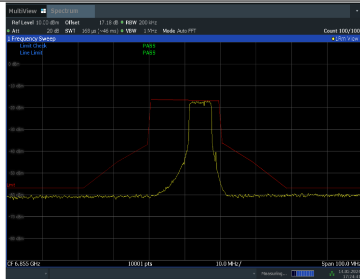
11BE20MIMO_Ant0_6855_106+26_OFDMA_2
