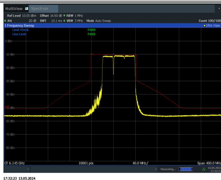
11BE80MIMO_Ant1_6145_484+242_Non-OFDMA_1
