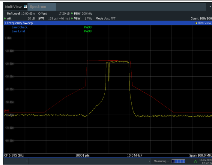
11BE20MIMO_Ant0_6995_106+26_OFDMA_2
