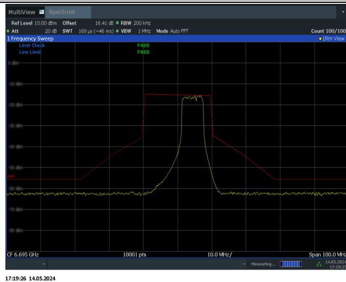
11BE20MIMO_Ant0_6695_106+26_OFDMA_2
