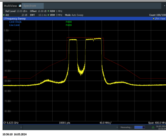
11BE80MIMO_Ant0_6625_484+242_Non-OFDMA_3
