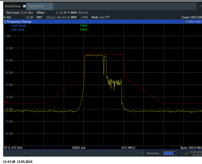
11BE20MIMO_Ant1_6475_52+26_OFDMA_1
