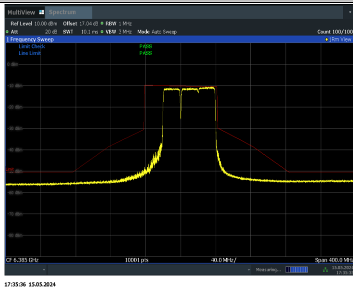
11BE80MIMO_Ant0_6385_484+242_Non-OFDMA_2
