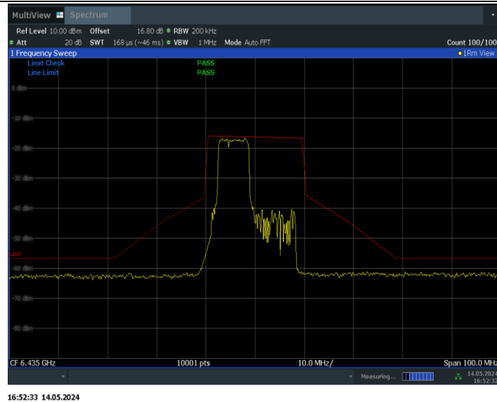
11BE20MIMO_Ant0_6435_106+26_OFDMA_1
