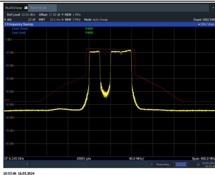
11BE80MIMO_Ant1_6545_484+242_Non-OFDMA_2
