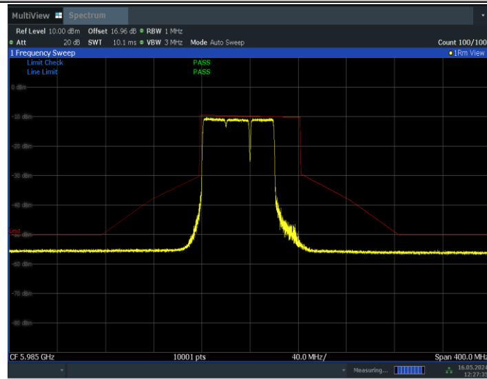
11BE80MIMO_Ant0_5985_484+242_Non-OFDMA_4
