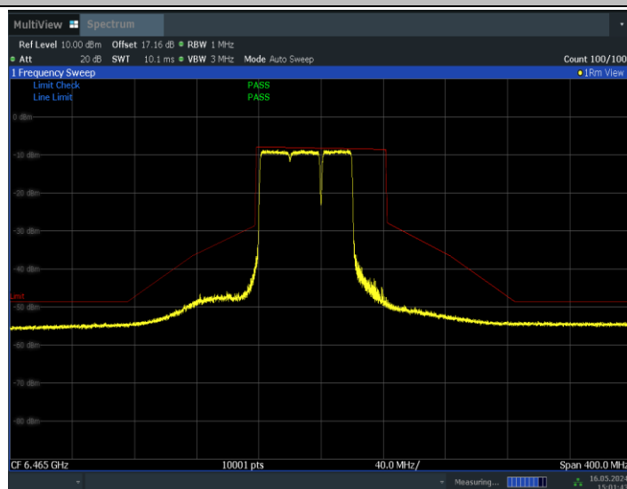
11BE80MIMO_Ant0_6465_484+242_Non-OFDMA_4
