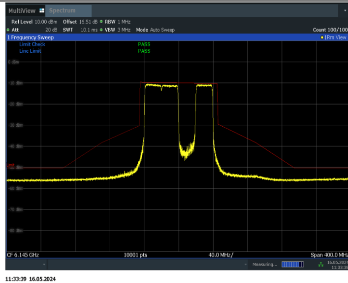
11BE80MIMO_Ant0_6145_484+242_Non-OFDMA_4
