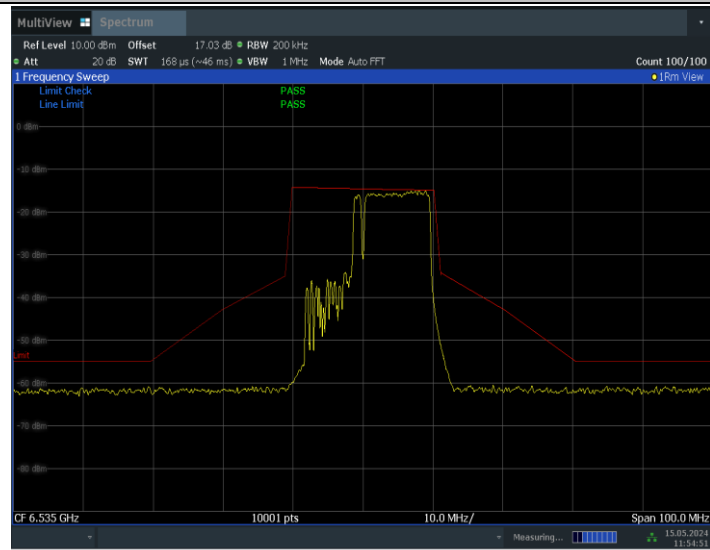
11BE20MIMO_Ant0_6535_106+26_OFDMA_2
