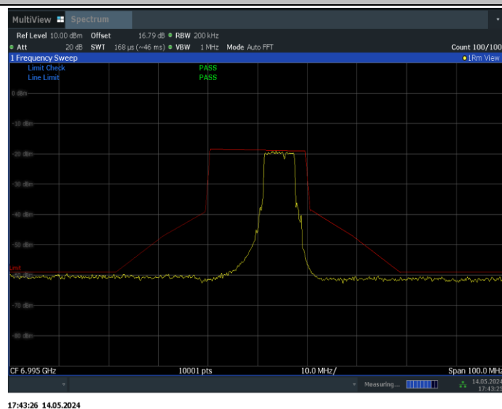
11BE20MIMO_Ant0_6995_52+26_OFDMA_3
