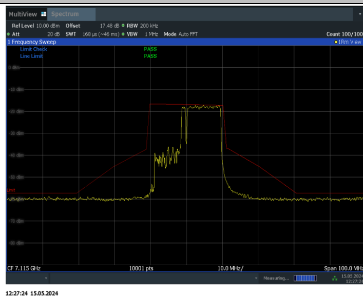
11BE20MIMO_Ant0_7115_106+26_OFDMA_2
