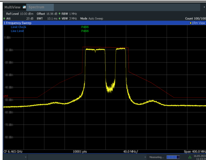
11BE80MIMO_Ant0_6465_484+242_Non-OFDMA_3
