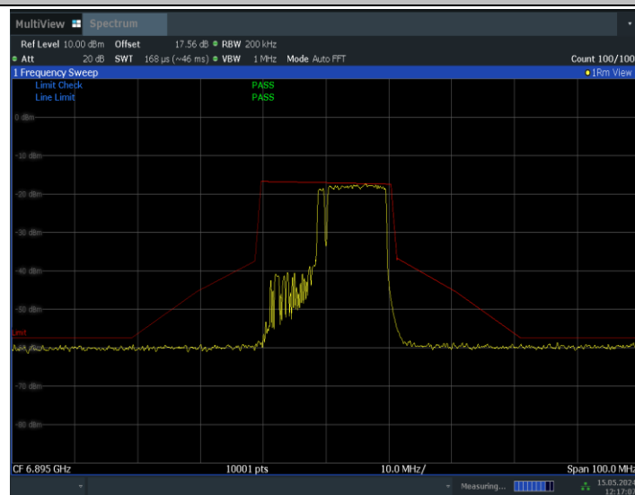
11BE20MIMO_Ant0_6895_106+26_OFDMA_2
