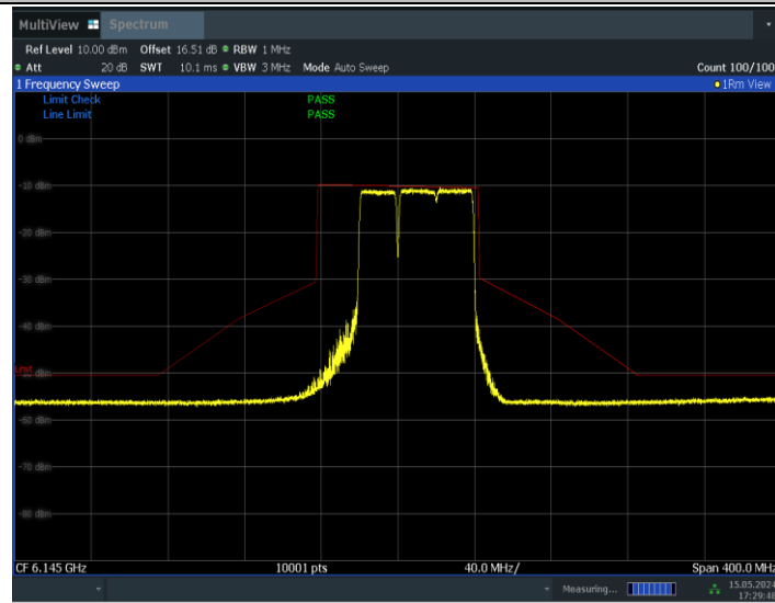
11BE80MIMO_Ant0_6145_484+242_Non-OFDMA_1
