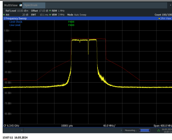
11BE80MIMO_Ant1_6545_484+242_Non-OFDMA_1
