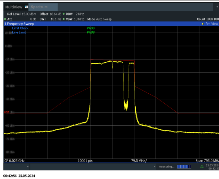
11BE160MIMO_Ant0_6025_996+484+242_Non-OFDMA_8
