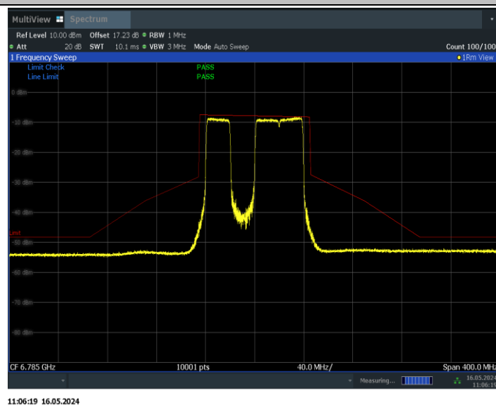
11BE80MIMO_Ant0_6785_484+242_Non-OFDMA_2
