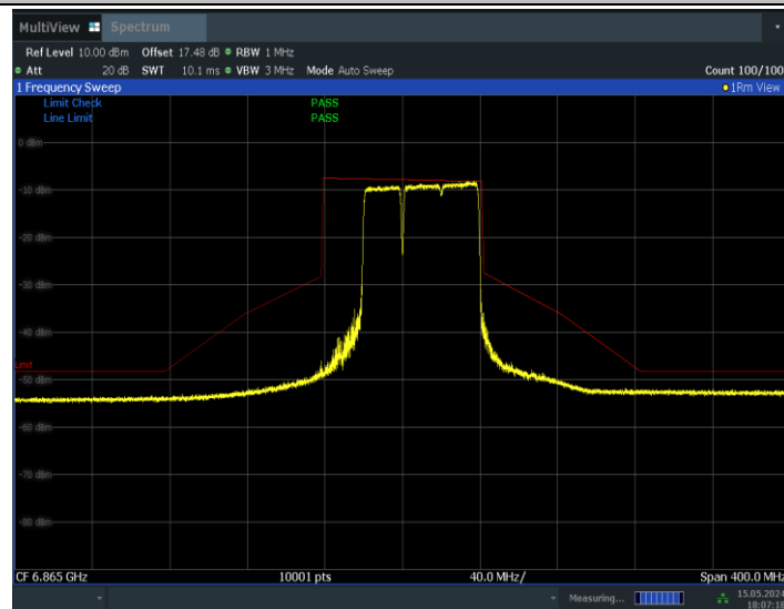
11BE80MIMO_Ant0_6865_484+242_Non-OFDMA_1
