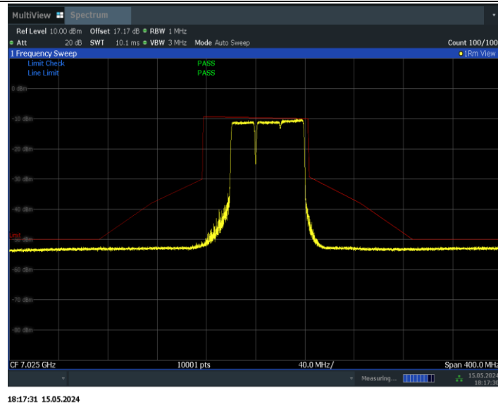
11BE80MIMO_Ant0_7025_484+242_Non-OFDMA_2
