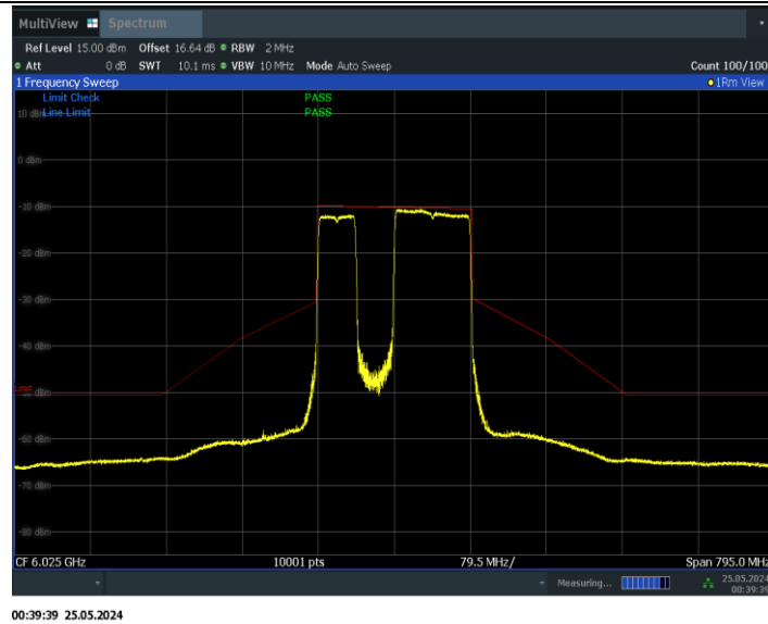
11BE160MIMO_Ant0_6025_996+484_Non-OFDMA_4
