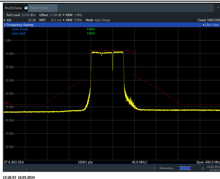
11BE80MIMO_Ant0_6865_484+242_Non-OFDMA_4
