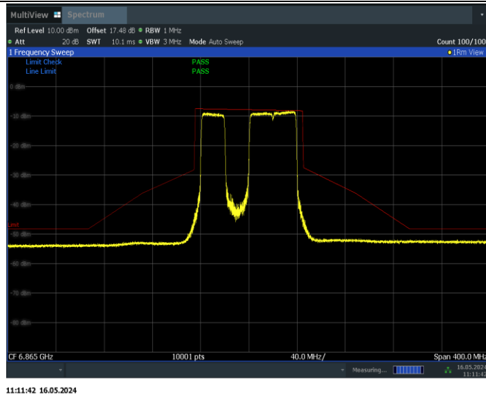
11BE80MIMO_Ant0_6865_484+242_Non-OFDMA_3
