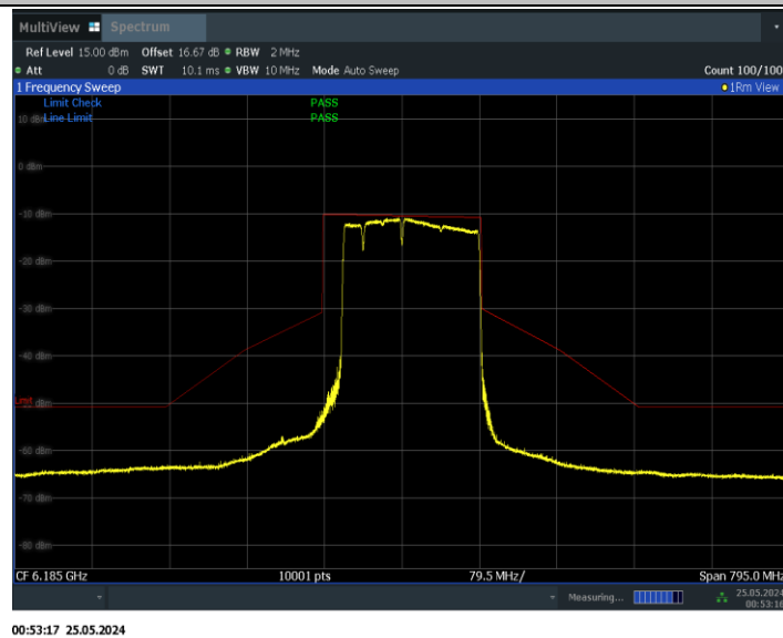
11BE160MIMO_Ant0_6185_996+484+242_Non-OFDMA_2
