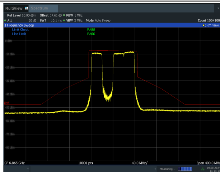
11BE80MIMO_Ant1_6865_484+242_Non-OFDMA_2
