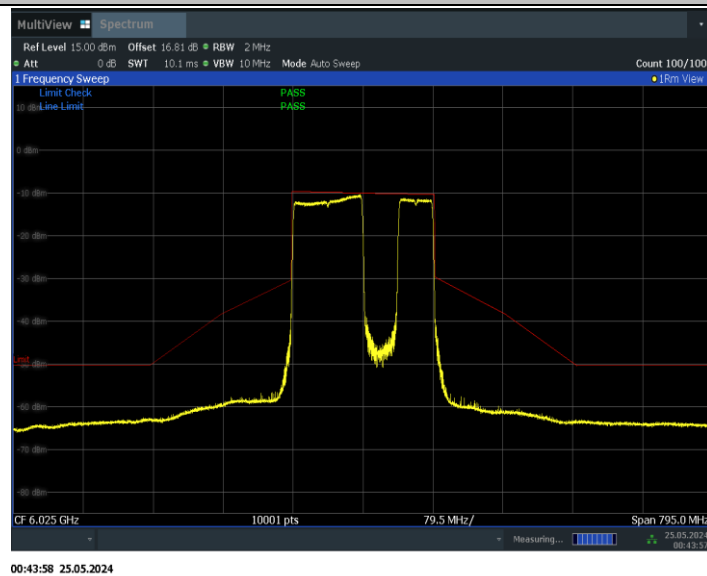
11BE160MIMO_Ant1_6025_996+484_Non-OFDMA_3
