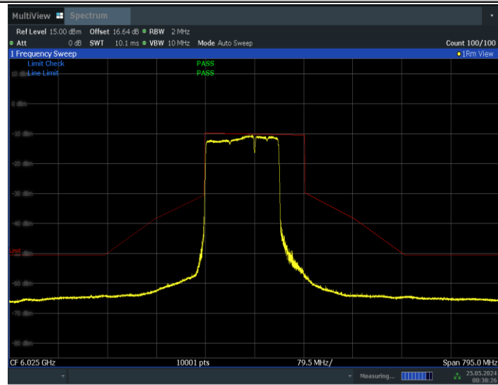
11BE160MIMO_Ant0_6025_996+484_Non-OFDMA_1
