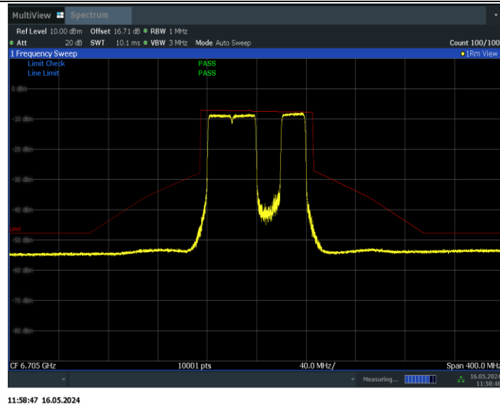
11BE80MIMO_Ant0_6705_484+242_Non-OFDMA_4
