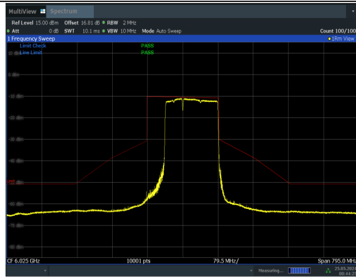
11BE160MIMO_Ant1_6025_996+484_Non-OFDMA_4
