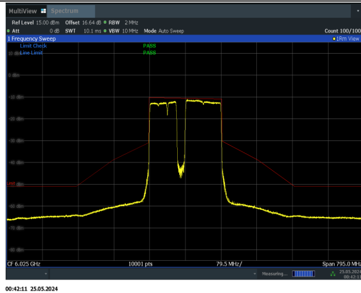
11BE160MIMO_Ant0_6025_996+484+242_Non-OFDMA_5
