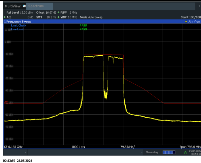
11BE160MIMO_Ant0_6185_996+484+242_Non-OFDMA_6
