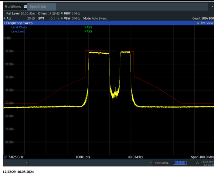
11BE80MIMO_Ant1_7025_484+242_Non-OFDMA_4
