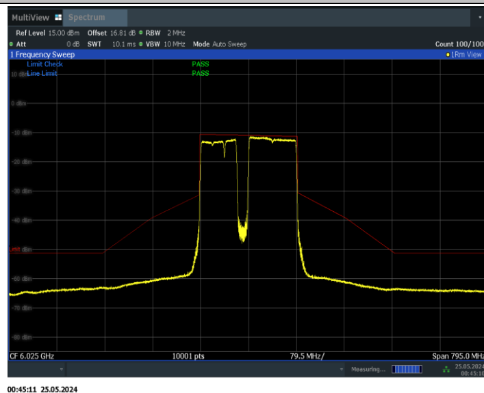
11BE160MIMO_Ant1_6025_996+484+242_Non-OFDMA_4
