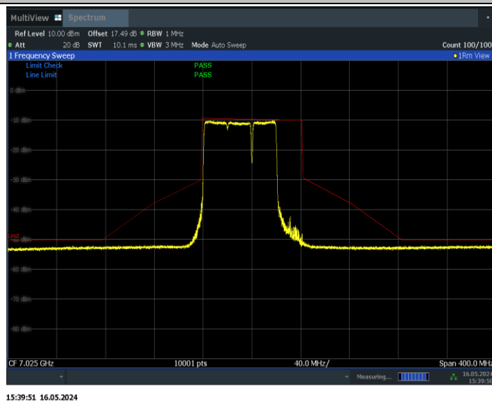
11BE80MIMO_Ant1_7025_484+242_Non-OFDMA_4
