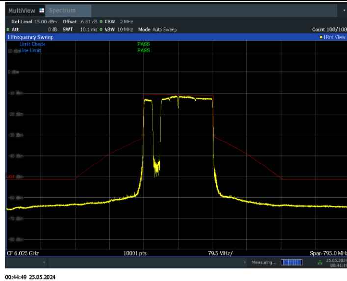
11BE160MIMO_Ant1_6025_996+484+242_Non-OFDMA_3
