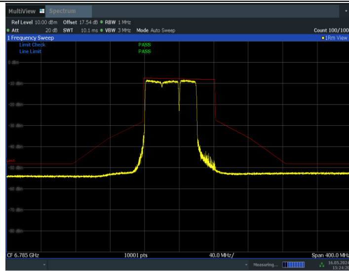
11BE80MIMO_Ant1_6785_484+242_Non-OFDMA_4
