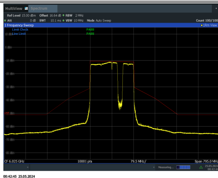
11BE160MIMO_Ant0_6025_996+484+242_Non-OFDMA_6
