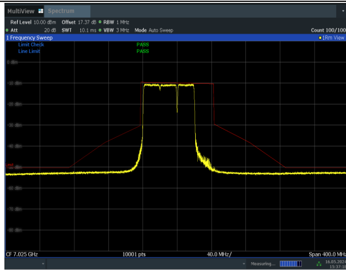
11BE80MIMO_Ant0_7025_484+242_Non-OFDMA_4
