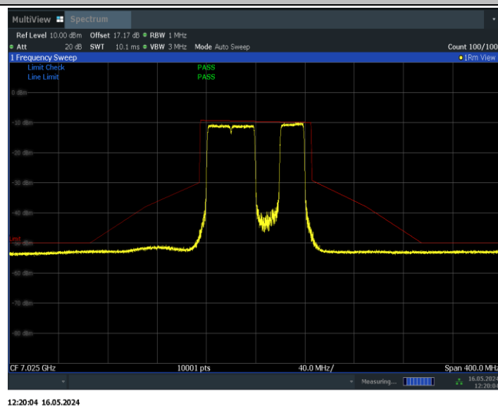
11BE80MIMO_Ant0_7025_484+242_Non-OFDMA_3
