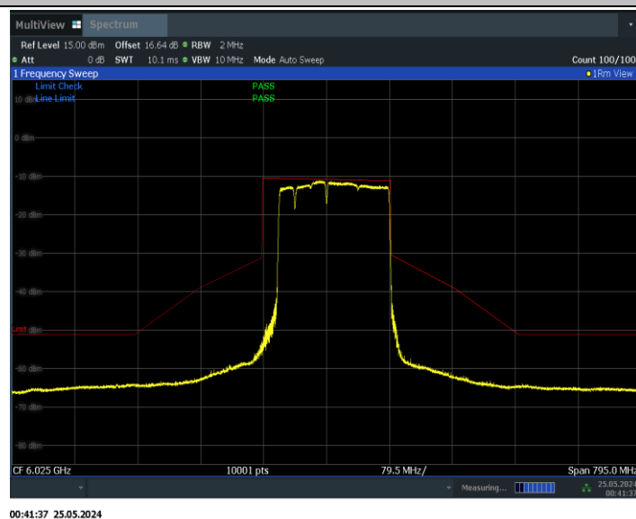
11BE160MIMO_Ant0_6025_996+484+242_Non-OFDMA_1
