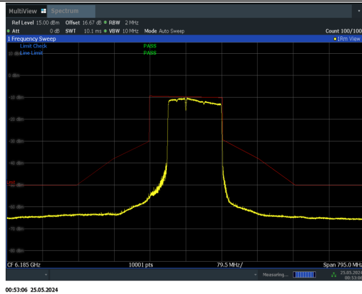
11BE160MIMO_Ant0_6185_996+484+242_Non-OFDMA_1
