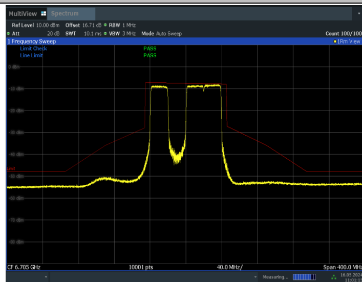
11BE80MIMO_Ant0_6705_484+242_Non-OFDMA_2
