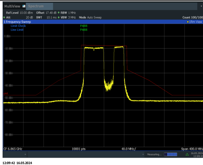
11BE80MIMO_Ant0_6865_484+242_Non-OFDMA_4
