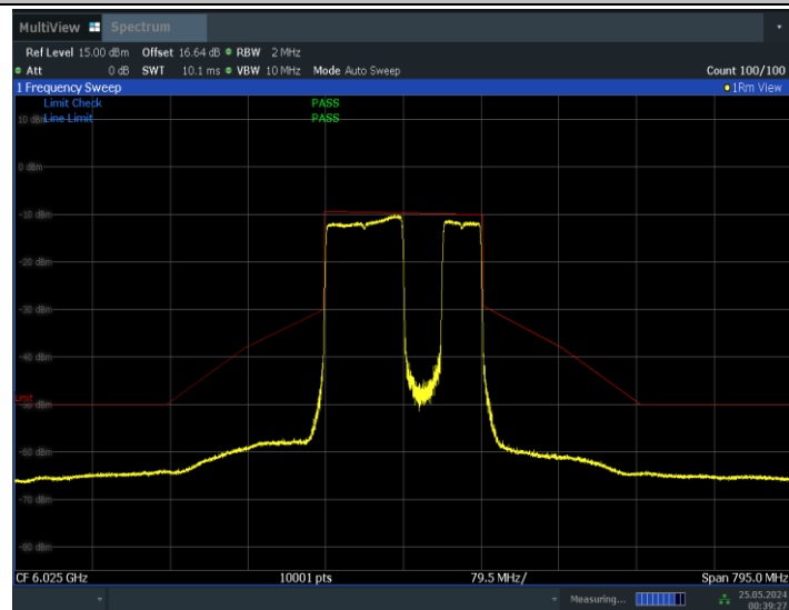
11BE160MIMO_Ant0_6025_996+484_Non-OFDMA_2
