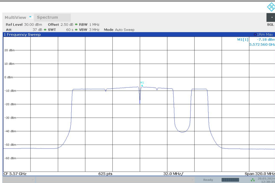
11BE160MIMO_Ant0_5570_996+484+242_OFDMA_7
