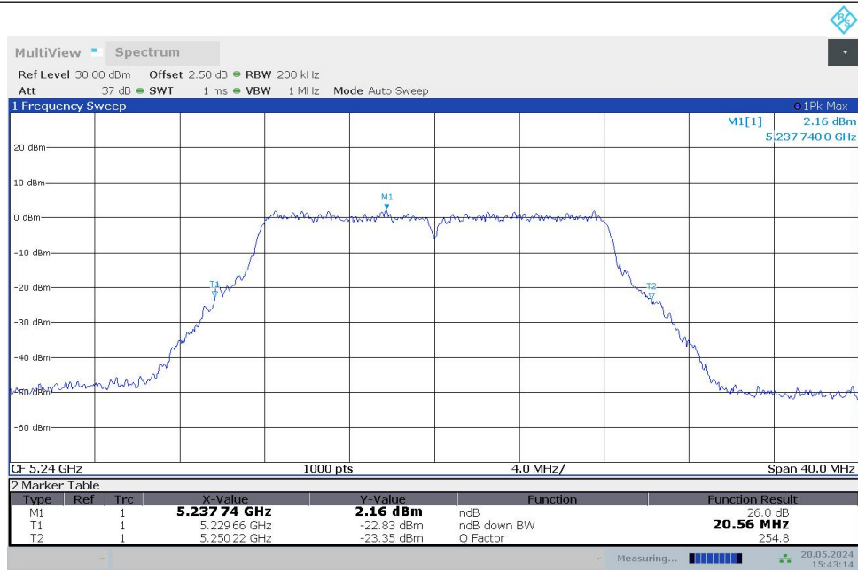
11A-MIMO_Ant1_5240
