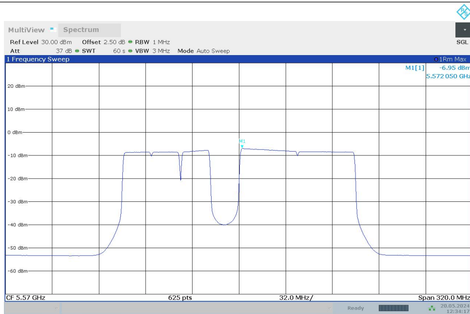
11BE160MIMO_Ant0_5570_996+484+242_OFDMA_5
