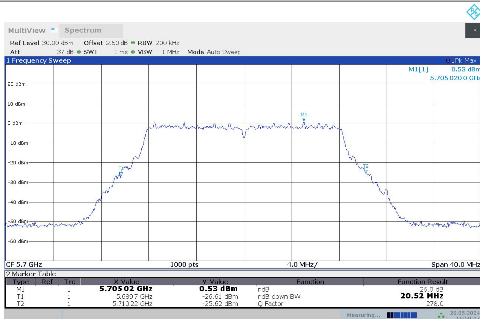
11A-MIMO_Ant1_5700
