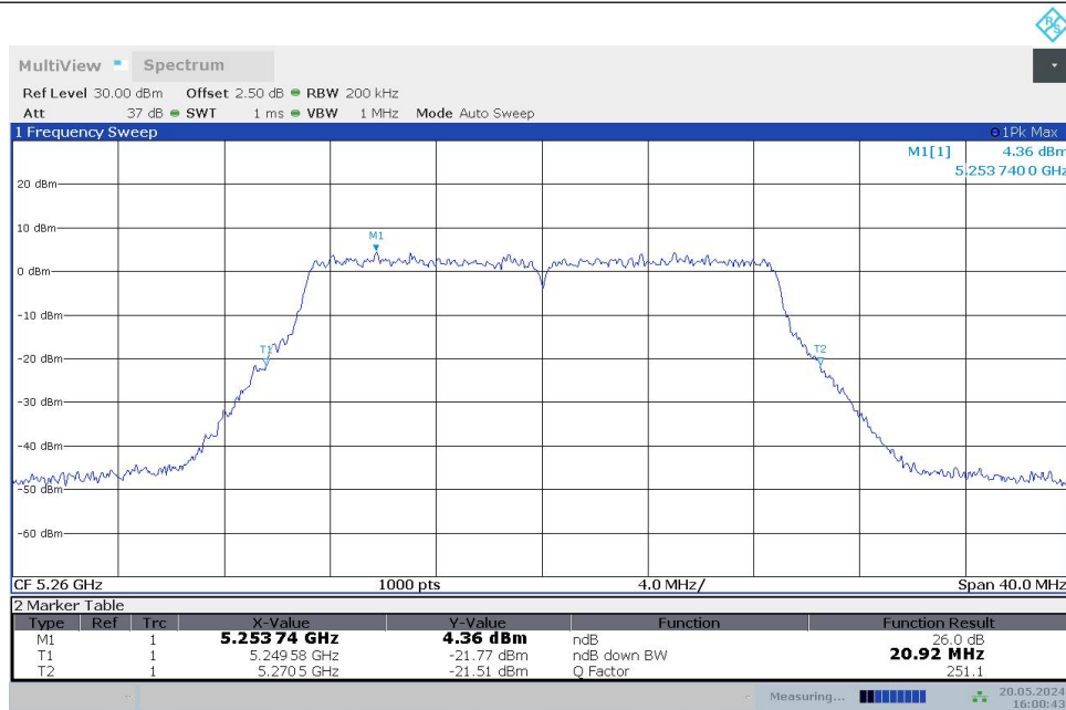
11AC20MIMO_Ant1_5260
