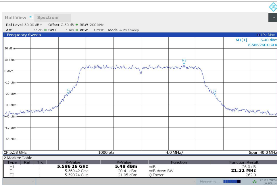
11AC20MIMO_Ant1_5580
