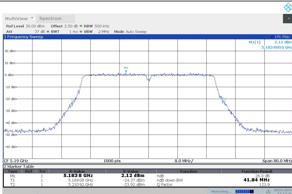
11N40MIMO_Ant1_5190
