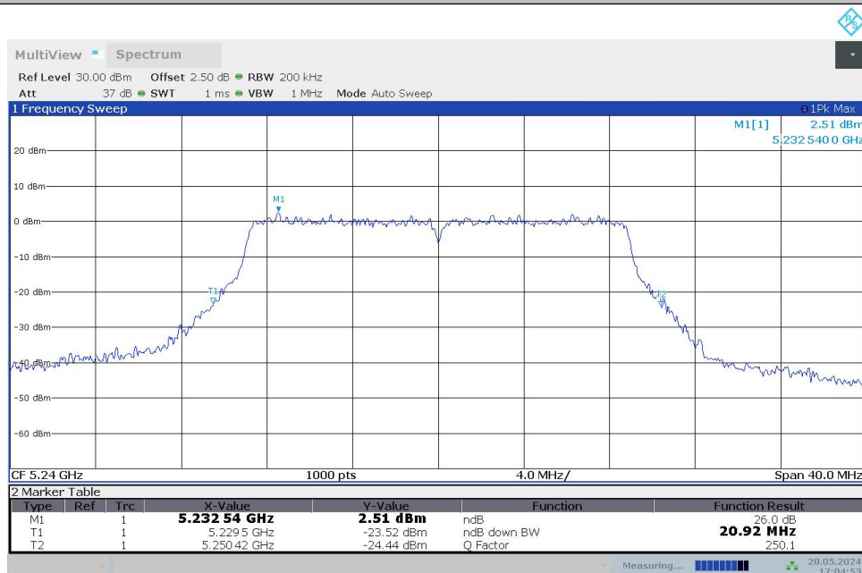
11AC20MIMO_Ant1_5240
