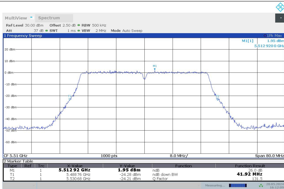
11N40MIMO_Ant1_5510
