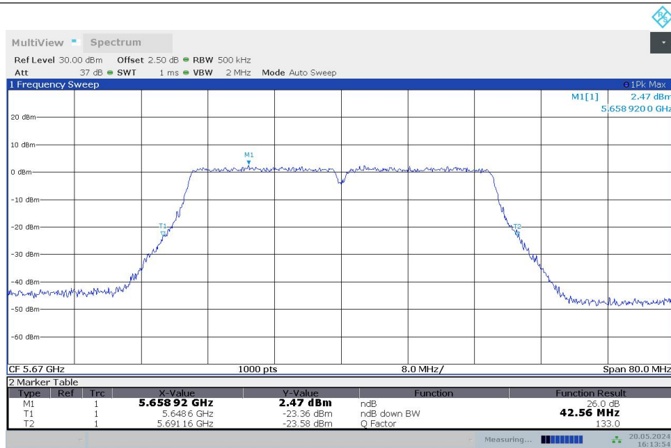
11N40MIMO_Ant1_5670
