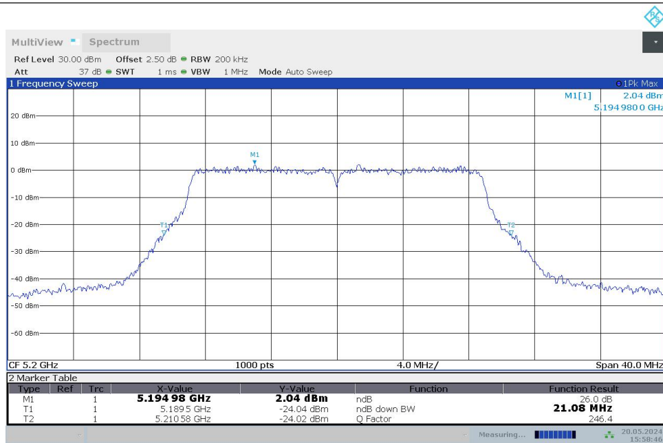
11AC20MIMO_Ant1_5200
