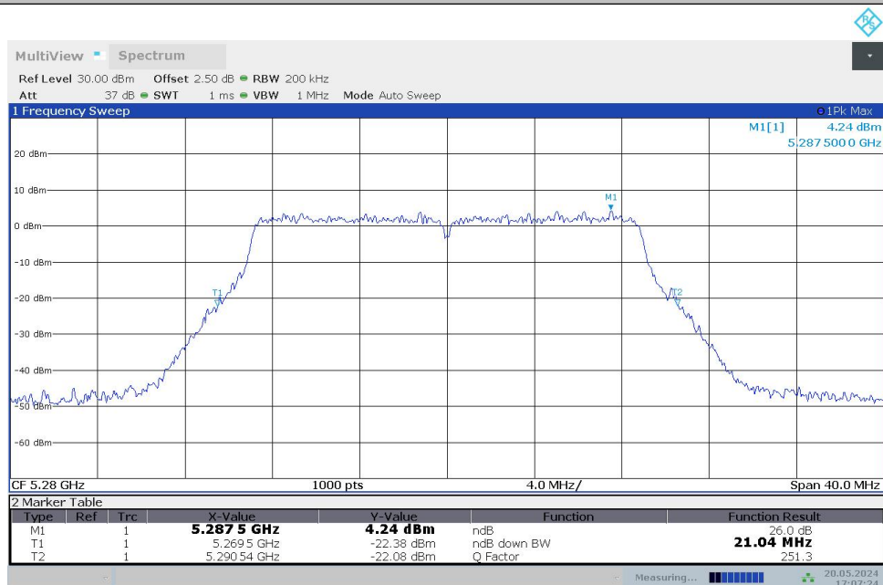
11AC20MIMO_Ant1_5280
