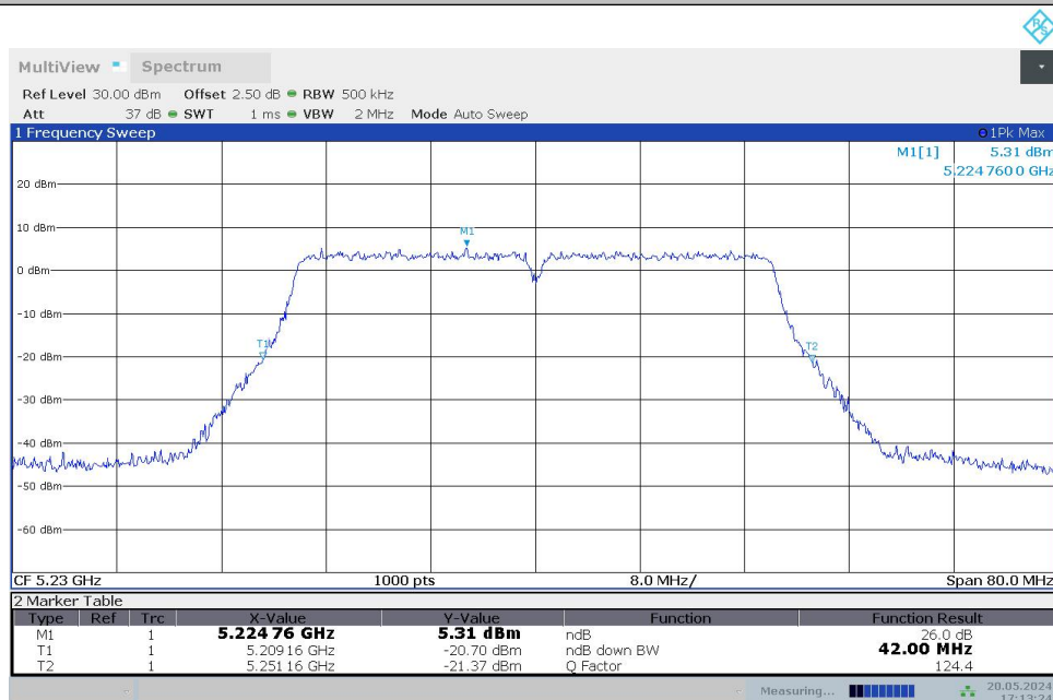
11N40MIMO_Ant1_5230
