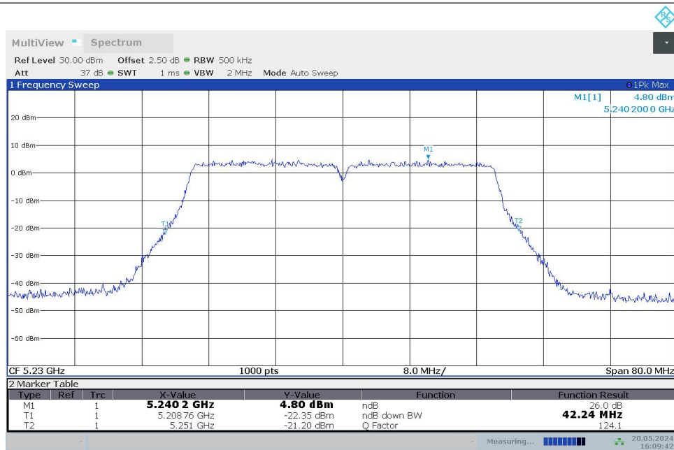
11N40MIMO_Ant1_5230
