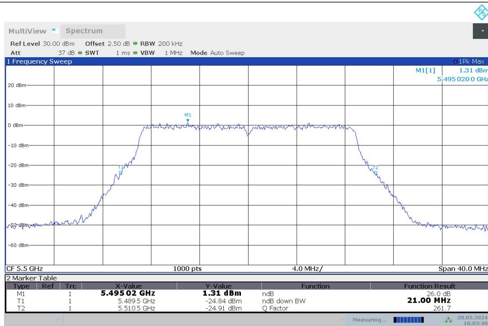
11AC20MIMO_Ant1_5500
