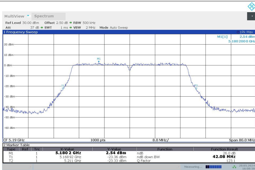
11N40MIMO_Ant1_5190
