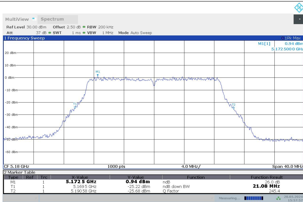
11AC20MIMO_Ant1_5180
