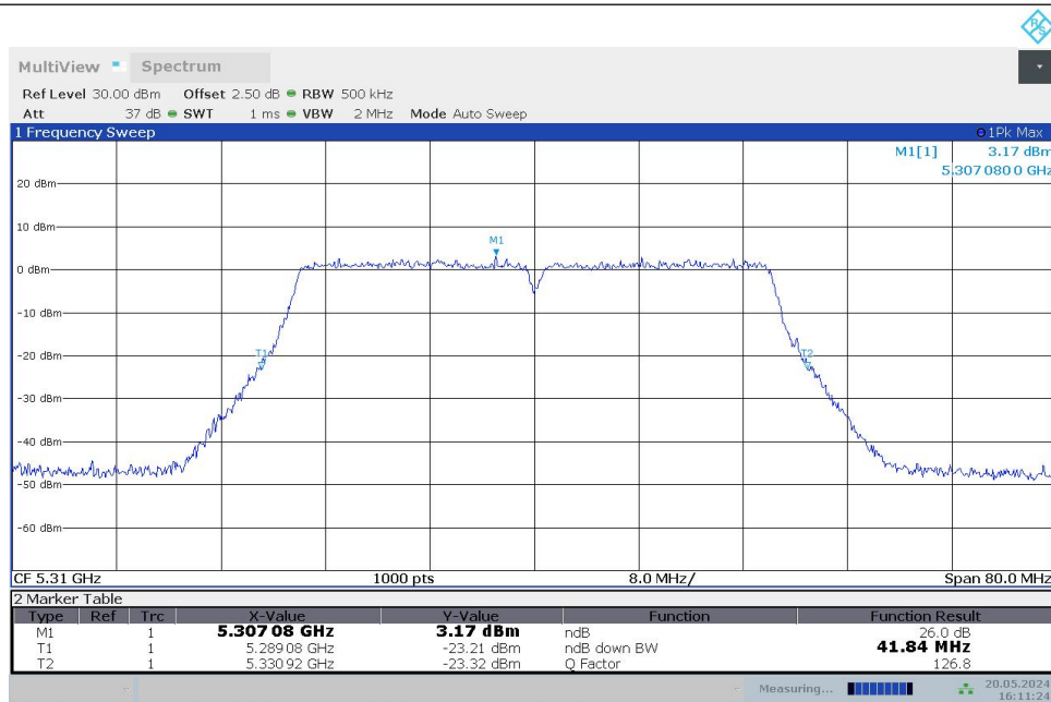
11N40MIMO_Ant1_5310
