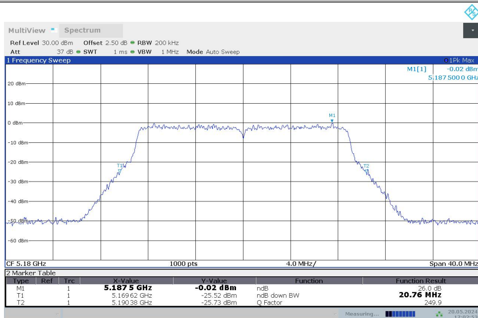
11AC20MIMO_Ant1_5180
