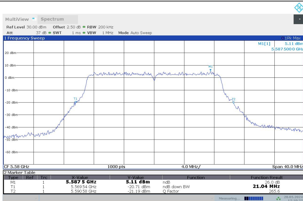
11AC20MIMO_Ant1_5580
