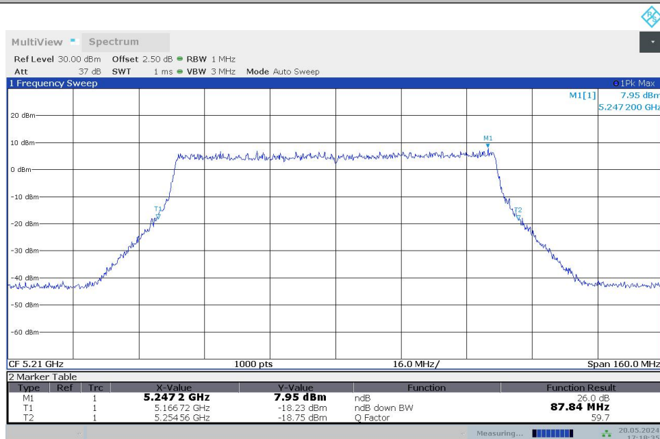
11BE80MIMO_Ant1_5210
