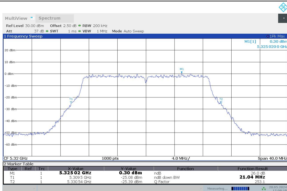
11AC20MIMO_Ant1_5320
