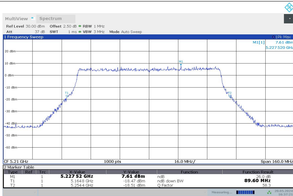
11BE80MIMO_Ant1_5210
