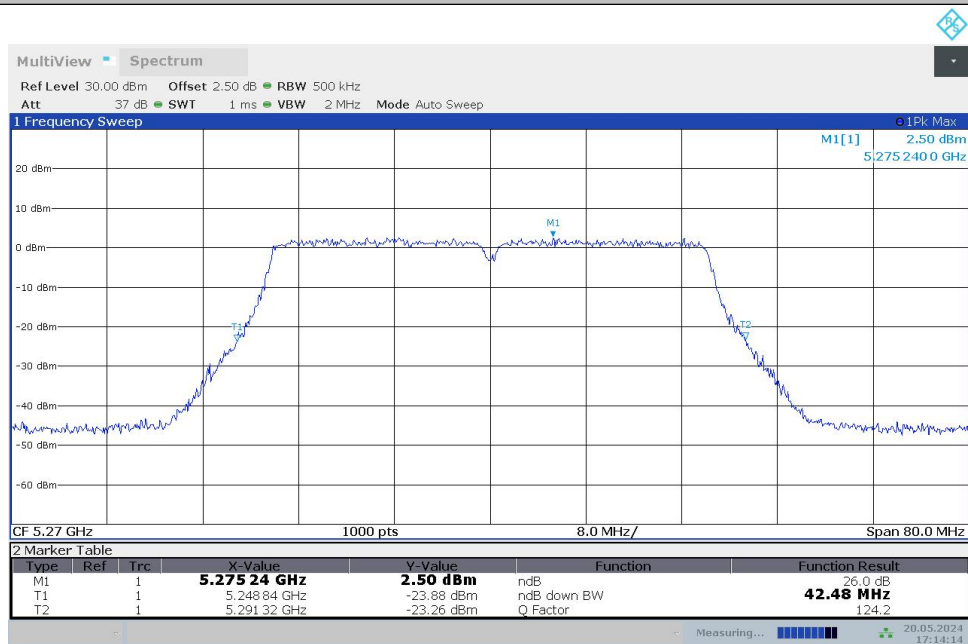
11N40MIMO_Ant1_5270
