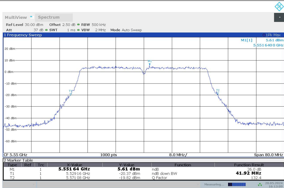
11N40MIMO_Ant1_5550
