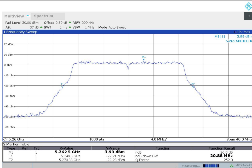
11AC20MIMO_Ant1_5260
