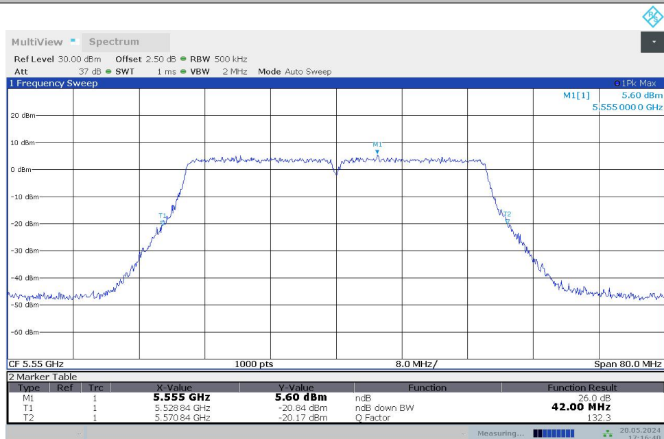
11N40MIMO_Ant1_5550
