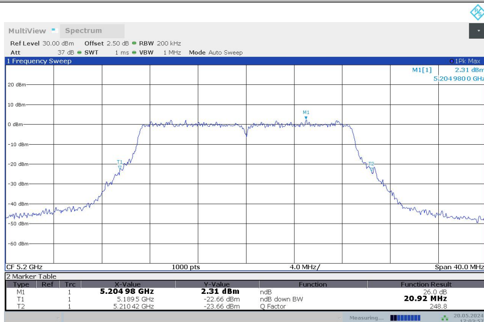
11AC20MIMO_Ant1_5200
