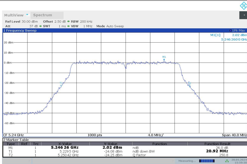
11AC20MIMO_Ant1_5240
