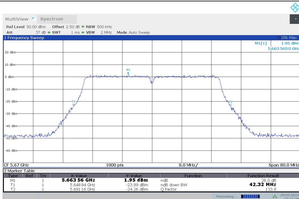
11N40MIMO_Ant1_5670
