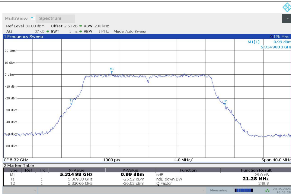
11AC20MIMO_Ant1_5320
