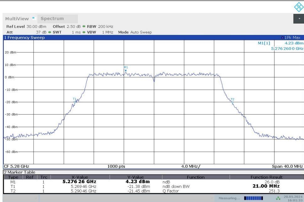
11AC20MIMO_Ant1_5280
