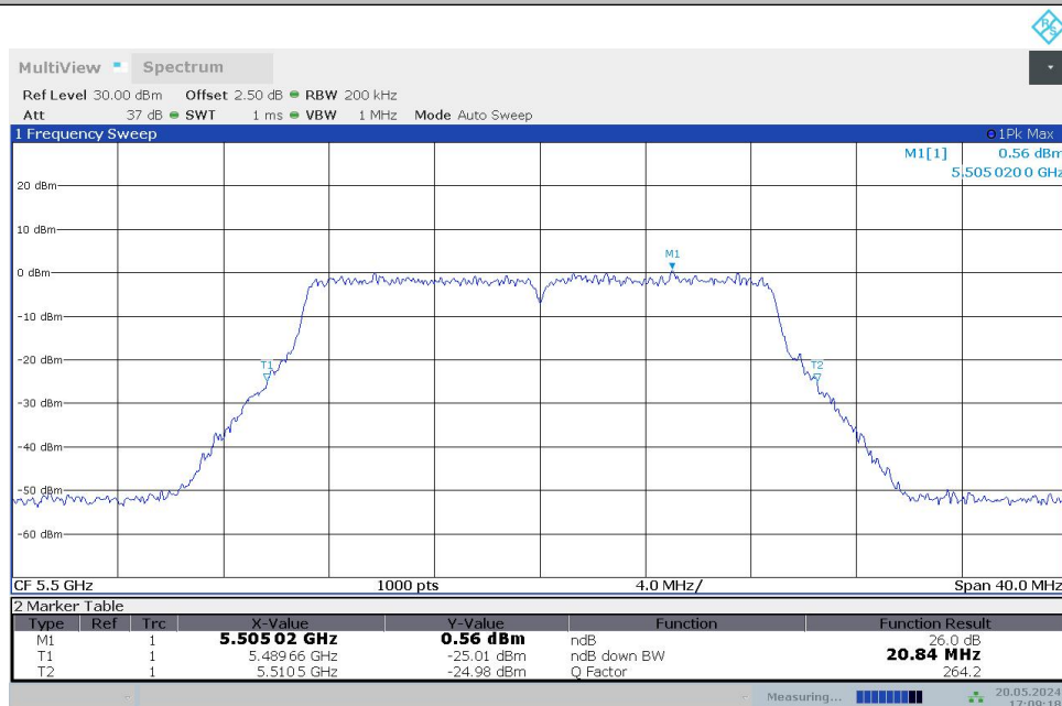
11AC20MIMO_Ant1_5500
