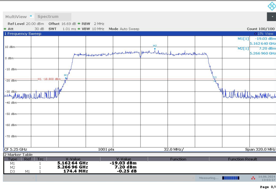
11AX160MIMO_Ant1_5250
