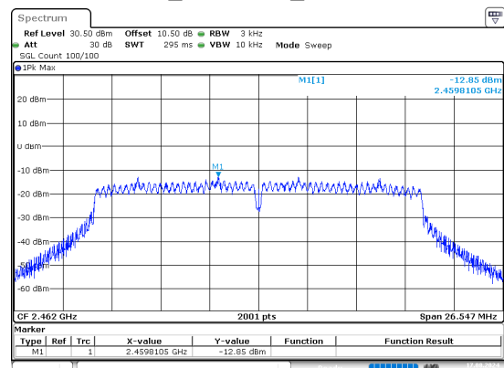
n20_2462MHz_Chain 1
