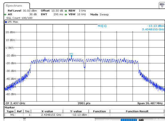
n20_2437MHz_Chain 1
