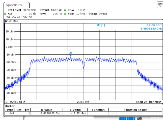
n20_2412MHz_Chain 1
