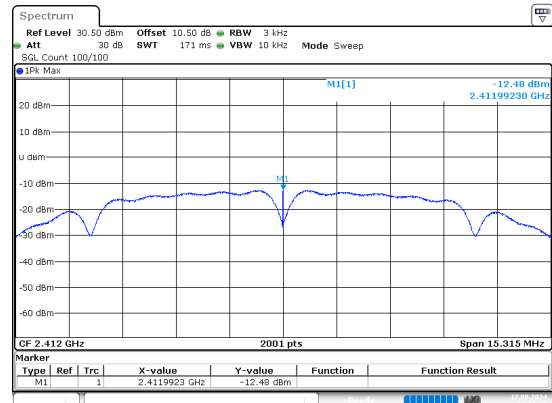
b_2412MHz_Chain 1
