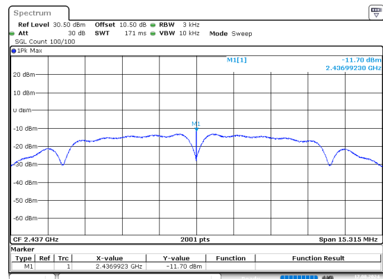
b_2437MHz_Chain 1
