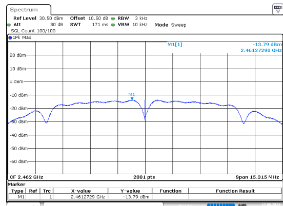
b_2462MHz_Chain 1
