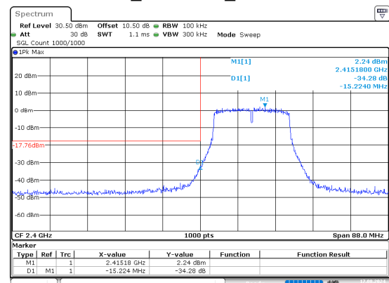
n20_2412MHz_Chain 1
