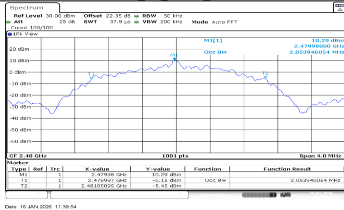
BLE 2M Ant BT 2480
