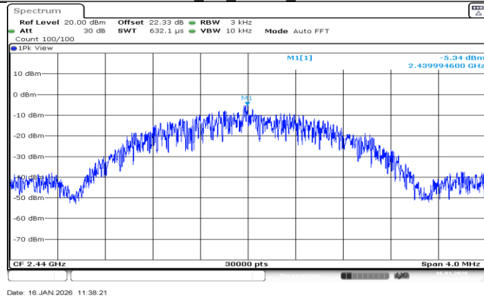
BLE 2M Ant BT 2440
