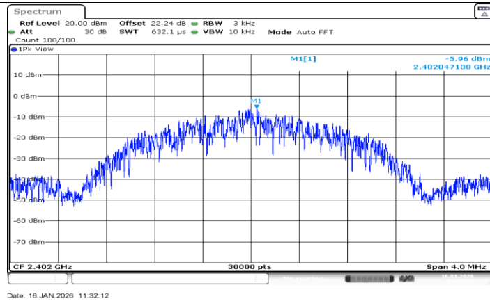
BLE 2M Ant BT 2402
