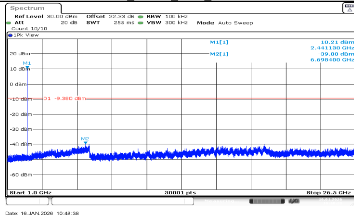
DH5 Ant BT 2441_1000~26500
