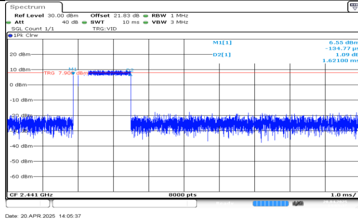
3DH3_Ant BT_Hop
