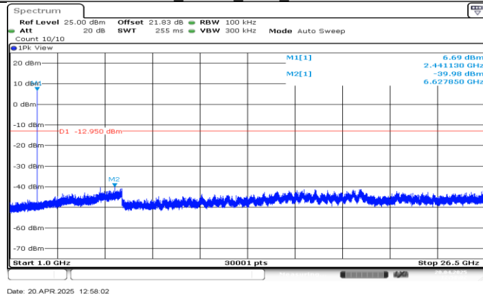
DH5_Ant BT_2441_1000~26500
