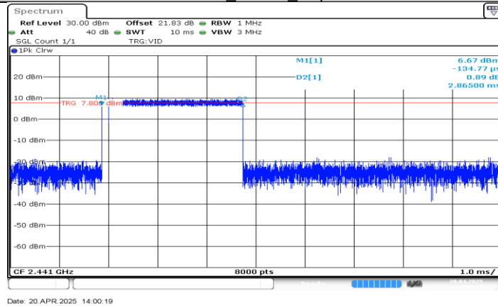
3DH5_Ant BT_Hop
