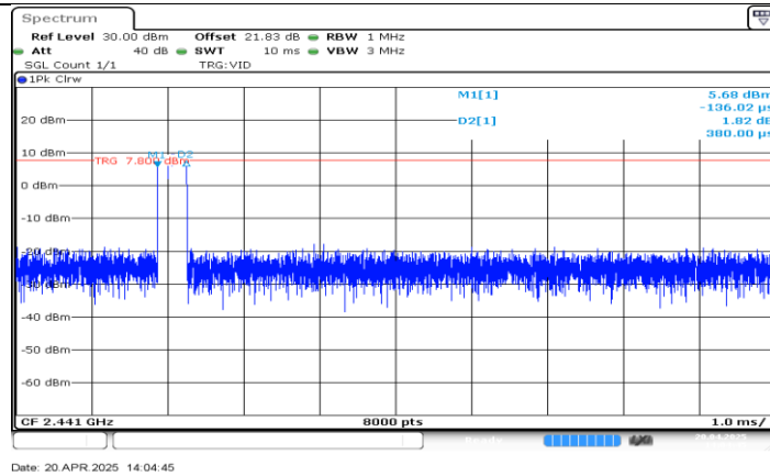
3DH1_Ant BT_Hop
