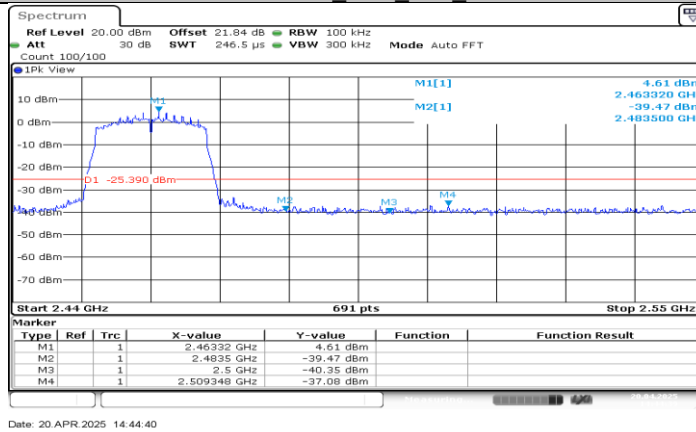
11N20MIMO_Ant0_High_2462
