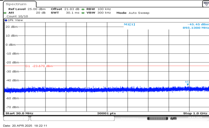
11B_Ant0_2437_30-1000
