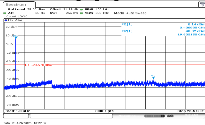
11B_Ant0_2437_1000-26500
