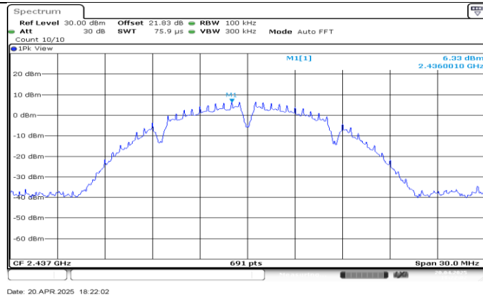
11B_Ant0_2437_0-Reference
