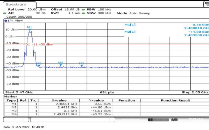
BLE 2M Ant1 High 2480
