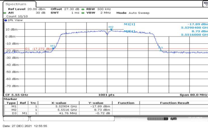
11N40MIMO Ant1 5550
