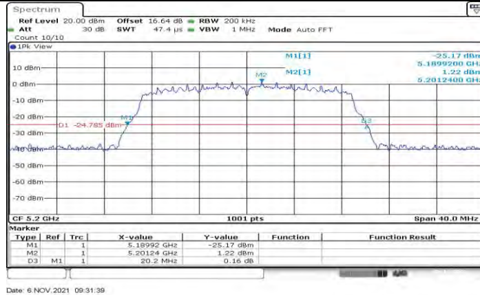
11N20MIMO Ant2 5200
