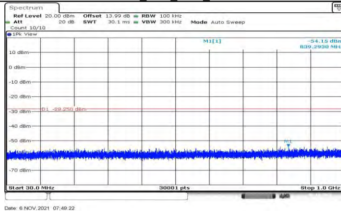
11N40MIMO_Ant1_2422_30~1000
