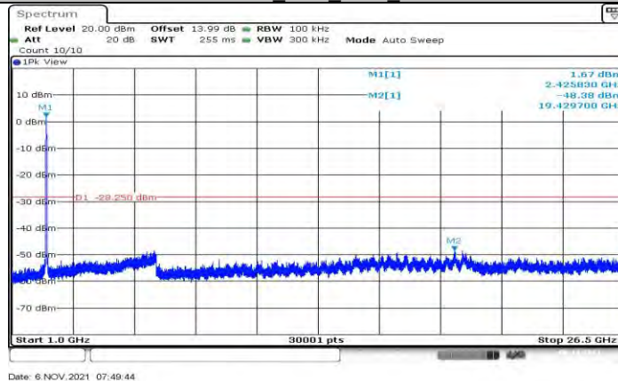
11N40MIMO_Ant1_2422_1000~26500
