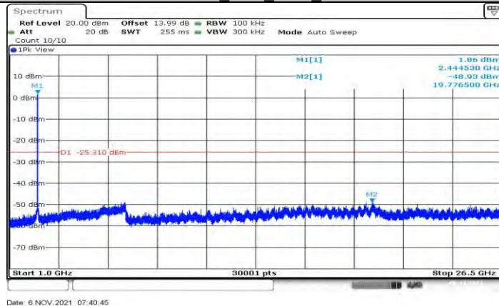
11N20MIMO_Ant1_2437_1000~26500
