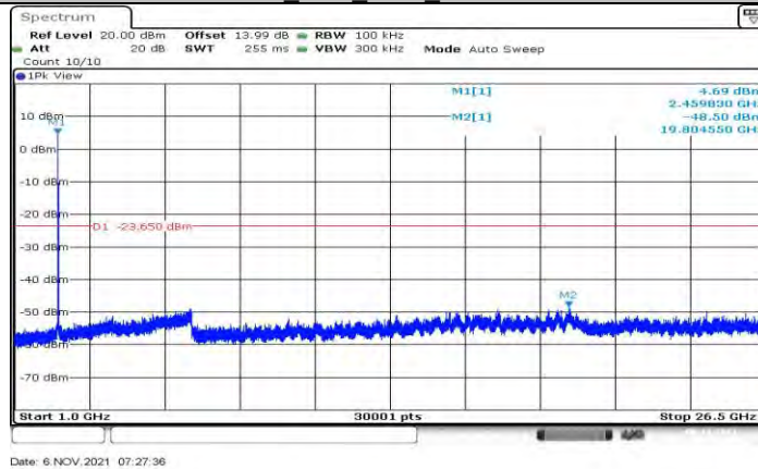
11B_Ant1_2462_1000~26500
