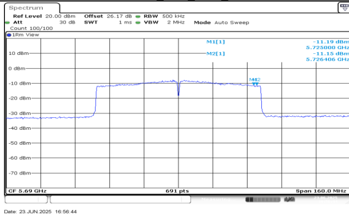
11AC80SISO_Ant0_5690_UNII-3
