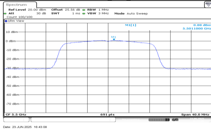
11N20SISO_Ant0_5500
