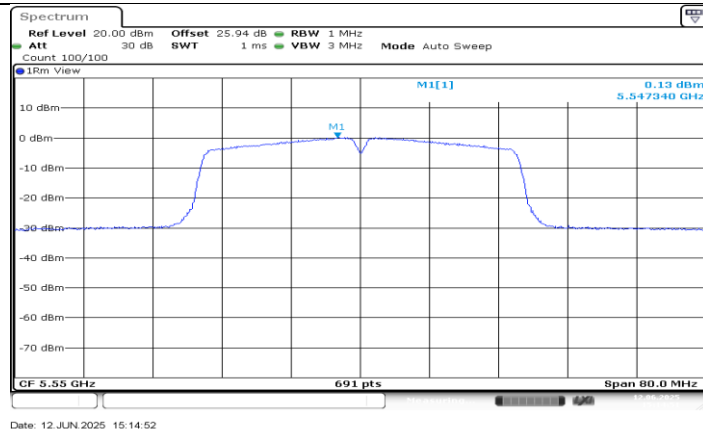
11N40SISO_Ant0_5550
