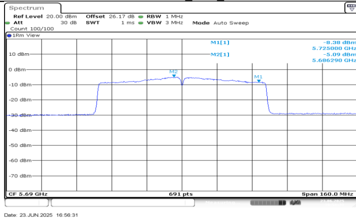
11AC80SISO_Ant0_5690_UNII-2C
