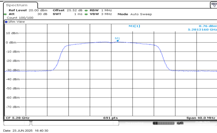
11N20SISO_Ant0_5280
