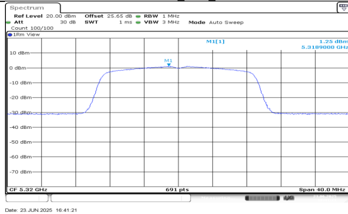
11N20SISO_Ant0_5320
