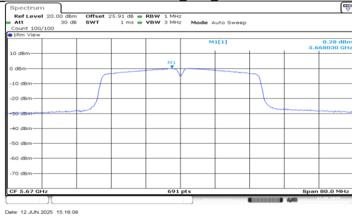
11N40SISO_Ant0_5670
