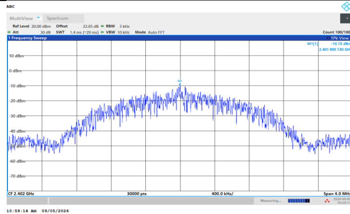
BLE_2M_Ant1_2402
