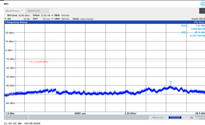
BLE_2M_Ant1_2402_1000~26500
