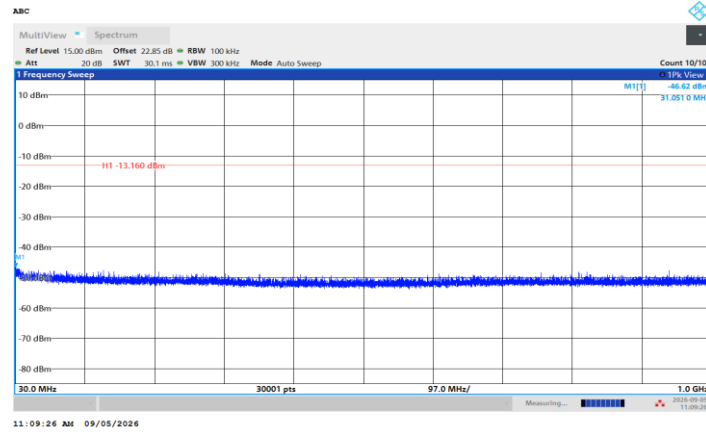
BLE_2M_Ant1_2480_30~1000
