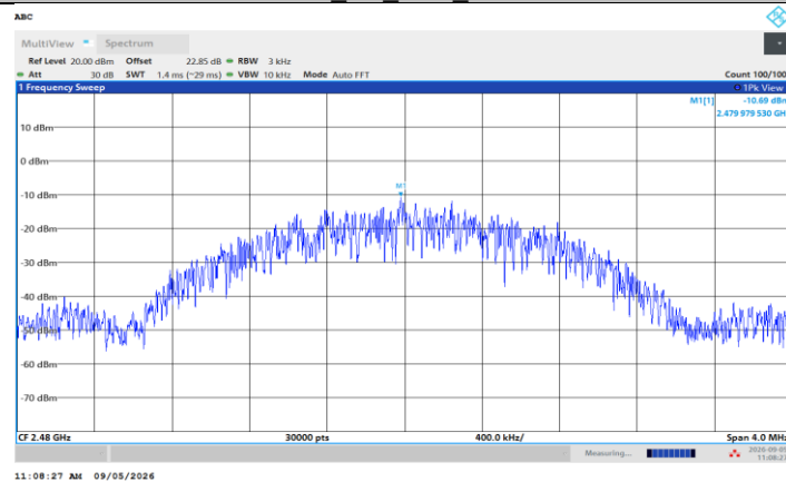
BLE_2M_Ant1_2480
