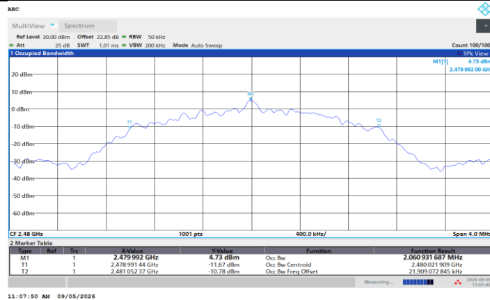
BLE_2M_Ant1_2480
