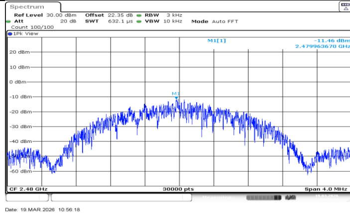
BLE_2M_Ant1_2480
