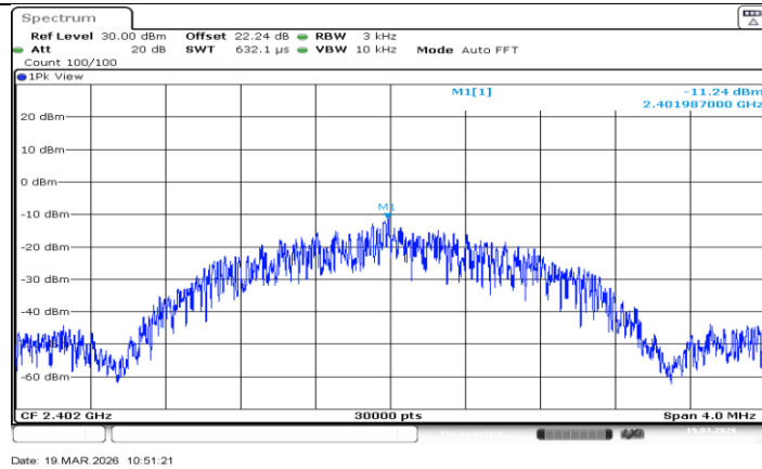
BLE_2M_Ant1_2402
