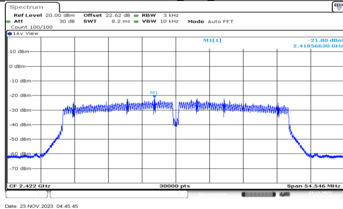
11N40MIMO_Ant2_2422
