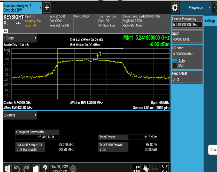
11A_Ant1_5240
