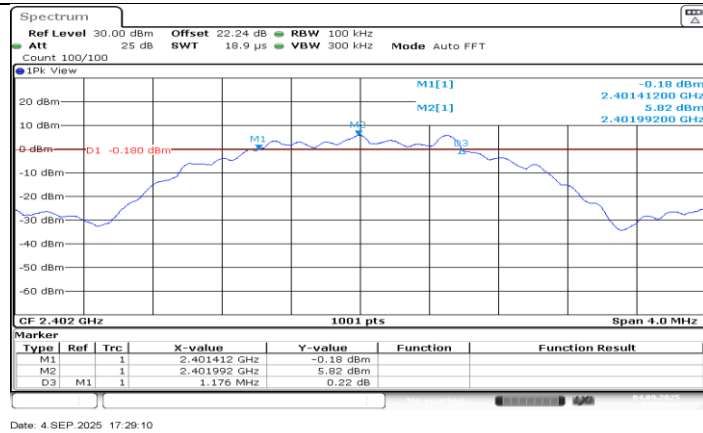
BLE 2M Ant3 2402
