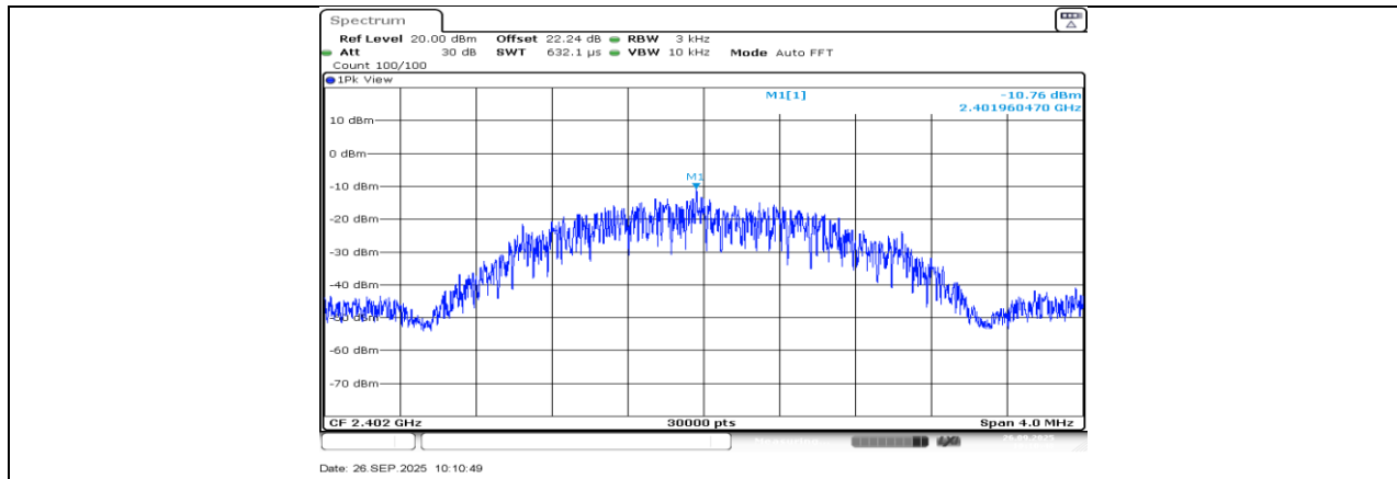
BLE 2M Ant3 2402
