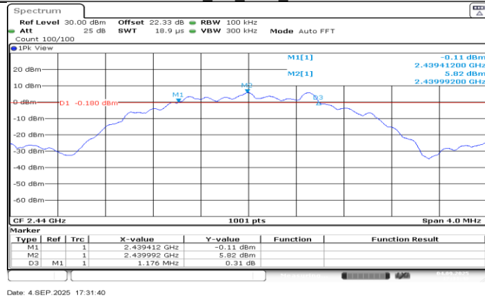
BLE 2M Ant3 2440
