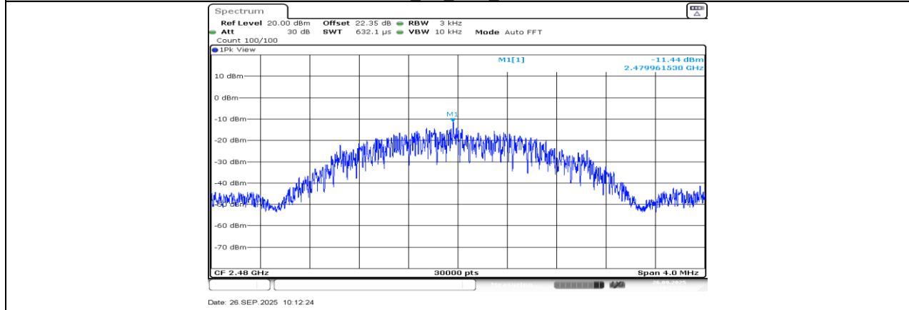
BLE 2M Ant3 2480
