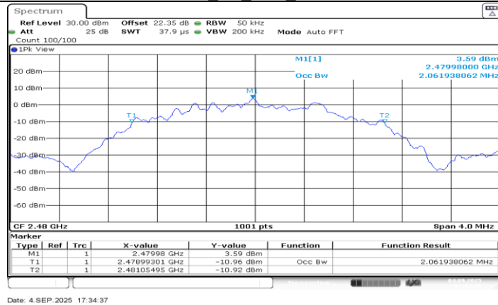
BLE 2M Ant3 2480
