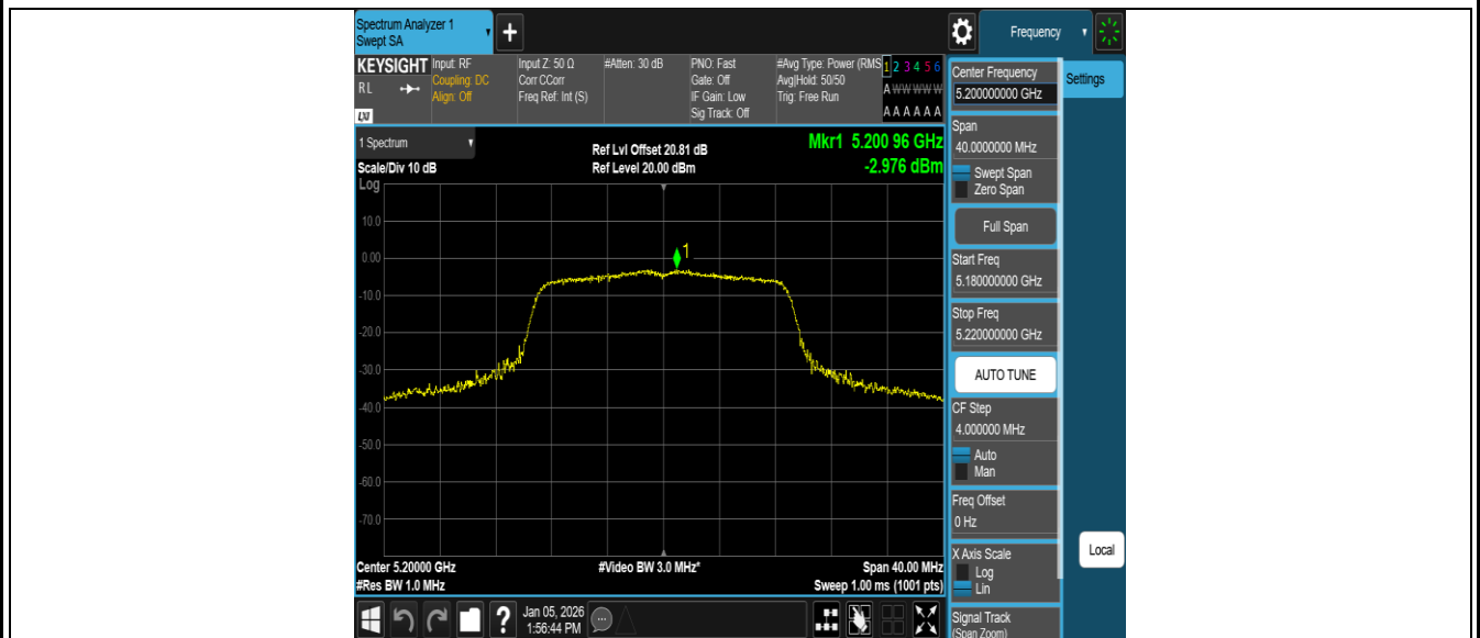
11N20MIMO Ant2 5200
