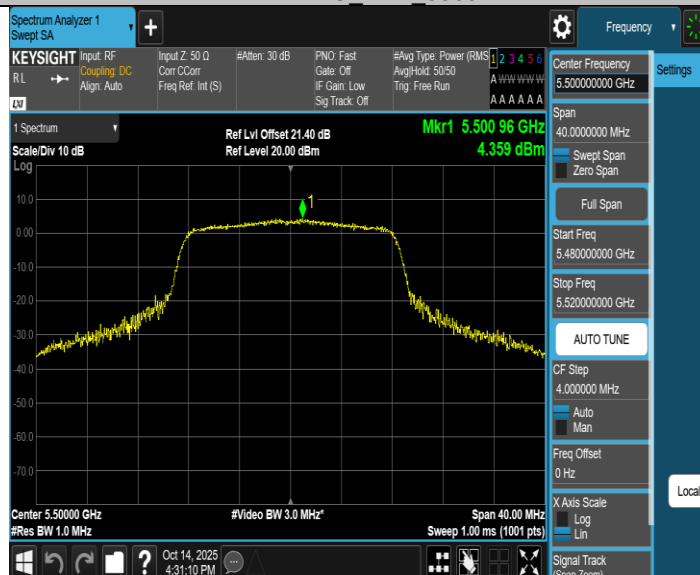
11A-SISO_Ant2_5500
