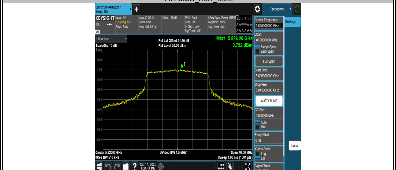
11A-SISO_Ant2_5825
