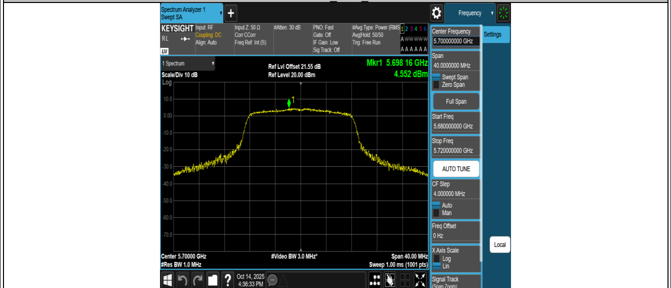
11A-SISO_Ant2_5700
