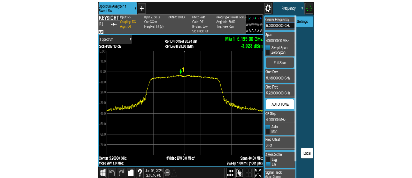
11AC20MIMO_Ant1_5200
