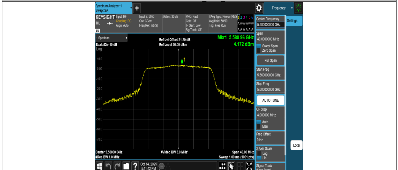
11AC20MIMO_Ant2_5580
