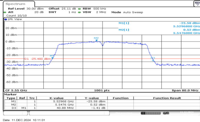
11N40MIMO_Ant1_5550
