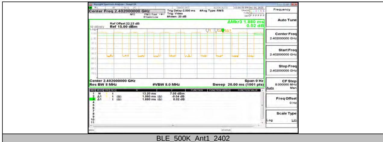
BLE_500K_Ant1_2402
