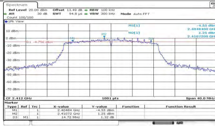
11N20MIMO_Ant1_2412
