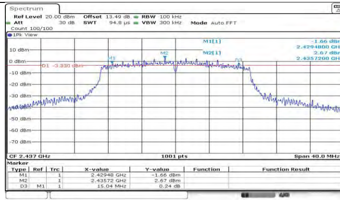
11N20MIMO Ant2 2437
