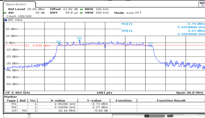
11AX20MIMO_Ant1_2462
