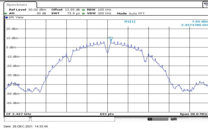
11B_Ant2_2437_0-Reference
