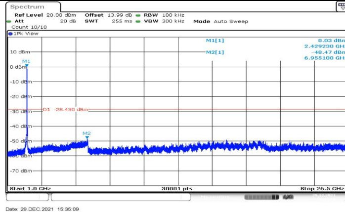
11AX40MIMO Ant1 2437 1000~26500
