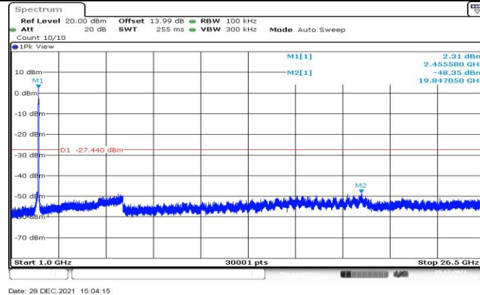
11N40MIMO Ant1 2452 1000-26500
