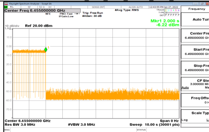
11AX20MIMO Ant1 6455 Center 6455 9
