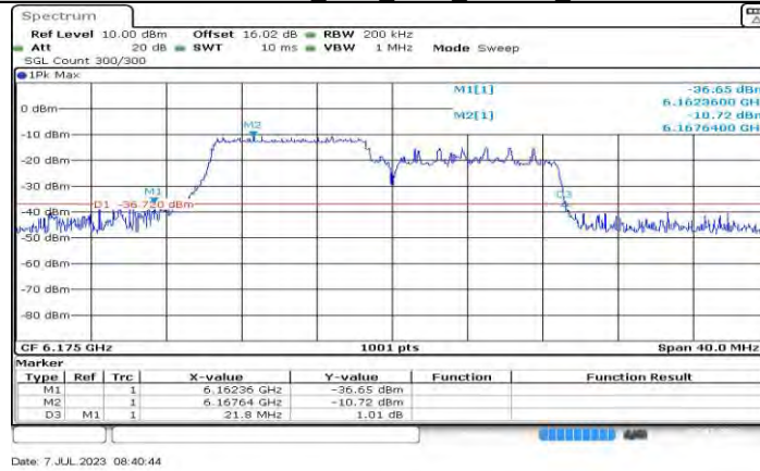
11AX20MIMO Ant1 6175 106Tone RU33
