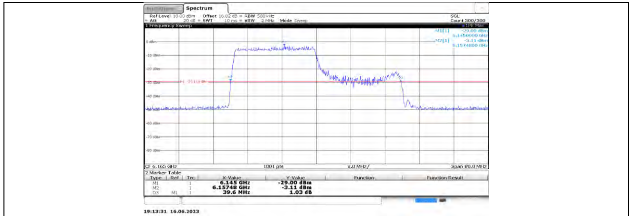
11AX40MIMO_Ant0_6165_242Tone_RU61
