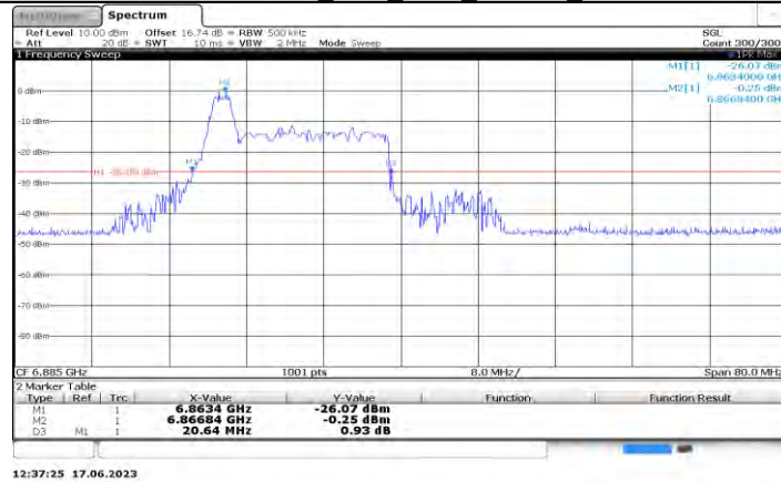
11AX40MIMO Ant0 6885 26Tone RU0
