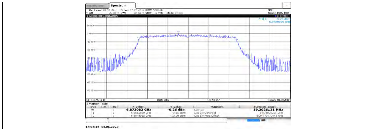
11AX20MIMO_Ant0_6875
