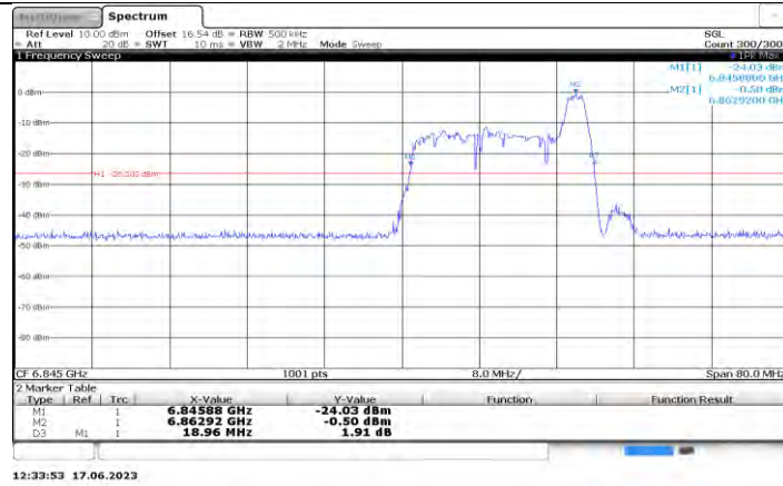
11AX40MIMO Ant1 6845 26Tone RU17
