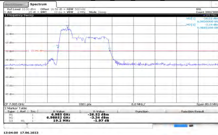
11AX40MIMO Ant0 7005 52Tone RU37
