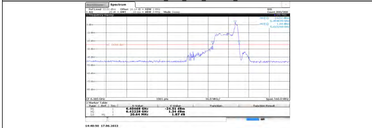
11AX80MIMO_Ant0_6385_26Tone_RU36
