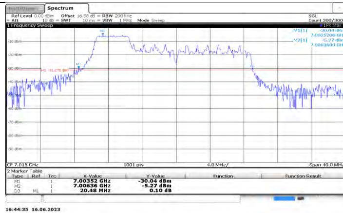
11AX20MIMO Ant0 7015 52Tone RU37
