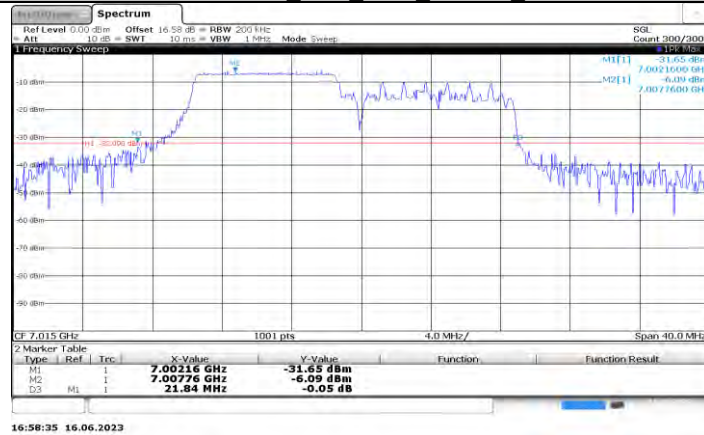
11AX20MIMO Ant0 7015 106Tone RU53
