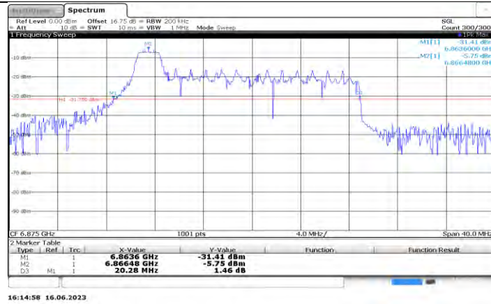
11AX20MIMO Ant0 6875 26Tone RU0
