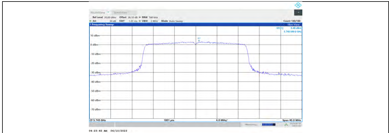
11AX20MIMO_Ant0_5745
