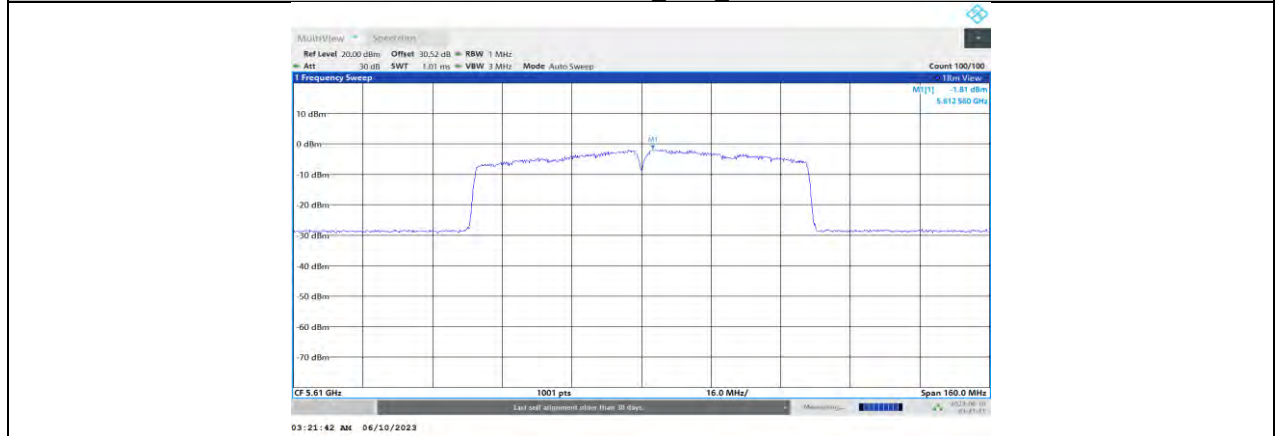
11AC80MIMO_Ant0_5610
