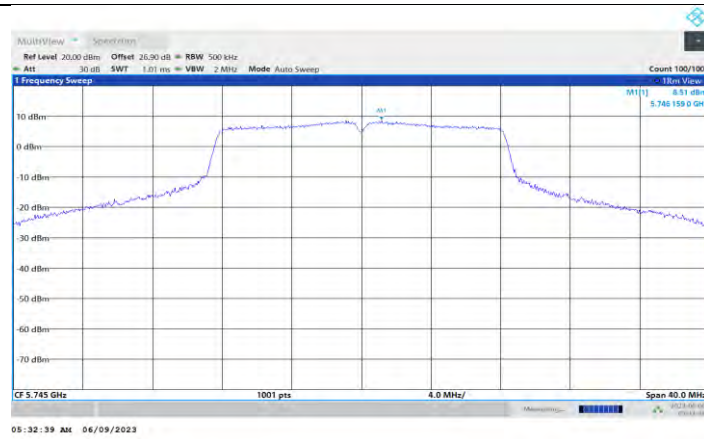
11A_Ant0_5745
