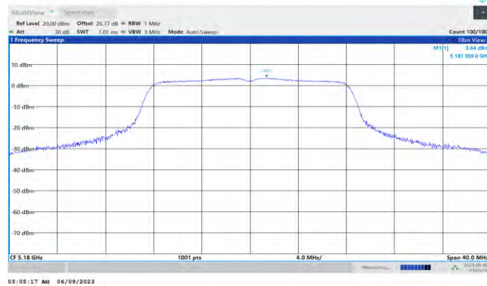
11A_Ant1_5180
