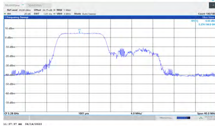
11AX20MIMO_Ant0_5280_106Tone_RU53
