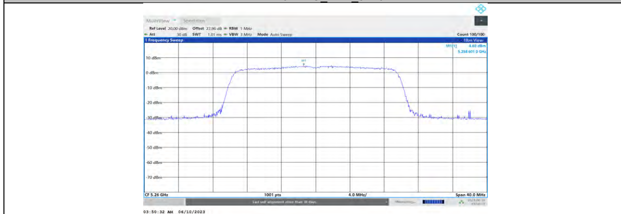
11AX20MIMO_Ant0_5260
