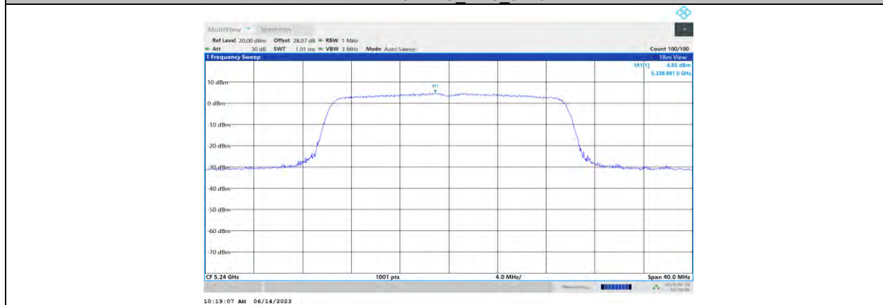
11AX20MIMO_Ant1_5240
