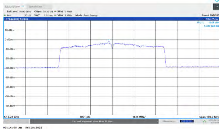
11AC80MIMO_Ant0_5210
