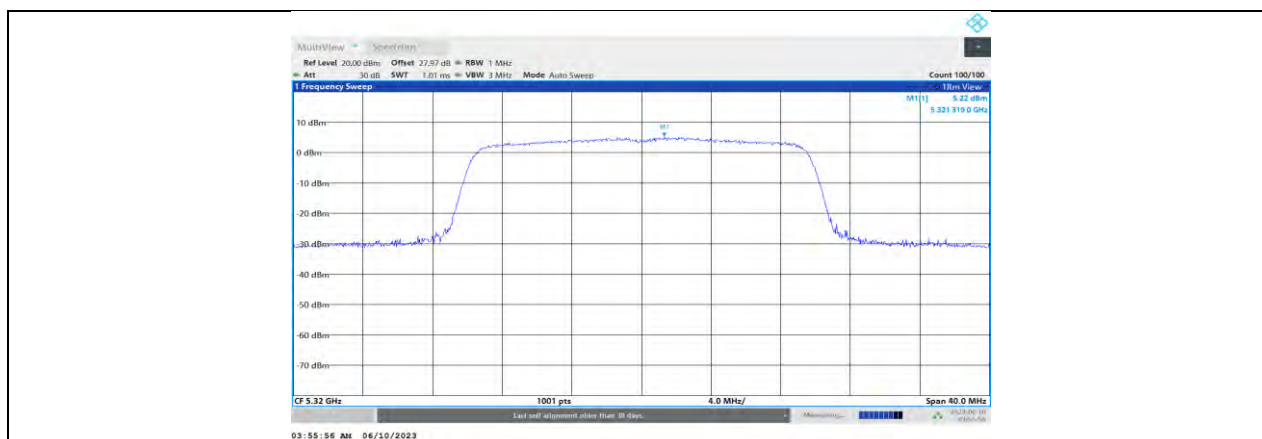
11AX20MIMO_Ant0_5320
