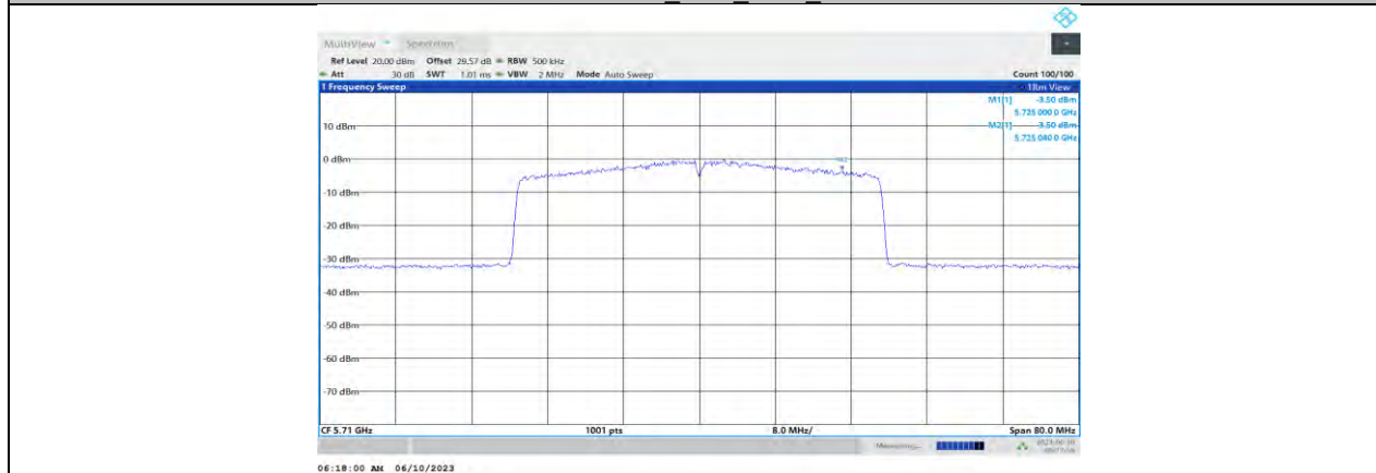
11AX40MIMO_Ant1_5710_UNII-3
