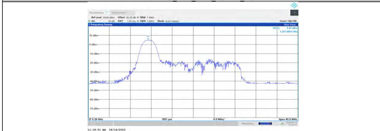
11AX20MIMO_Ant1_5260_26Tone_RU0
