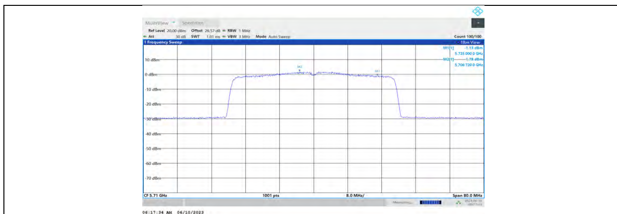
11AX40MIMO_Ant1_5710_UNII-2C
