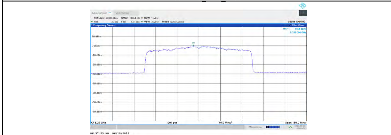
11AX80MIMO_Ant1_5290
