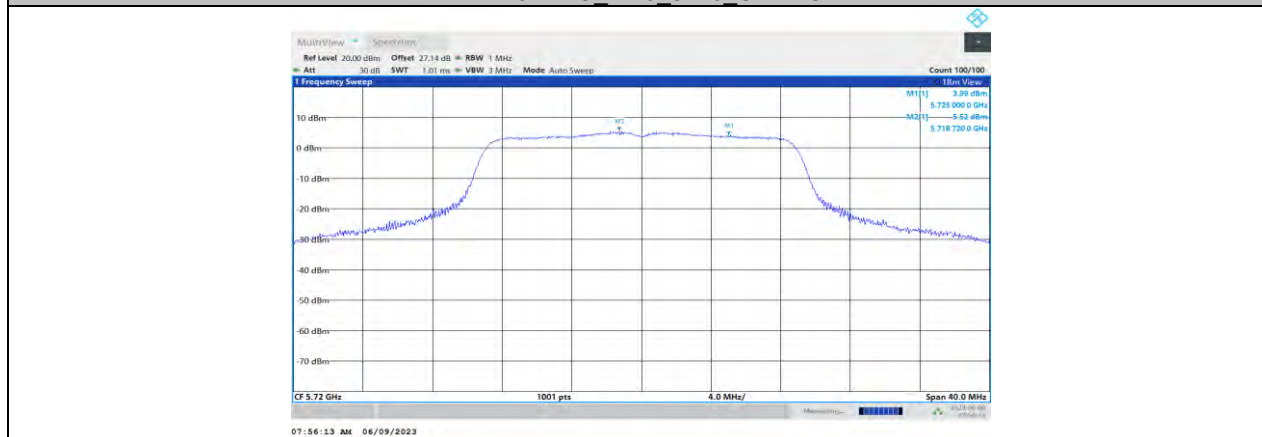
11N20MIMO_Ant1_5720_UNII-2C
