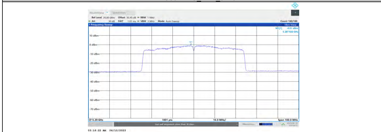
11AC80MIMO_Ant0_5290
