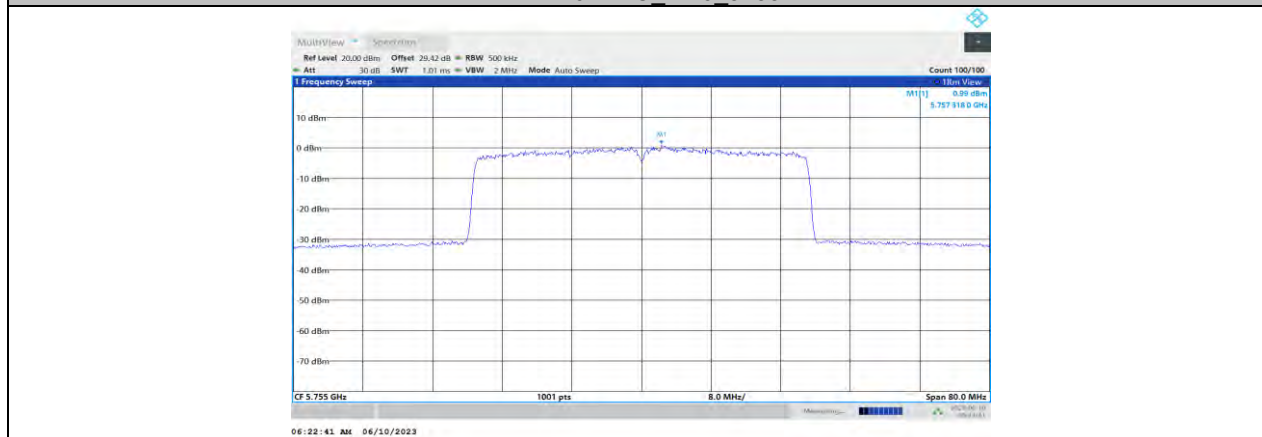
11AX40MIMO_Ant1_5755
