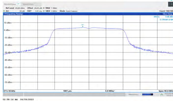
11A_Ant0_5180
