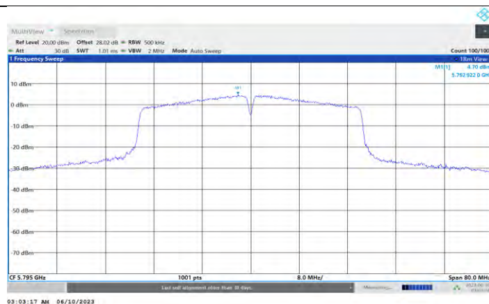
11N40MIMO_Ant0_5795
