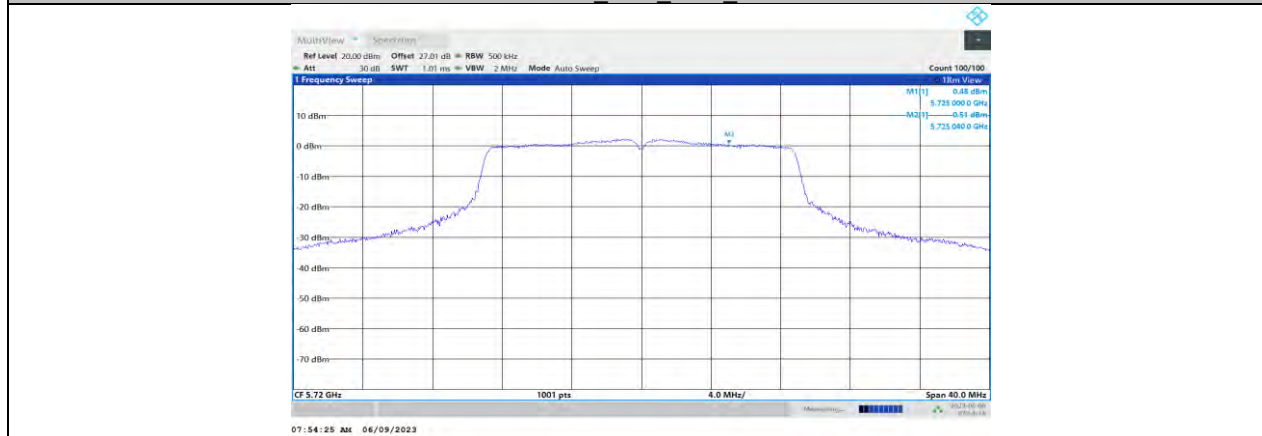
11N20MIMO_Ant0_5720_UNII-3
