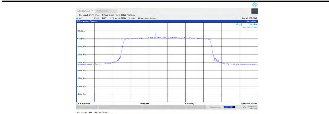
11AX20MIMO_Ant0_5825
