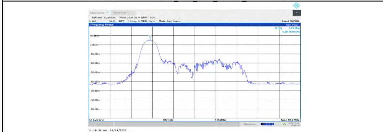
11AX20MIMO_Ant0_5260_26Tone_RU0
