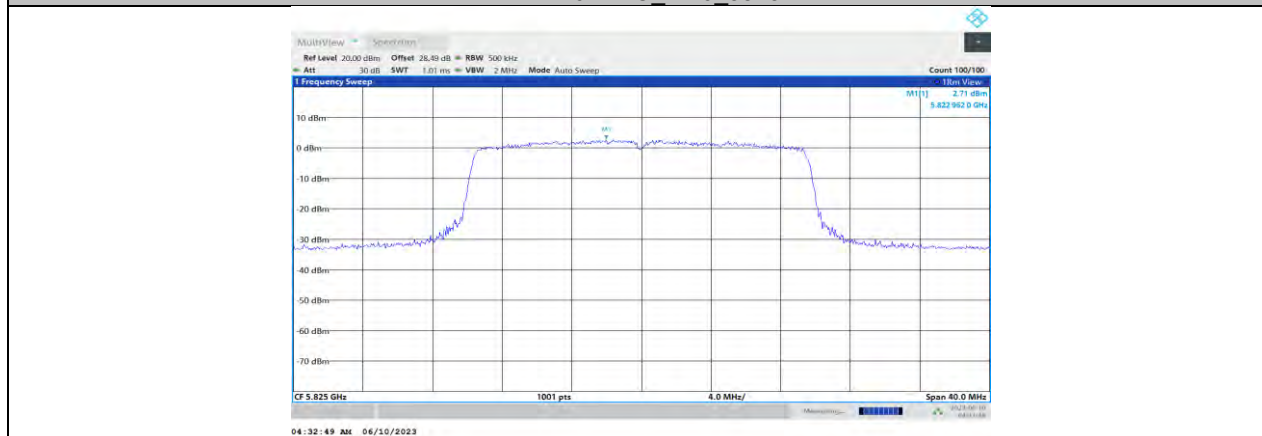
11AX20MIMO_Ant1_5825
