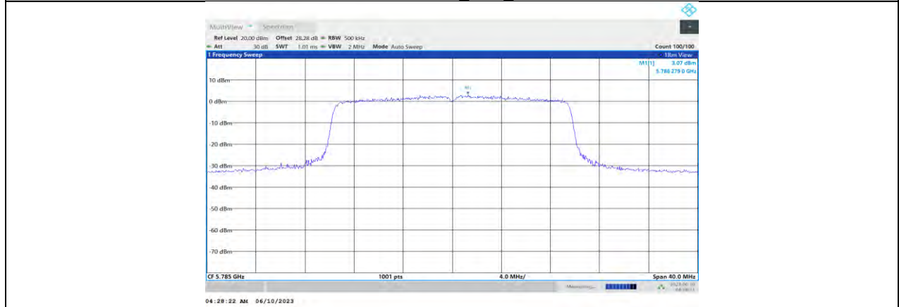
11AX20MIMO_Ant0_5785
