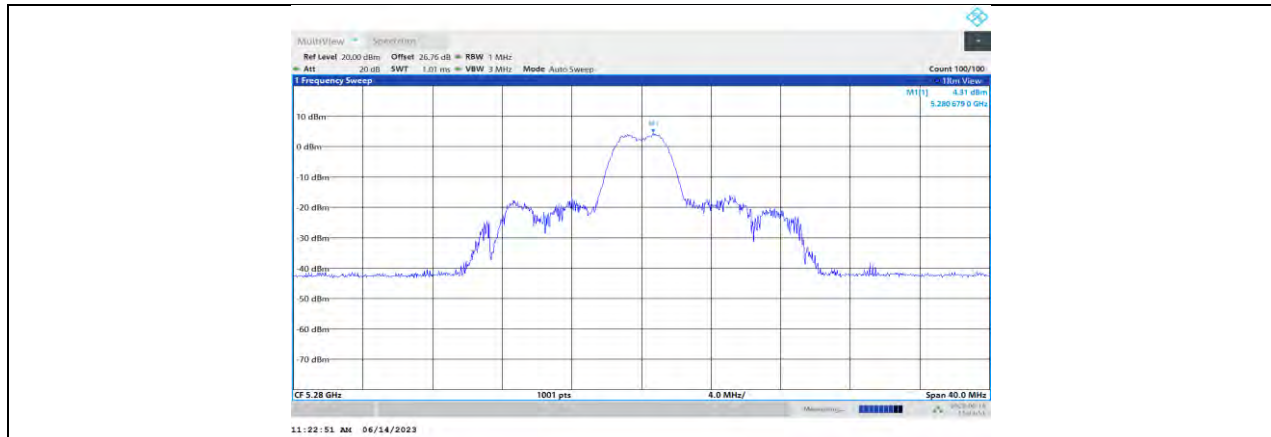
11AX20MIMO_Ant1_5280_26Tone_RU4
