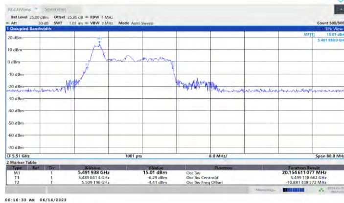
11AX40MIMO Ant1 5510 26Tone RU0
