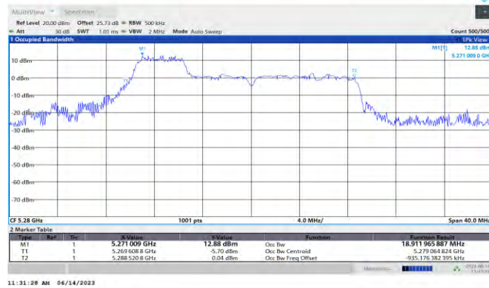
11AX20MIMO Ant0 5280 52Tone RU37
