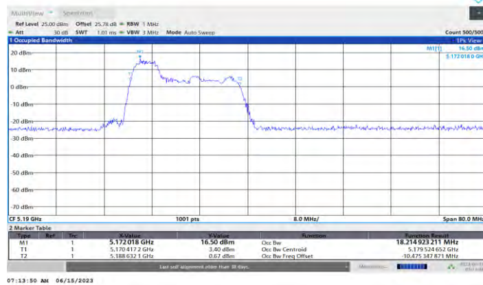
11AX40MIMO Ant1 5190 52Tone RU37
