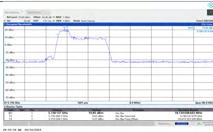
11AX40MIMO Ant1 5755 52Tone RU37
