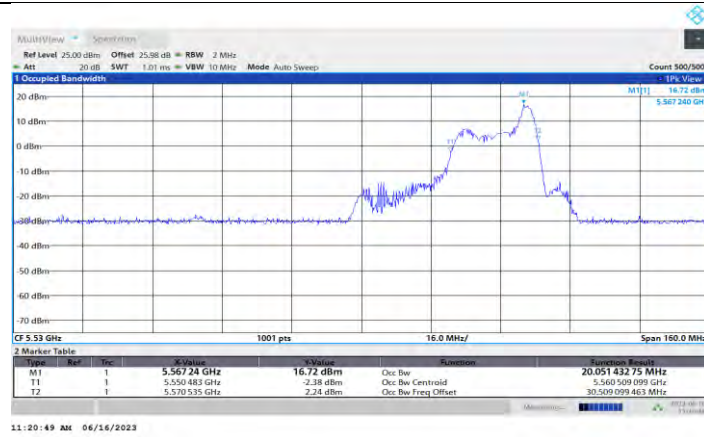
11AX80MIMO_Ant1_5530_26Tone_RU36
