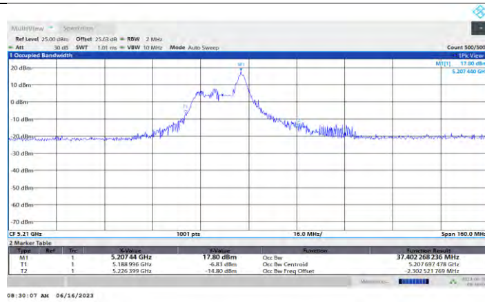
11AX80MIMO_Ant0_5210_26Tone_RU17
