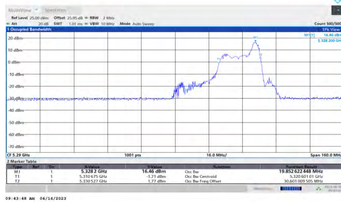
11AX80MIMO_Ant1_5290_26Tone_RU36
