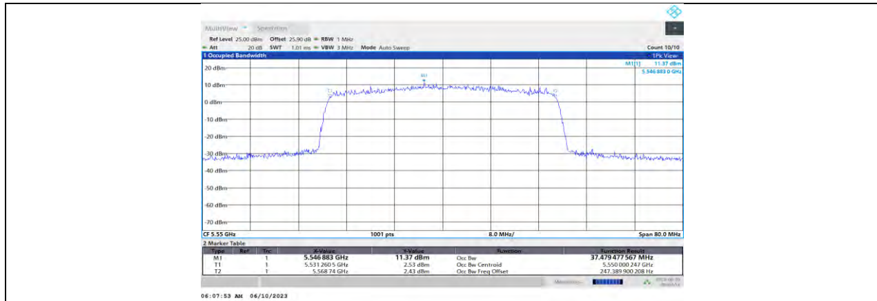
11AX40MIMO_Ant0_5550
