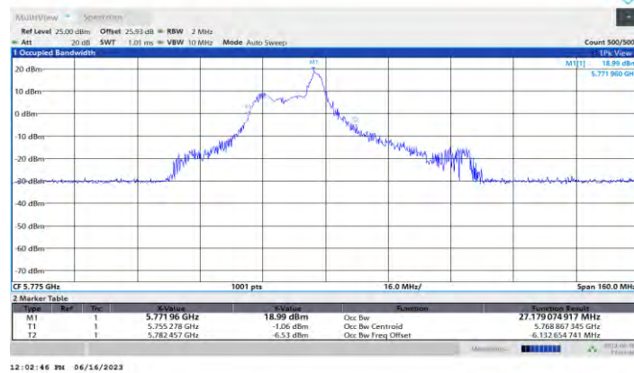
11AX80MIMO_Ant0_5775_26Tone_RU17
