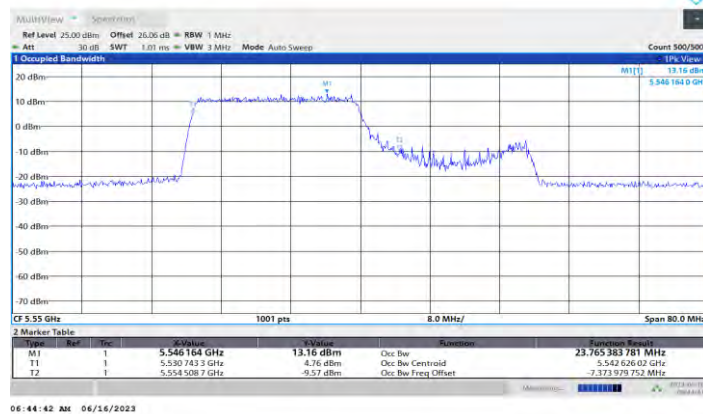
11AX40MIMO Ant1 5550 242Tone RU61
