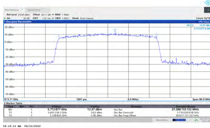
11AX40MIMO_Ant1_5710
