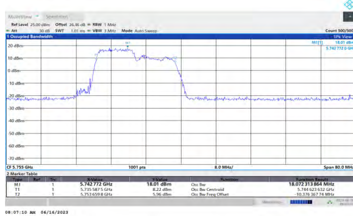
11AX40MIMO Ant1 5755 106Tone RU53
