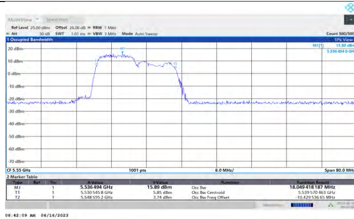
11AX40MIMO Ant1 5550 106Tone RU53
