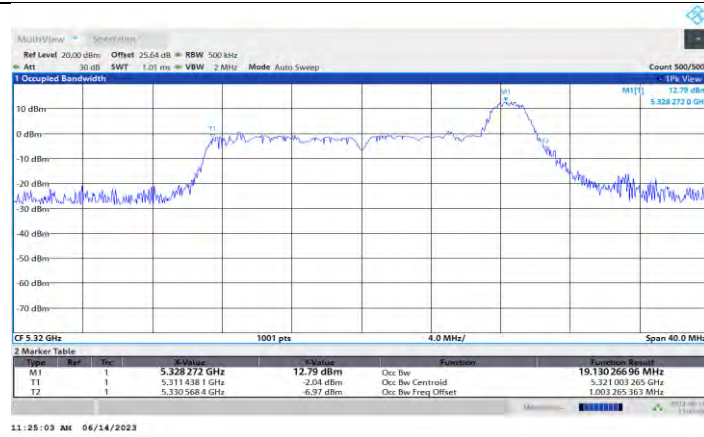
11AX20MIMO Ant0 5320 26Tone RU8
