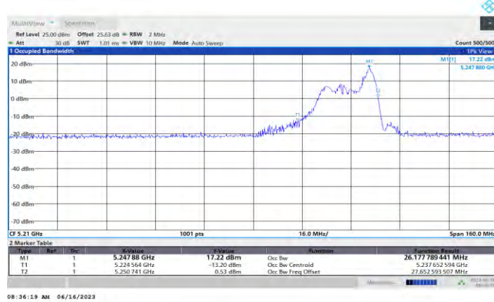
11AX80MIMO_Ant0_5210_26Tone_RU36
