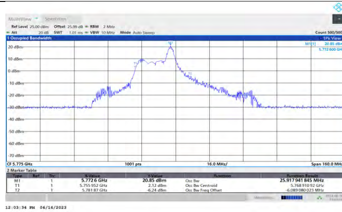
11AX80MIMO_Ant1_5775_26Tone_RU17
