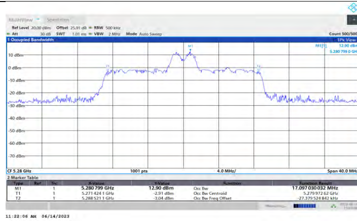
11AX20MIMO Ant1 5280 26Tone RU4
