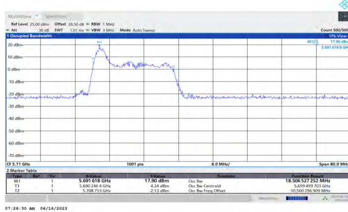
11AX40MIMO Ant0 5710 26Tone RU0
