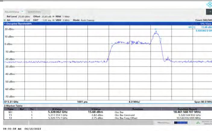
11AX40MIMO Ant1 5310 26Tone RU17
