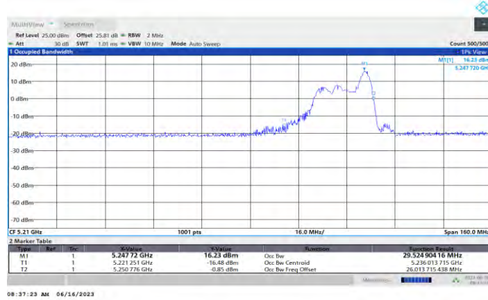
11AX80MIMO_Ant1_5210_26Tone_RU36
