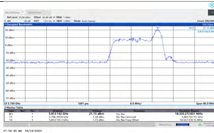
11AX40MIMO_Ant0_5795_26Tone_RU17
