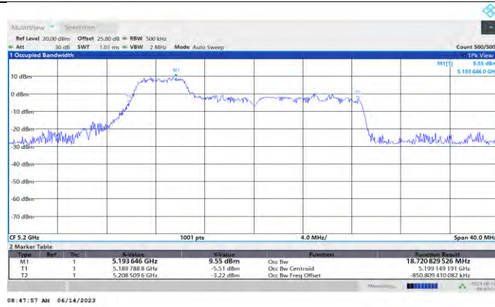
11AX20MIMO Ant1 5200 52Tone RU37
