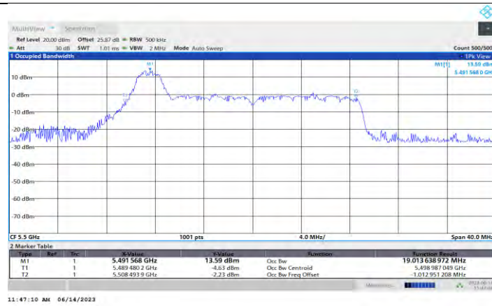
11AX20MIMO Ant1 5500 26Tone RU0
