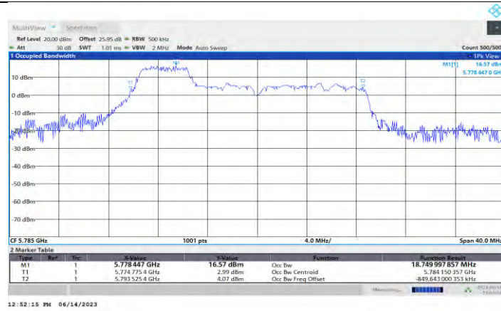
11AX20MIMO Ant0 5785 52Tone RU37
