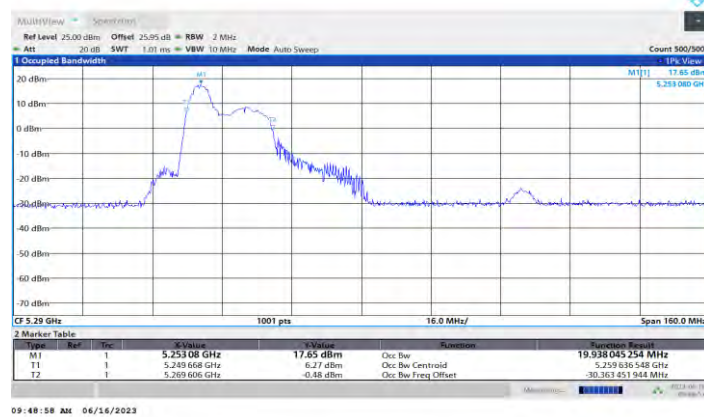
11AX80MIMO_Ant1_5290_52Tone_RU37
