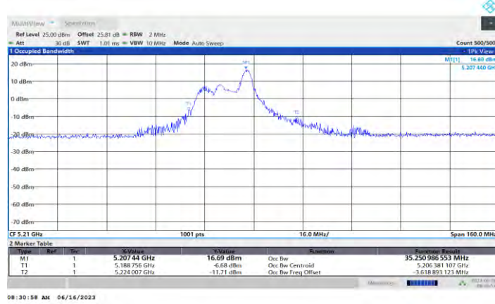
11AX80MIMO_Ant1_5210_26Tone_RU17
