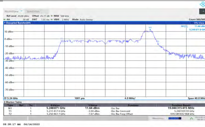
11AX20MIMO Ant1 5240 26Tone RU8
