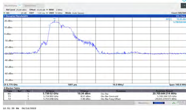
11AX80MIMO_Ant0_5775_106Tone_RU53
