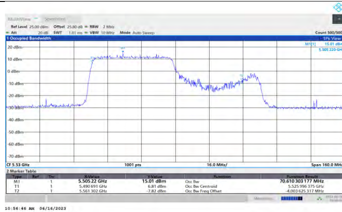
11AX80MIMO_Ant0_5530_484Tone_RU65
