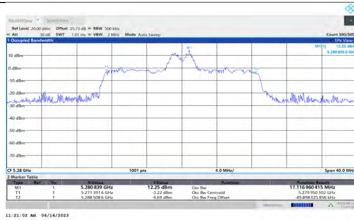
11AX20MIMO Ant0 5280 26Tone RU4
