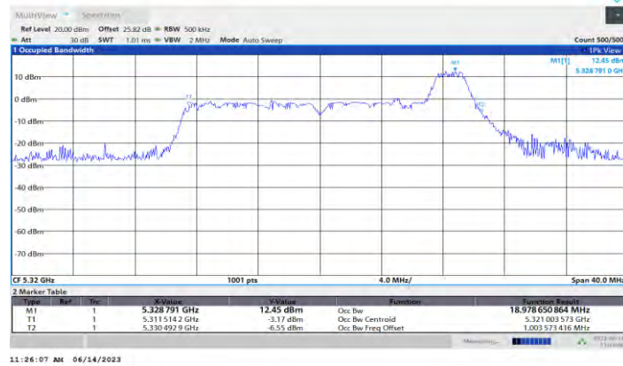
11AX20MIMO Ant1 5320 26Tone RU8
