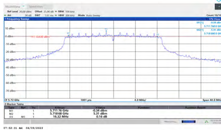
11N20MIMO_Ant0_5720
