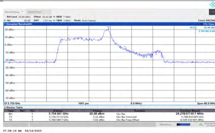
11AX40MIMO Ant0 5755 26Tone RU8
