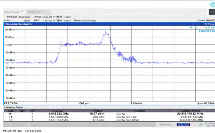
11AX40MIMO Ant0 5550 26Tone RU8
