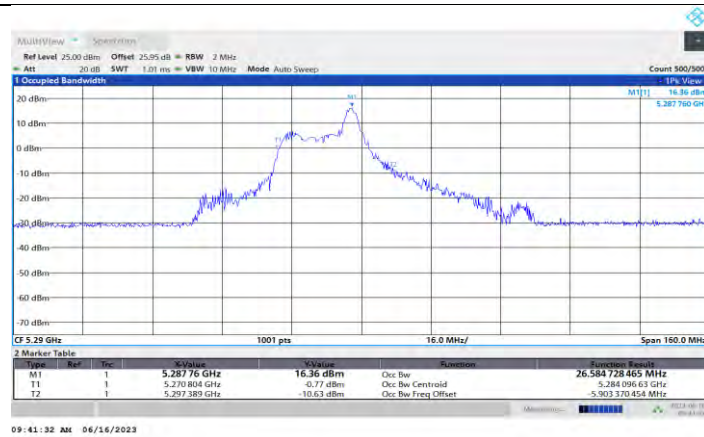
11AX80MIMO_Ant1_5290_26Tone_RU17
