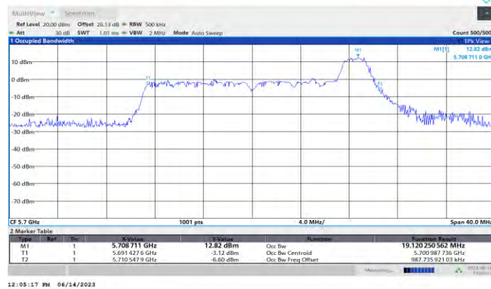
11AX20MIMO Ant1 5700 26Tone RU8
