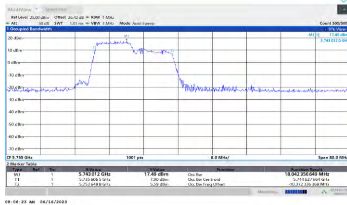
11AX40MIMO Ant0 5755 106Tone RU53
