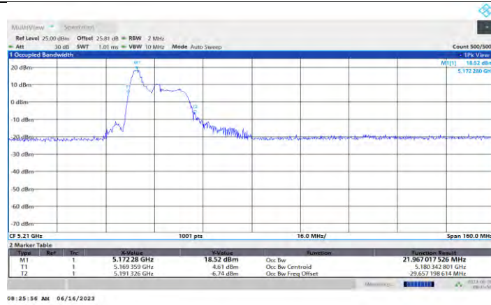
11AX80MIMO_Ant1_5210_26Tone_RU0
