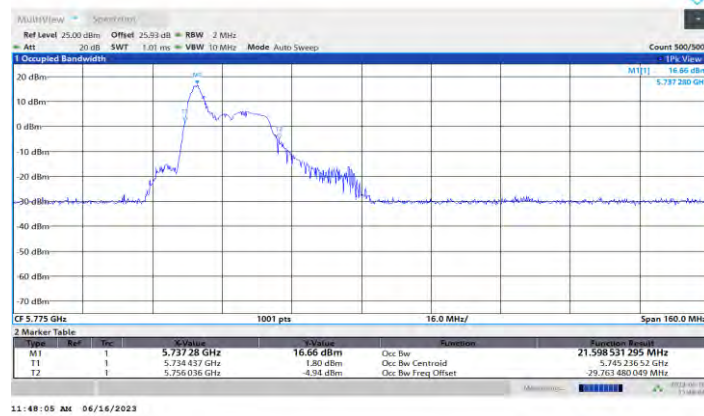
11AX80MIMO_Ant0_5775_26Tone_RU0
