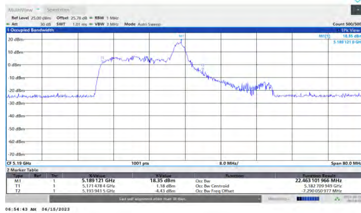
11AX40MIMO Ant1 5190 26Tone RU8
