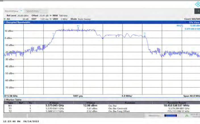
11AX20MIMO Ant1 5580 106Tone RU53
