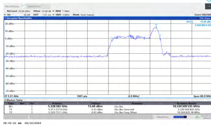
11AX40MIMO Ant0 5310 26Tone RU17
