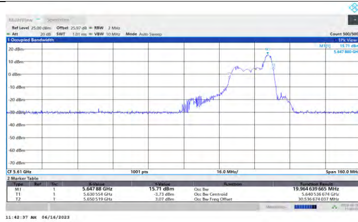
11AX80MIMO_Ant1_5610_26Tone_RU36
