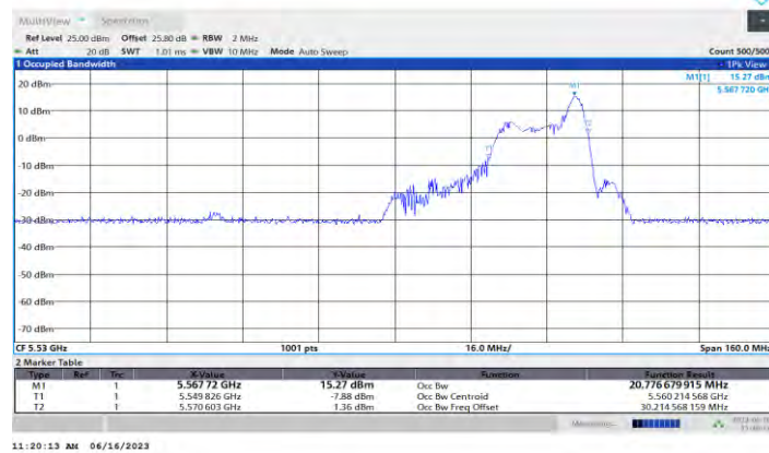
11AX80MIMO_Ant0_5530_26Tone_RU36
