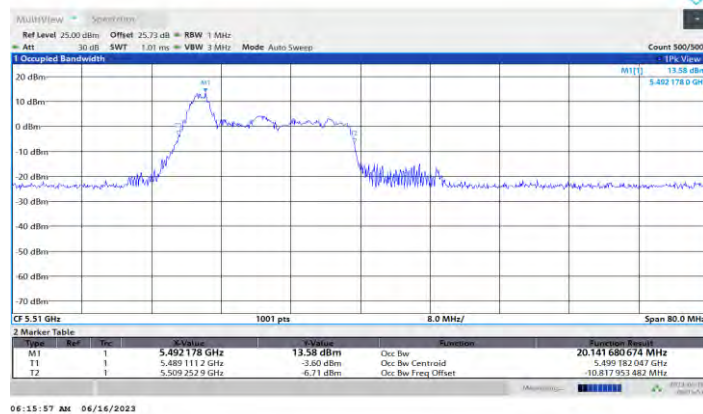
11AX40MIMO Ant0 5510 26Tone RU0
