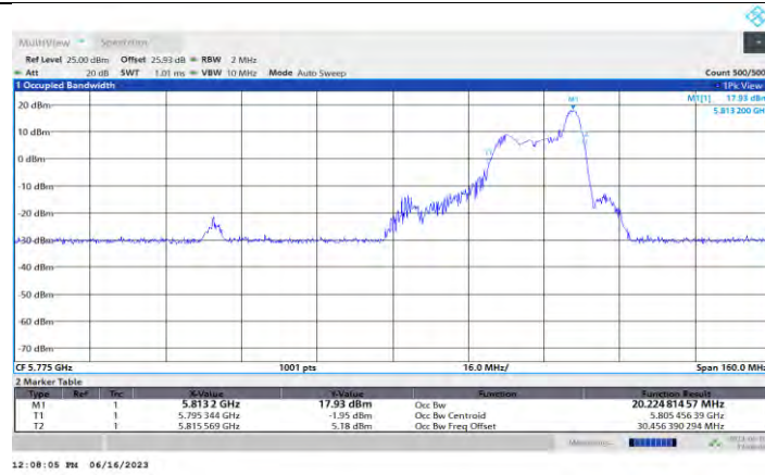
11AX80MIMO_Ant0_5775_26Tone_RU36
