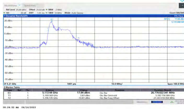
11AX80MIMO_Ant0_5210_26Tone_RU0
