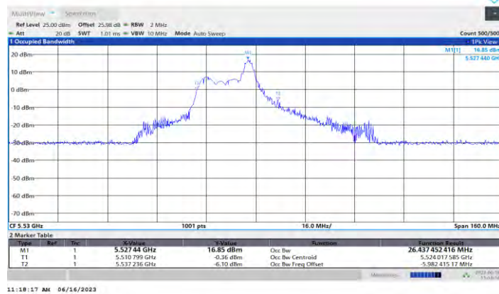
11AX80MIMO_Ant1_5530_26Tone_RU17
