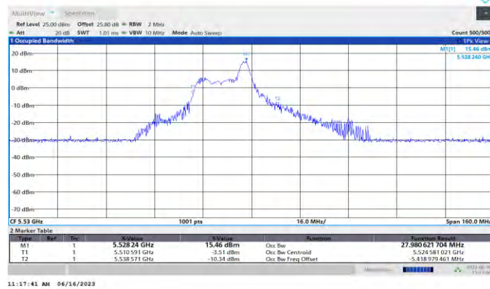
11AX80MIMO_Ant0_5530_26Tone_RU17
