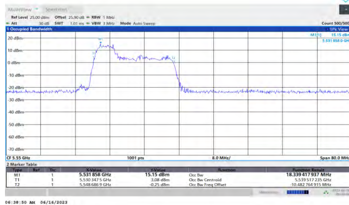
11AX40MIMO Ant0 5550 52Tone RU37
