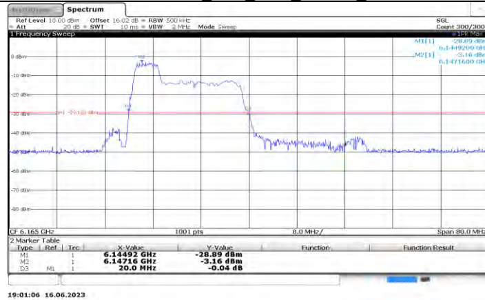
11AX40MIMO Ant0 6165 52Tone RU37
