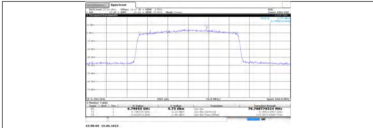
11AX80MIMO_Ant0_6785
