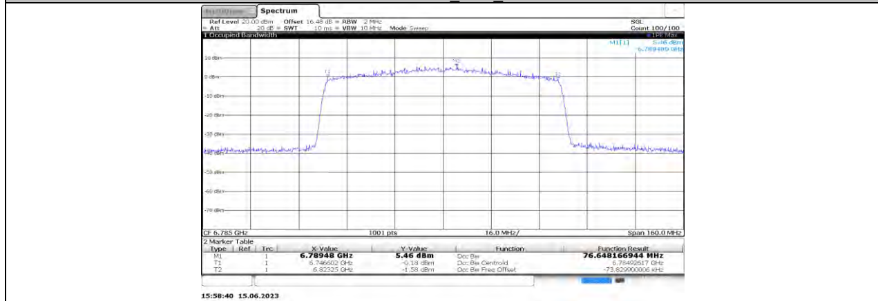
11AX80MIMO_Ant1_6785
