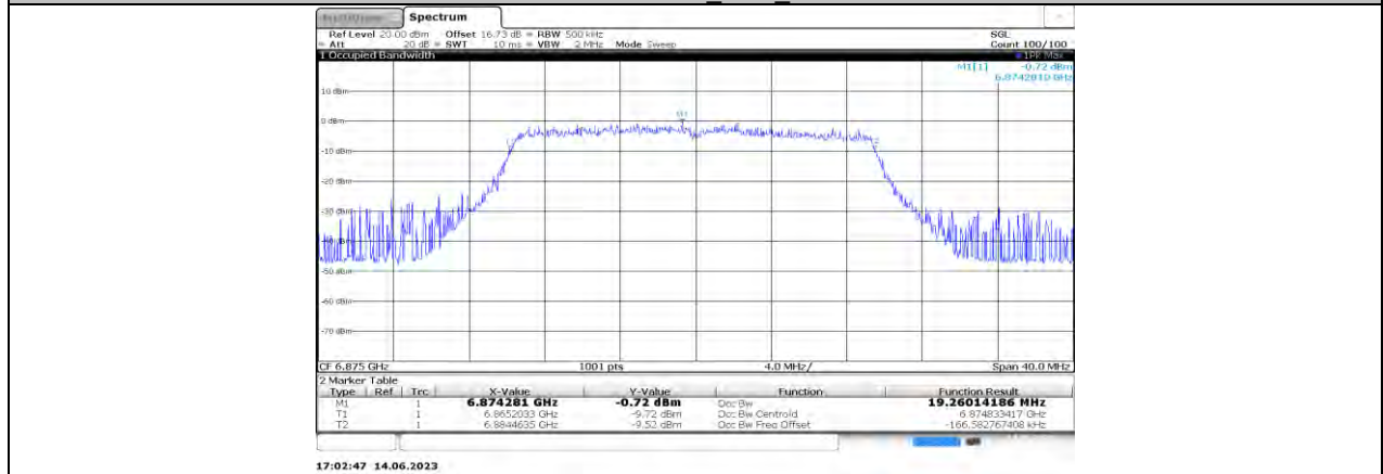
11AX20MIMO_Ant1_6875
