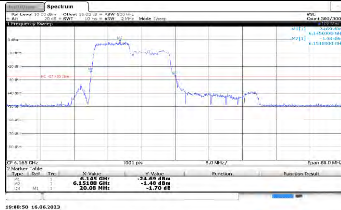
11AX40MIMO Ant0 6165 106Tone RU53
