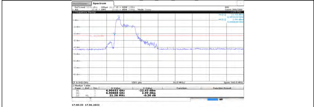
11AX80MIMO_Ant0_6945_52Tone_RU37
