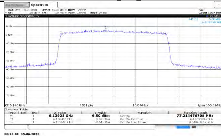
11AX80MIMO_Ant0_6145
