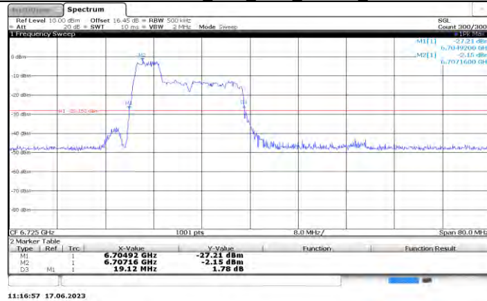
11AX40MIMO Ant0 6725 52Tone RU37
