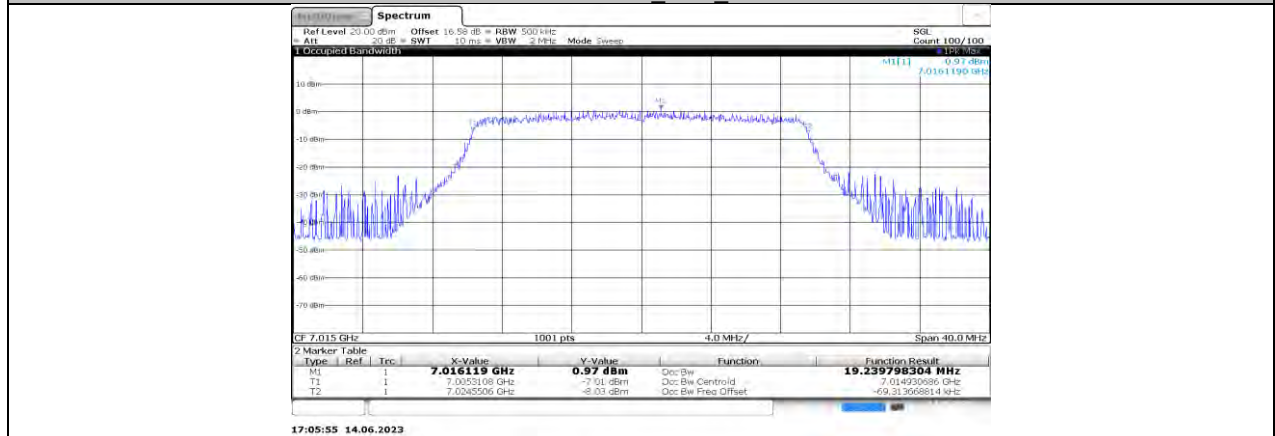
11AX20MIMO_Ant0_7015
