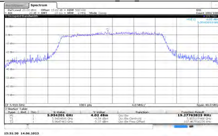
11AX20MIMO_Ant1_5955
