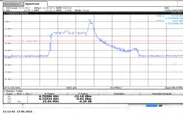
11AX40MIMO Ant0 6725 26Tone RU8
