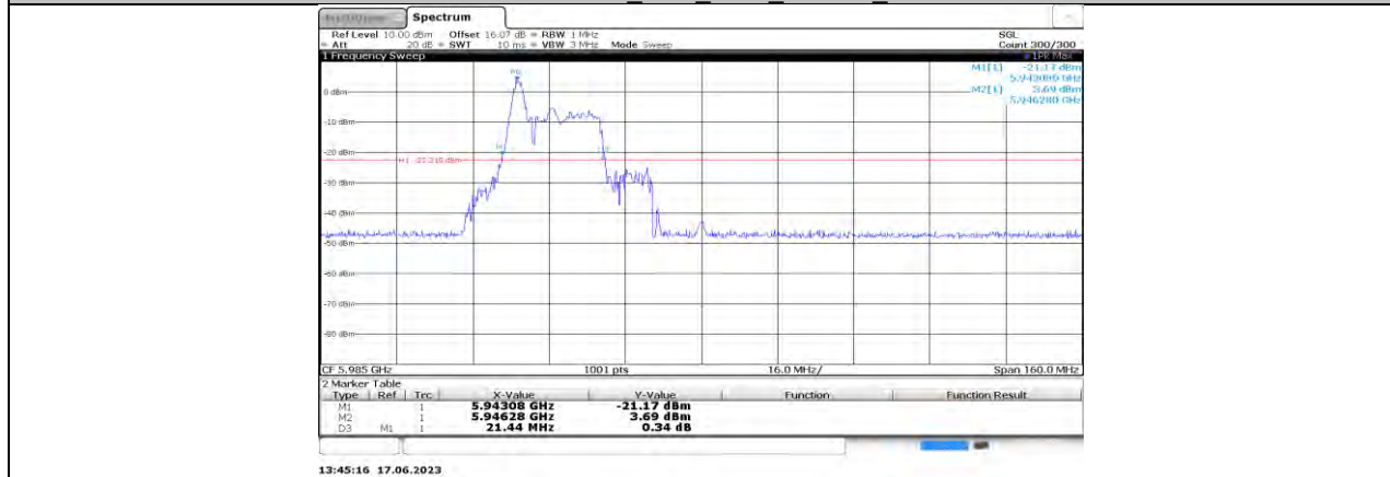
11AX80MIMO_Ant1_5985_26Tone_RU0
