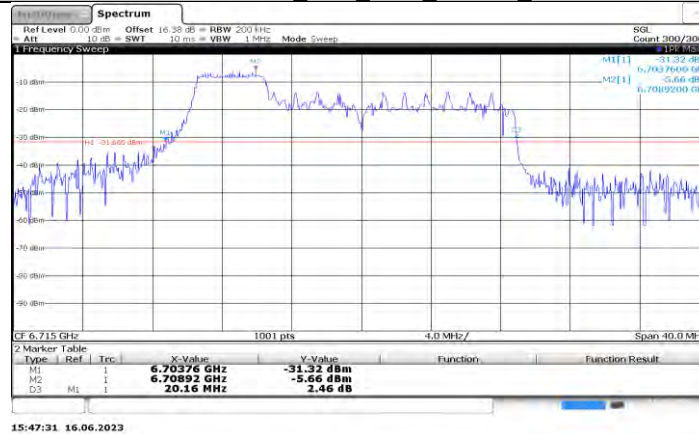
11AX20MIMO_Ant1_6715_52Tone_RU37
