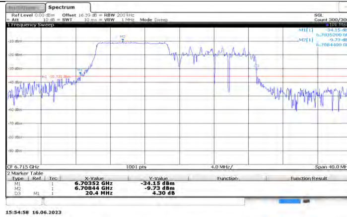
11AX20MIMO_Ant0_6715_106Tone_RU53
