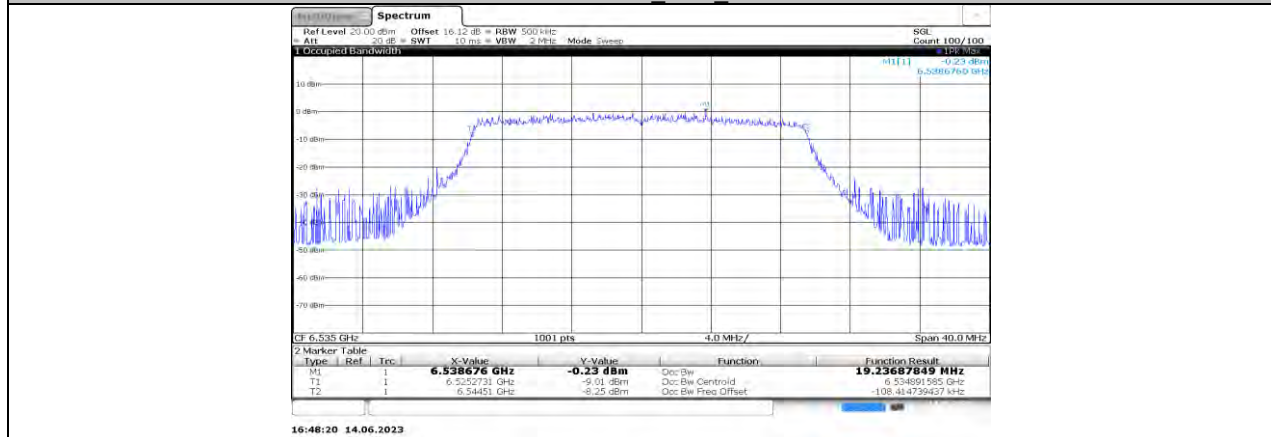
11AX20MIMO_Ant1_6535
