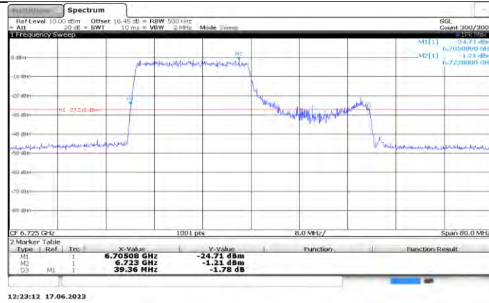
11AX40MIMO Ant0 6725 242Tone RU61
