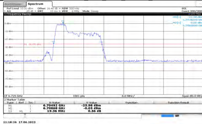
11AX40MIMO Ant1 6725 52Tone RU37
