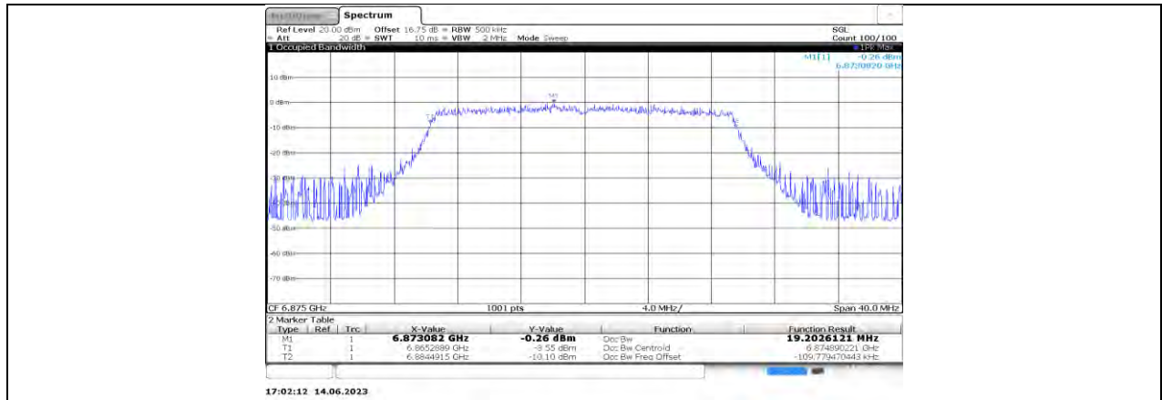
11AX20MIMO_Ant0_6875
