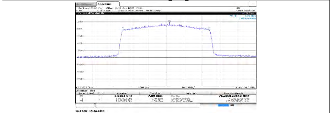
11AX80MIMO_Ant1_7025
