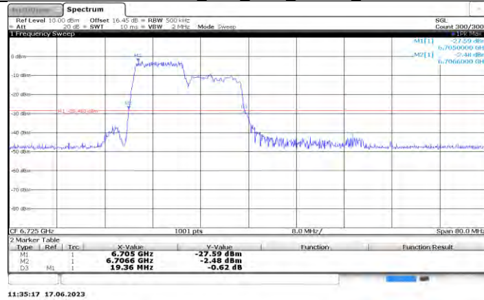
11AX40MIMO Ant0 6725 106Tone RU53
