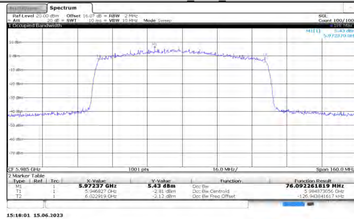
11AX80MIMO_Ant1_5985
