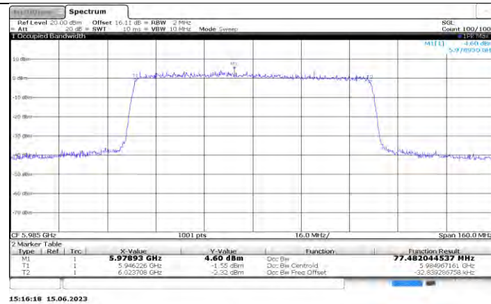
11AX80MIMO_Ant0_5985
