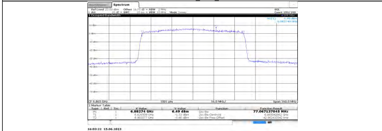
11AX80MIMO_Ant0_6865
