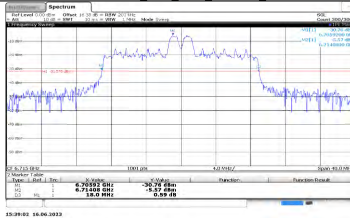
11AX20MIMO_Ant1_6715_26Tone_RU4
