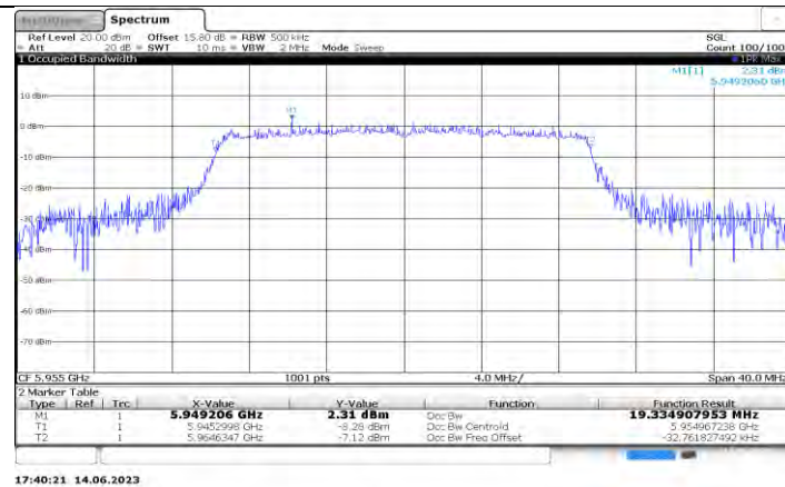
11AX20MIMO_Ant0_5955
