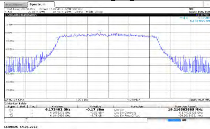
11AX20MIMO_Ant0_6175
