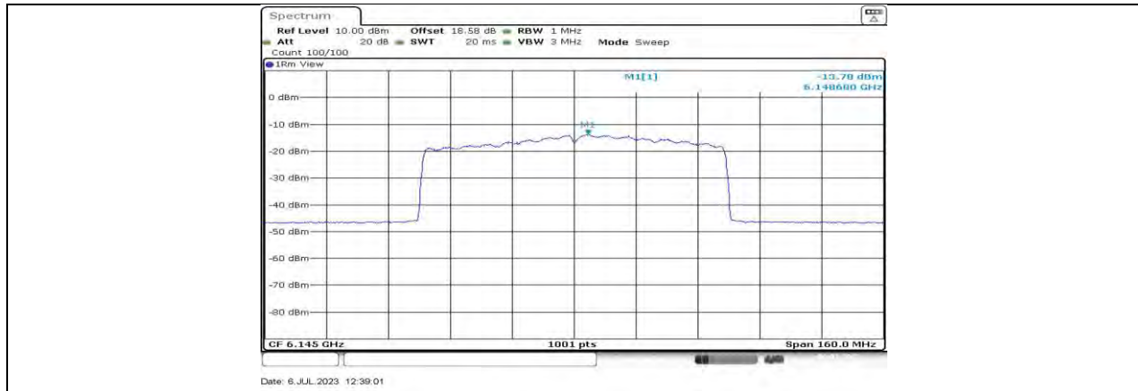
11AX80MIMO_Ant1_6145
