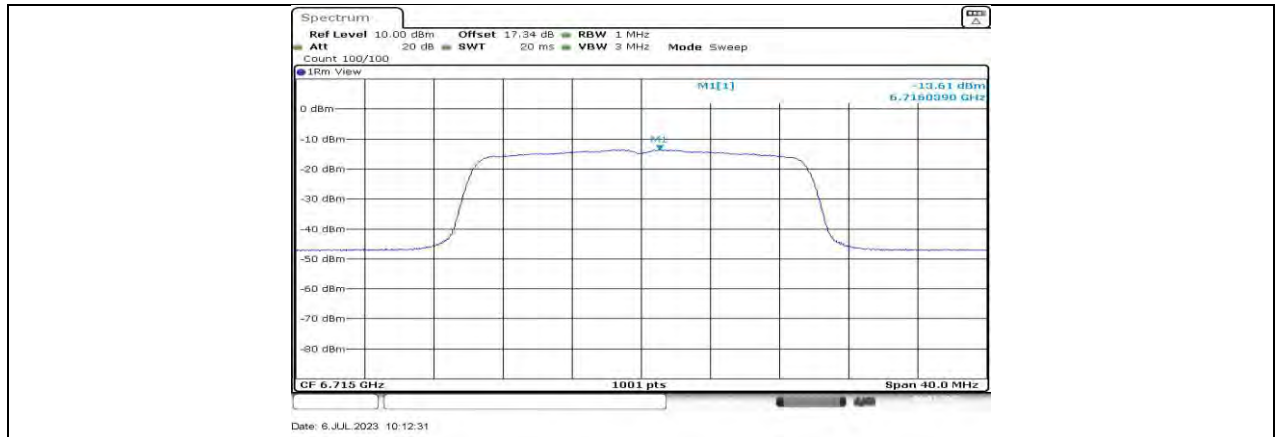
11AX20MIMO_Ant1_6715
