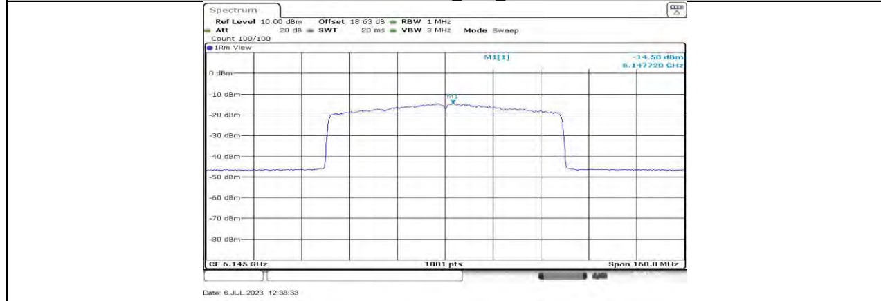
11AX80MIMO_Ant0_6145
