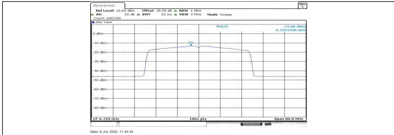
11AX40MIMO_Ant1_6725
