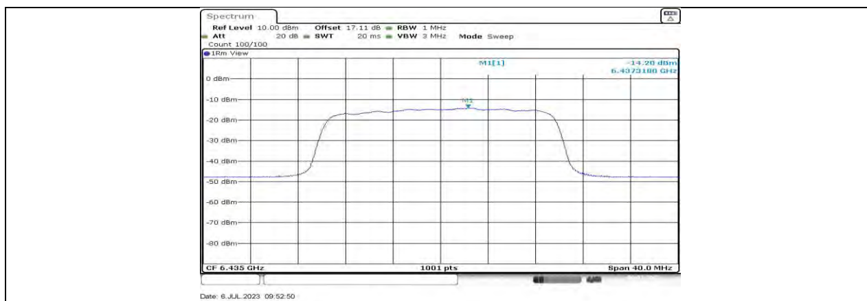
11AX20MIMO_Ant0_6435
