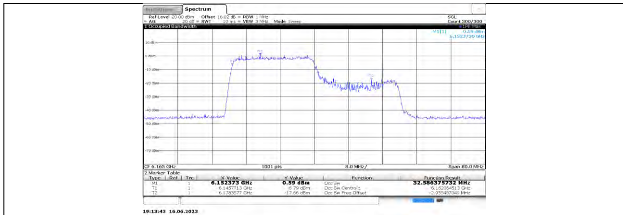
11AX40MIMO_Ant0_6165_242Tone_RU61
