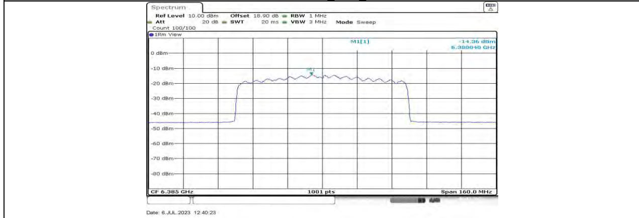
11AX80MIMO_Ant0_6385
