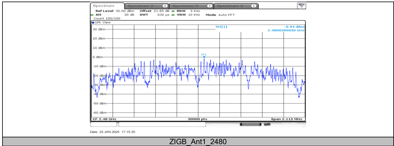
ZIGB_Ant1_2480
