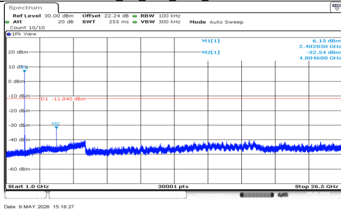
BLE_2M_Ant2_2402_1000~26500
