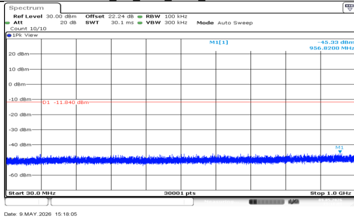
BLE_2M_Ant2_2402_30~1000
