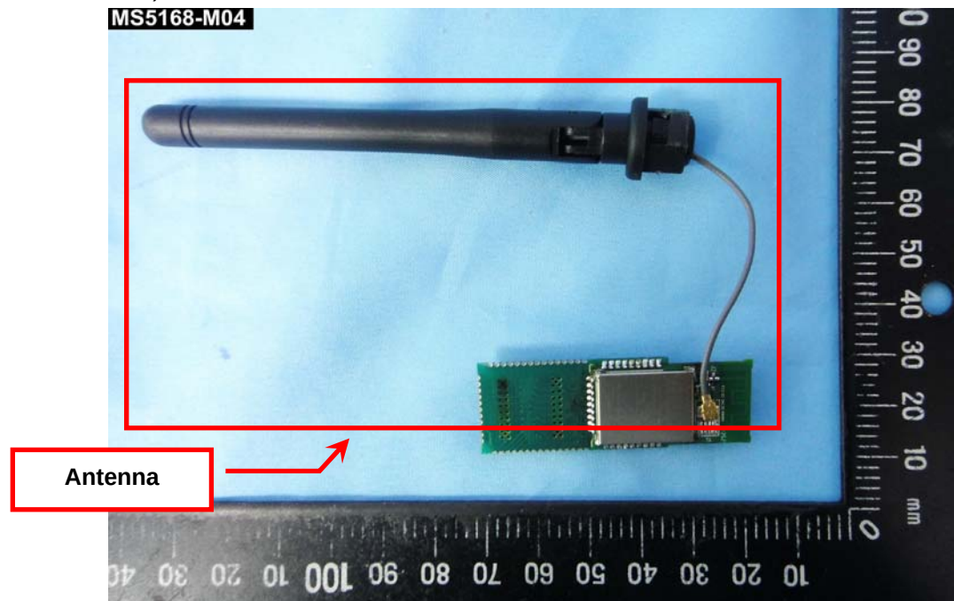
EUT Photo 1 )
